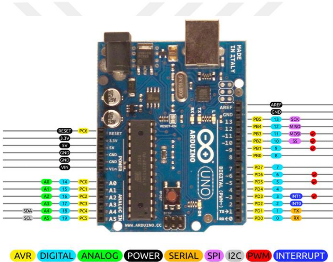
Şekil 3.3 Arduino Uno R3 Kontrol Kartı Port Bağlantıları (İnt. Kyn. 2).
