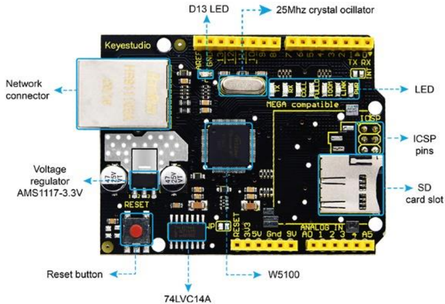
Şekil 3.4 Arduino Uno Ethernet Shield Wiznet5100 Port Bağlantıları (İnt. Kyn. 3).
