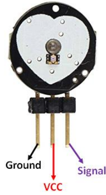
Şekil 3.9 Pulse Nabız Ölçer Algılayıcı (İnt. Kyn. 7).
