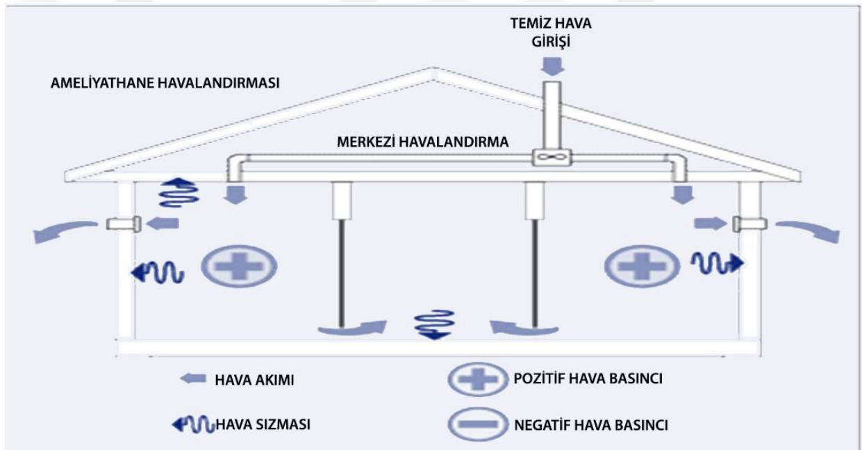
Resim 34 Ameliyathane İklimlendirmesi [25]
