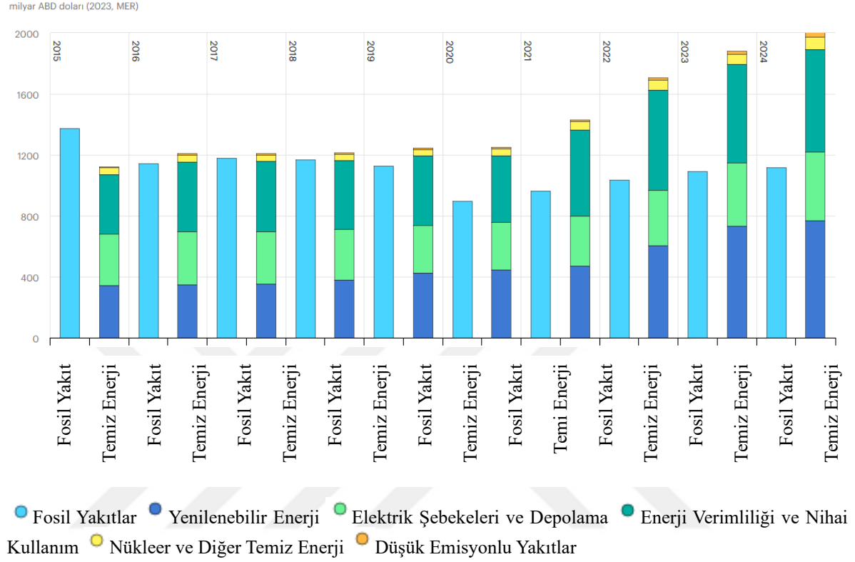
Şekil 2.4 Temiz Enerji ve Fosil Yakıtlara Küresel Yatırım, 2015-2024
