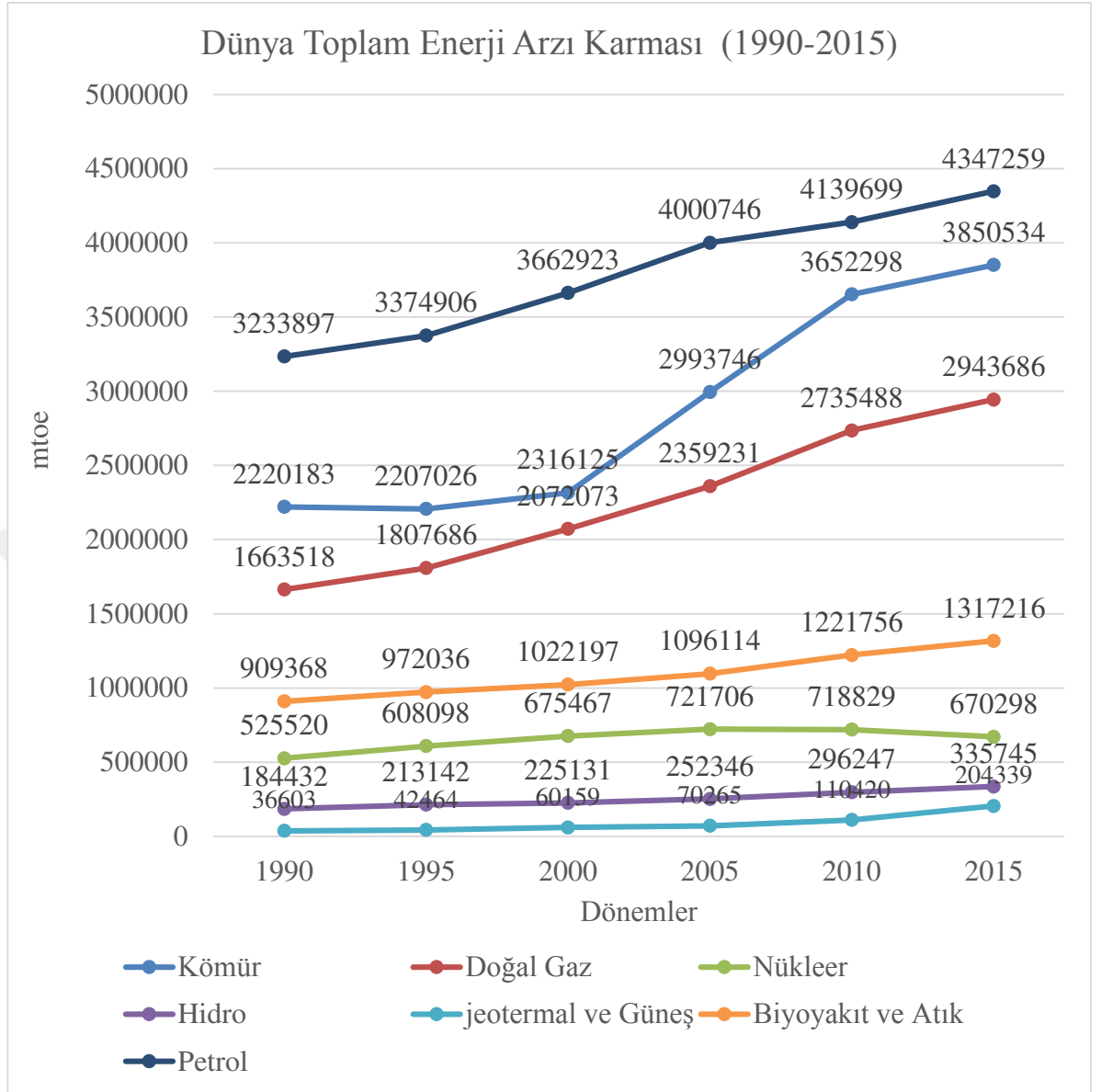
Şekil 24 Dünya Toplam Enerji Arzı Karması (1990-2015)
