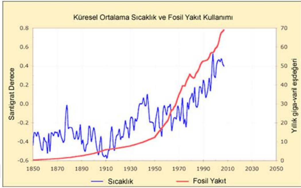
Şekil 1.10 Küresel Ortalama Sıcaklık ve Fosil Yakıt Kullanımı
