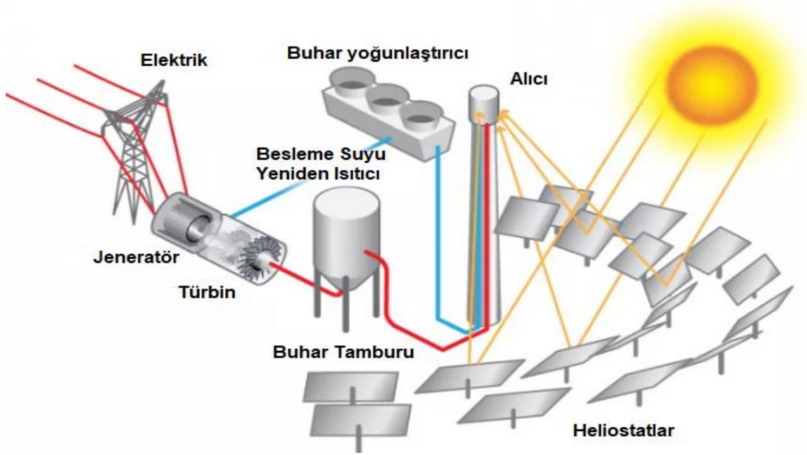
Şekil 3.2.3.b Güneş ışınları yansıtma prensibi (Office of Energy Efficiency and Renewable Energy/US Department of Energy)
