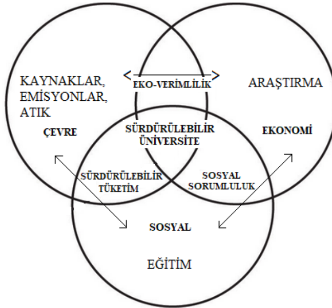
Şekil 2.1: Sürdürülebilirlik Modeli
