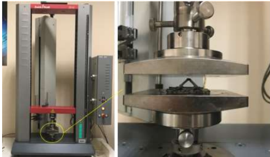
Şekil 4.2. Zwick Roell Z010 Basma testi makinesi ve teste hazır numunenin çeneler arasındaki görüntüsü
