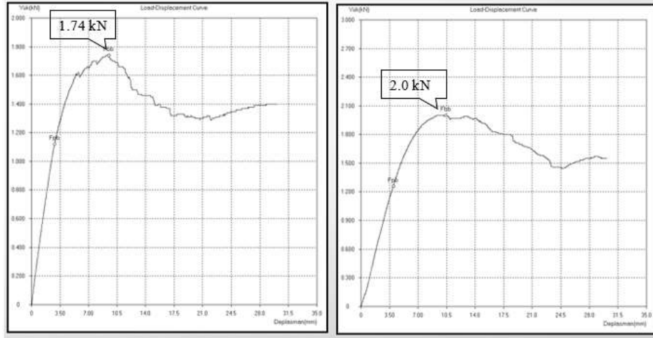
Şekil 4.10. Uç uca yapıştırılan numunelerin kuvvet deplasman grafikleri
