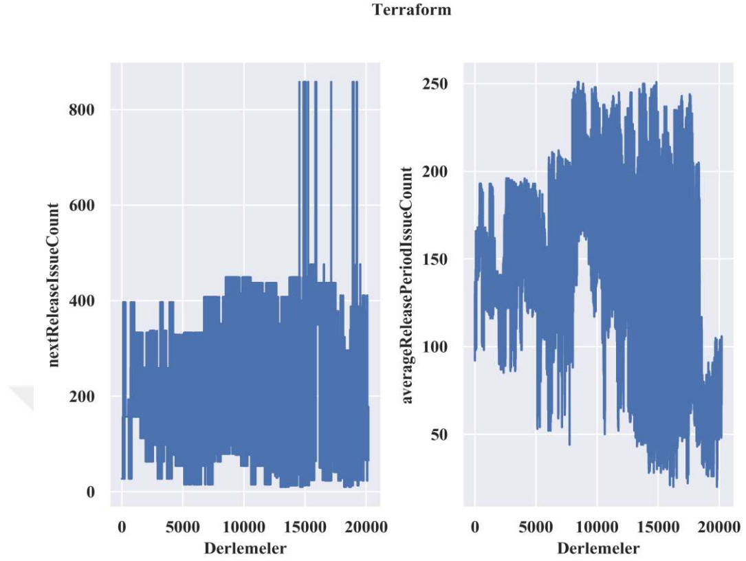
Şekil 4.3. Terraform projesi için öngörü hedeflerinin dağılımı
