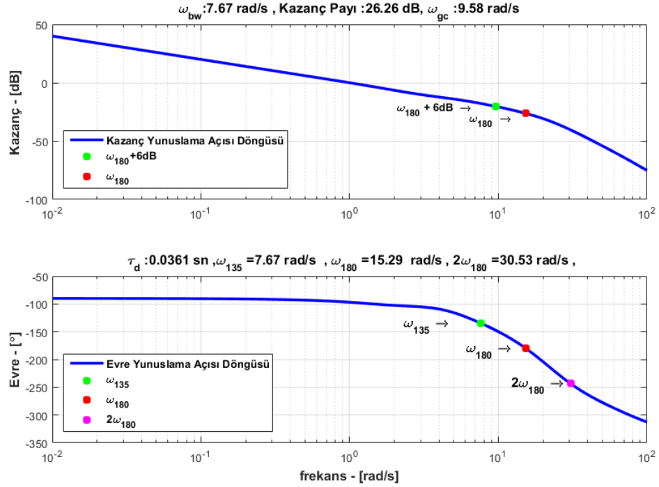
Şekil 4.31 Yunuslama açısı döngüsü bant genişliği ölçütü analizi
