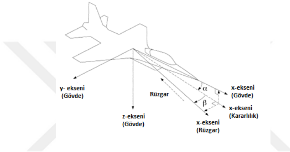
Şekil 2.7 Hava aracı üzerinde bulunan eksen takımları
