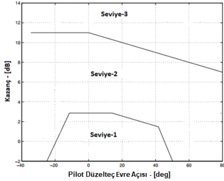
Şekil 3.9 Neal-Smith uçuş kalitesi grafiği
