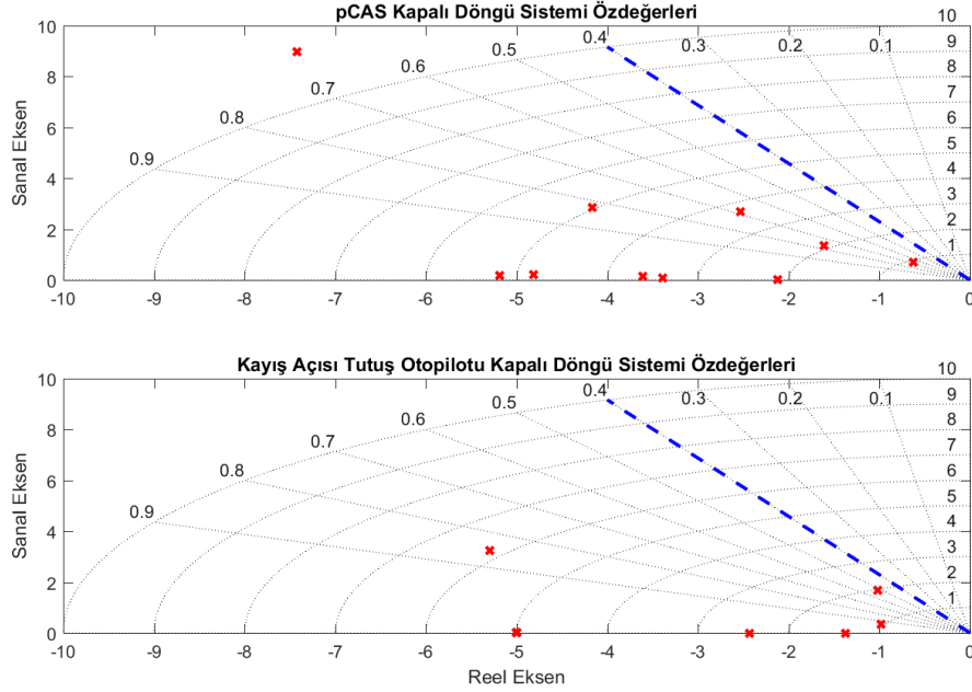
Şekil 4.15 Kapalı döngü sistem özdeğerleri
