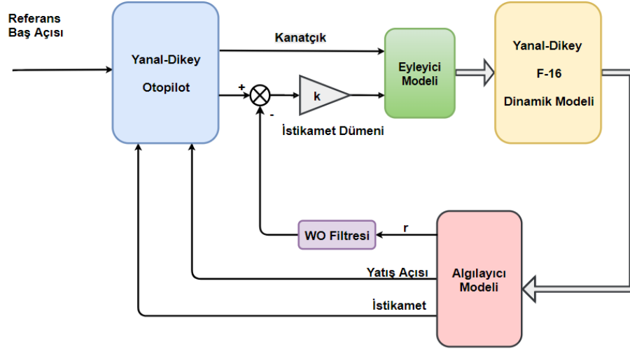
Şekil 3.3 Yanal-dikey bütünleşik otopilot mimarisi
