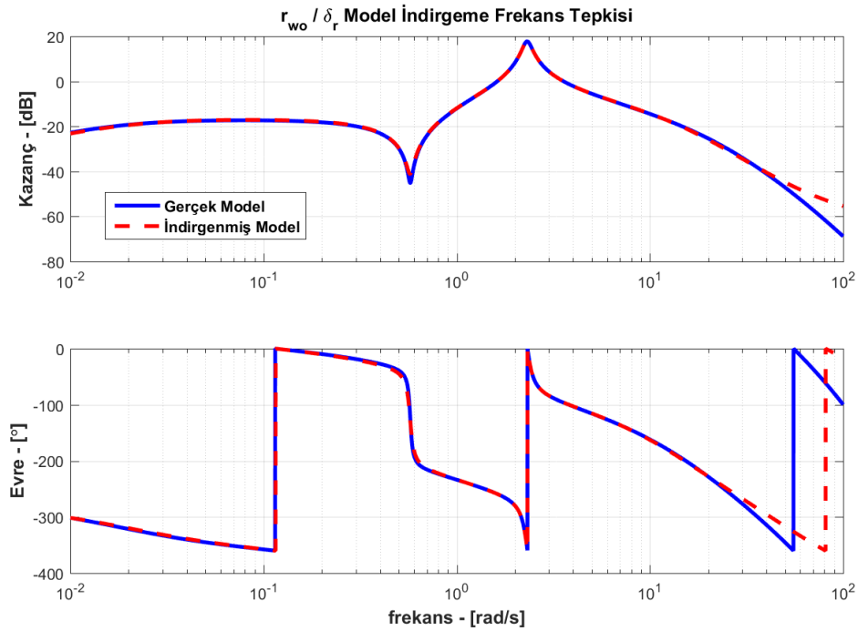
Şekil 4.5 r_{wo} döngüsü modelinin indirgenmiş model ile frekans tepkisinin karşılaştırması
