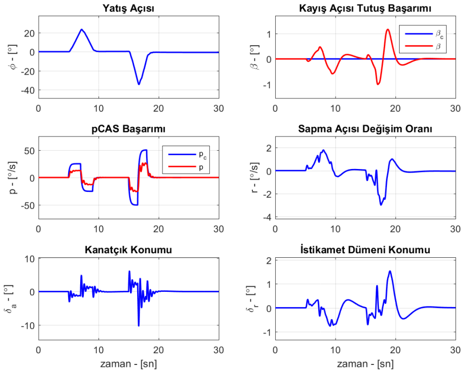
Şekil 5.4 p kazancı arttırılmış pCAS testi sonucu
