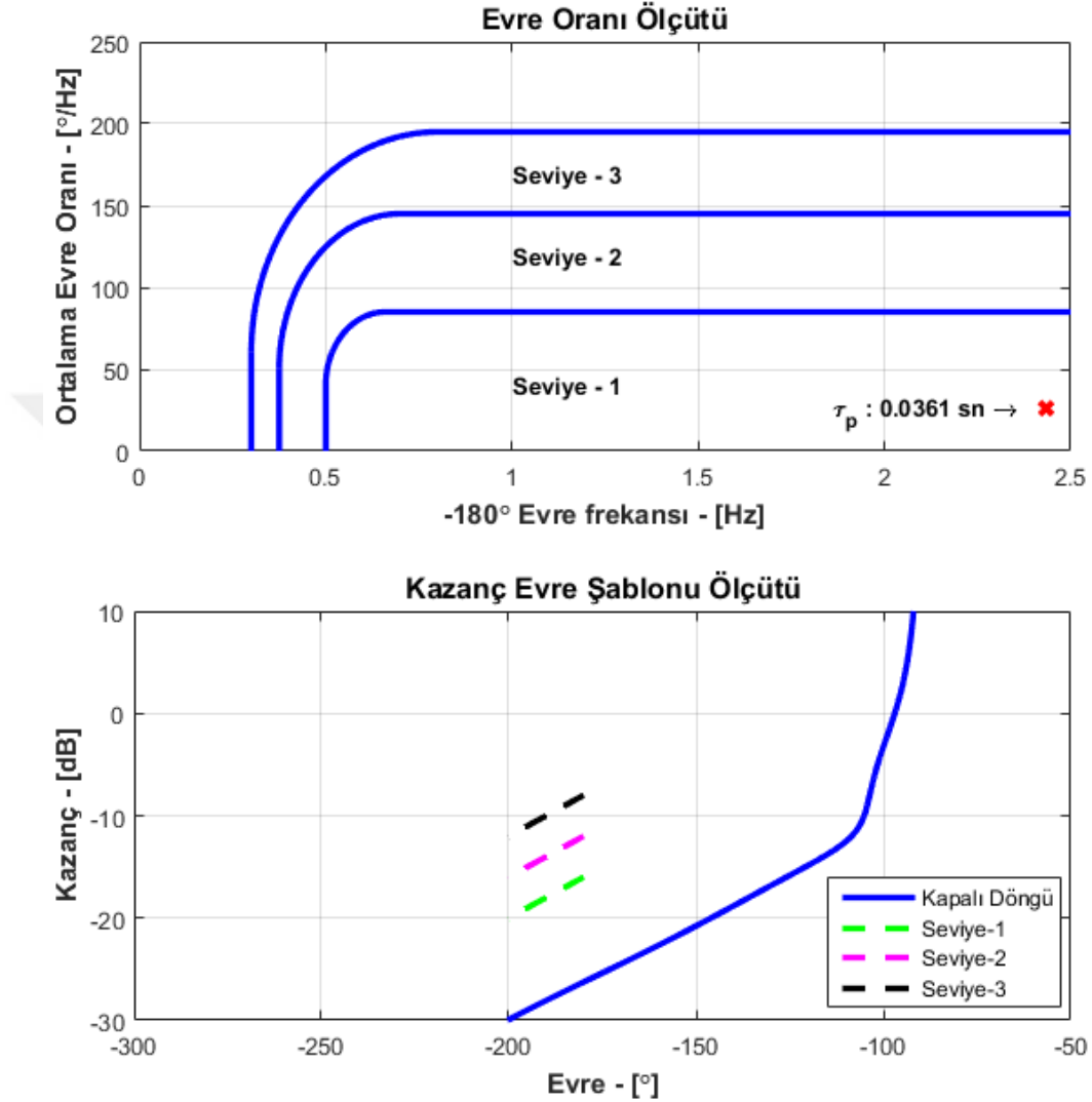
Şekil 4.33 Kullanım kalitesi evre oranı ile kazanç evre şablonu ölçütü analizi
