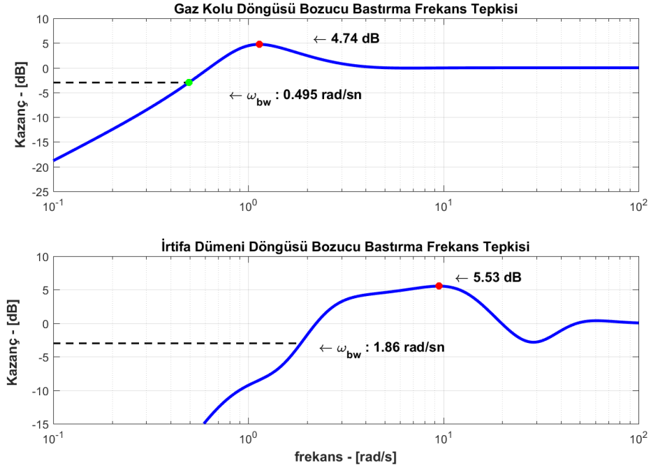
Şekil 4.58 Gaz kolu ve irtifa dümeni döngüleri bozucu bastırma analizi
