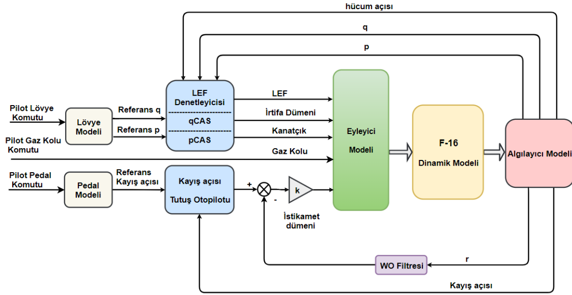
Şekil 3.1 Pilot destekleyici uçuş denetim sistemi mimarisi
