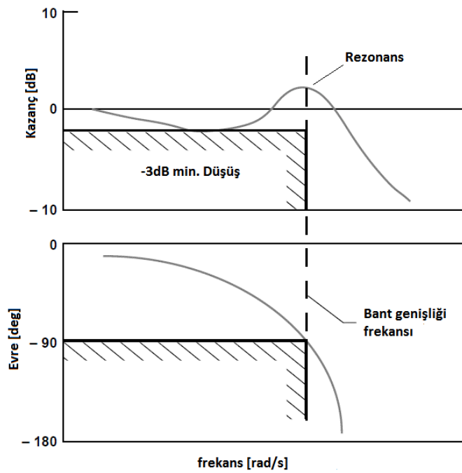
Şekil 3.10 Neal-Smith ölçütü yöntemi
