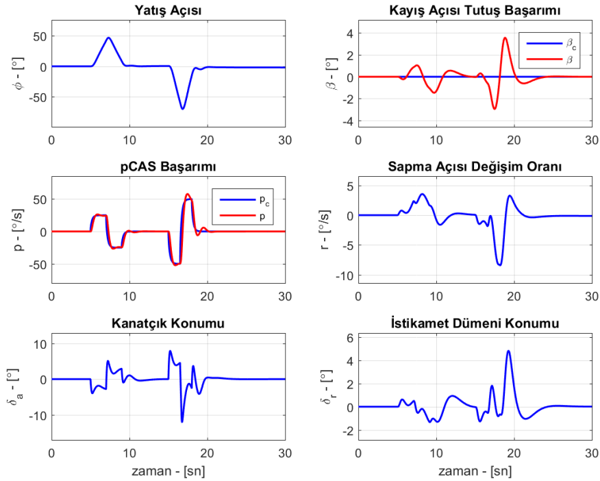
Şekil 5.6 Model hatası eklenmiş pCAS testi sonucu
