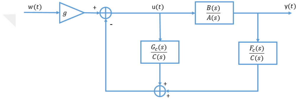
Şekil 4.1 SÜGÖNDE yöntemi şeması
