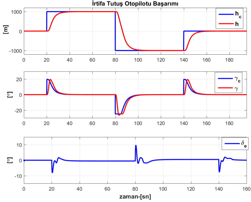
Şekil 4.52 İrtifa tutuş otopilotu basamak girişi tepkisi başarımı
