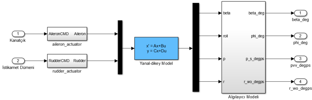
Şekil 4.4 F-16 yanal-dikey eksen genişletilmiş modeli
