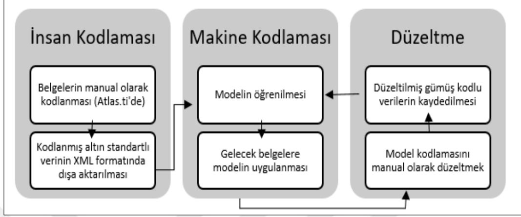
Şekil 4: Yan, McCracken ve Crowston'un yarı-otomatik içerik analizi şeması
