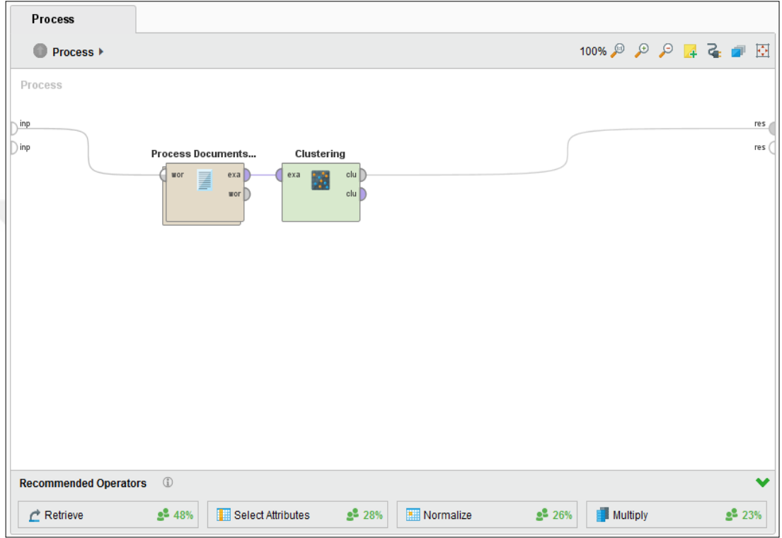
Şekil 5: Kümeleme algoritması
