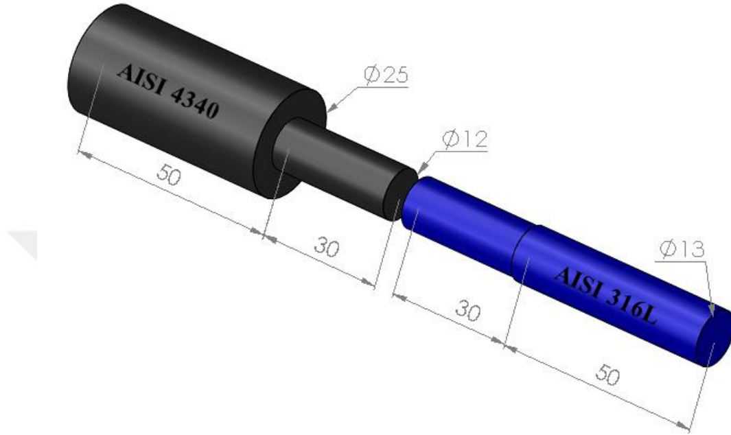
Şekil 4. 1. Kaynak yapılan numunelerin katı modellenmiş görüntüsü.
