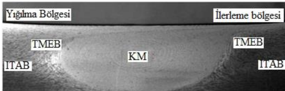
Şekil 3. 6. SKK işlemi sonrası oluşan mikroyapılar (Srubar, 2009).
