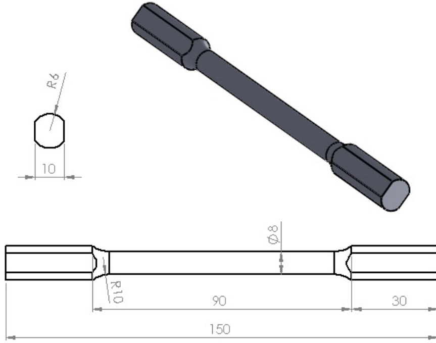
Şekil 4. 13. Burulma numunesi ölçüleri.
