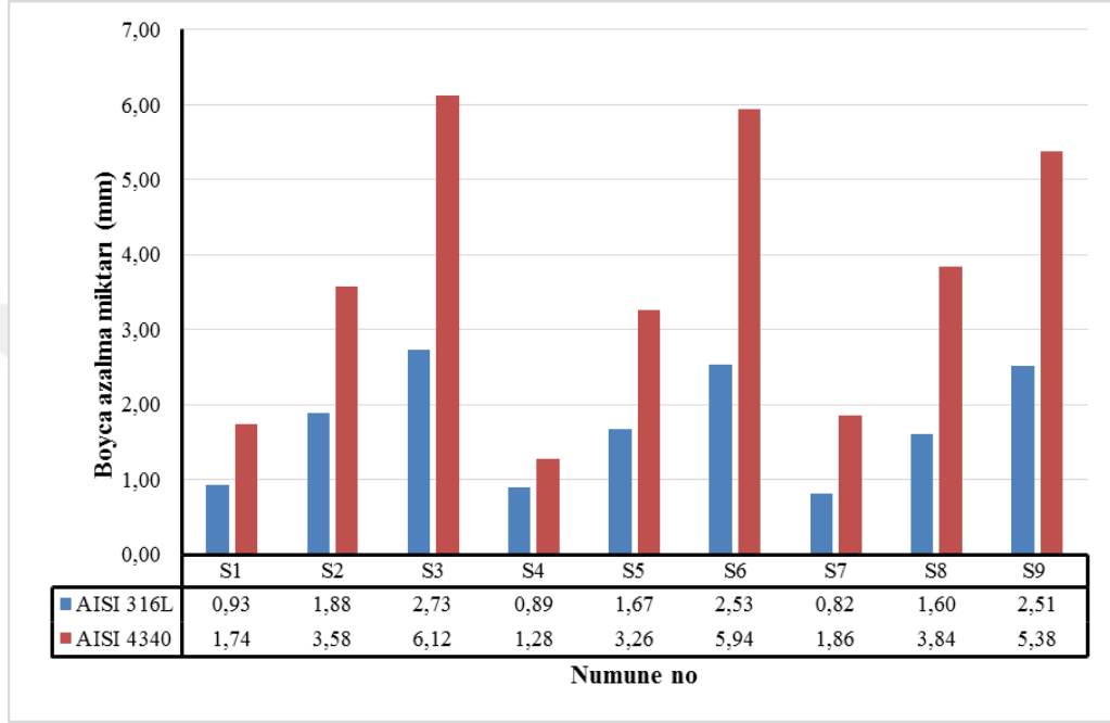
Şekil 5. 2. AISI 316L ve AISI 4340 numunelerin boyca azalma miktarları.
