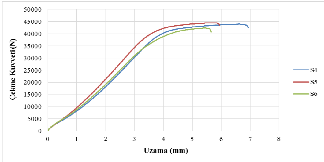
Şekil 5. 15. 2200 dev/dak'da kaynak edilen AISI316L/AISI4340 çeliklerin çekme deney sonuçları
