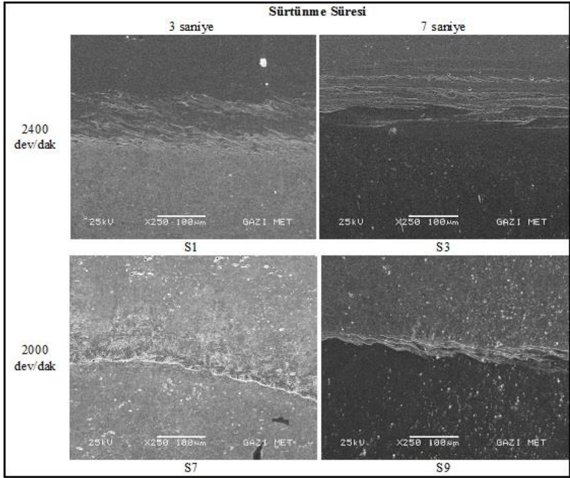
Şekil 5. 7. Farklı dönme devri ve sürtünme süresi parametreleri kullanılarak kaynak edilen malzemelerin arayüzeylerinin SEM fotoğrafları.
