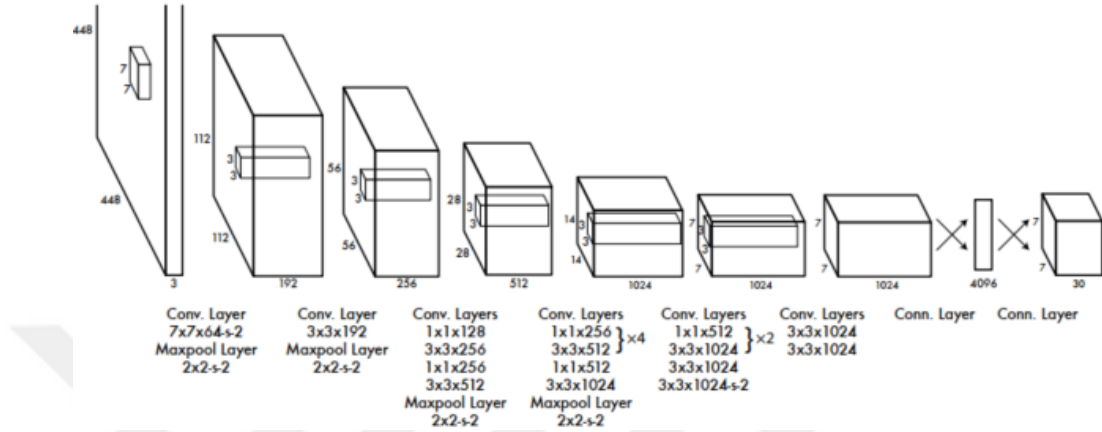
Şekil 2.18. Nesne tespitinden sorumlu YOLO katmanlı mimarisi [68]
