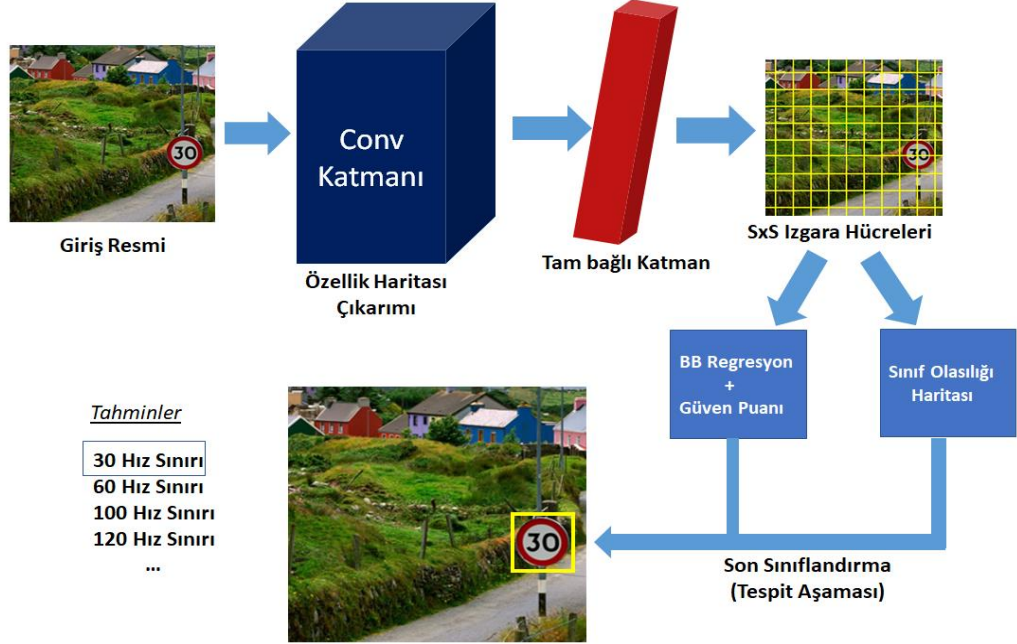
Şekil 2.16. YOLO'nun nesne tespitiye yönelik çalışma prensibi
