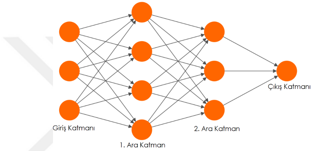
Şekil 2.2. Çok katmanlı bir YSA yapısı
