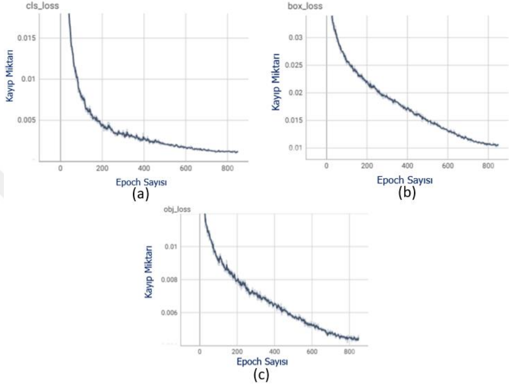
Şekil 3.23. Modelin eğitim sonucu performansı (a) Sınıflandırma doğruluğunun kayıp grafiği (b) Sınırlandırıcı kutunun doğruluğu için oluşan kutu kaybı (c) Oluşan nesnellik kayıp grafiği
