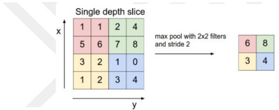
Şekil 2.6. Havuzlama işlemlerinden max-havuzlama işleminin yapılması [49]
