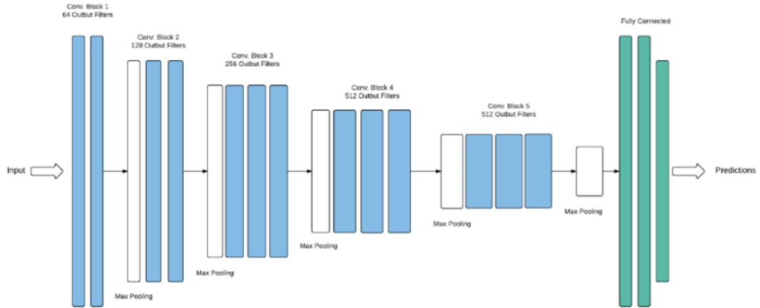
Şekil 2.10. VGGNet mimarisi genel yapısı
