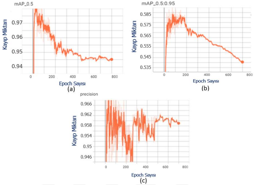
Şekil 3.33. Modelin eğitim performansına ilişkin oluşan (a) IoU değeri 0,5 için oluşan ortalama kesinlik (b)IoU değeri 0,5 ile 0,95 arasındaki adımlarda oluşan ortalama kesinlik (c) Kesinlik grafikleri
