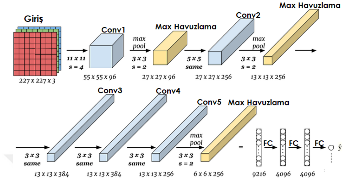
Şekil 2.8. Alexnet mimarisi sınıflandırma adımları [57]
