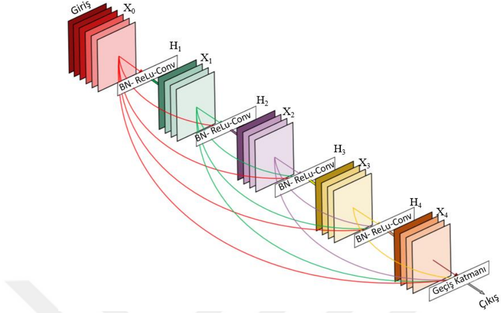
Şekil 2.21. Büyüme hızı k=4 olan 5 katmanlı bir DenseNet bloğu [77].
