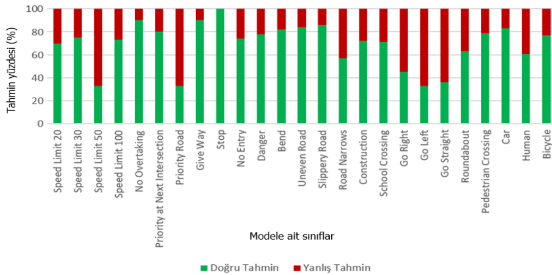
Şekil 3.25. Modelin test sonucuna ilişkin tahmin doğruluğu grafiği
