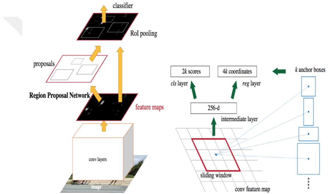
Şekil 2.14. Faster R-CNN modelinin çalışma prensibi [66]
