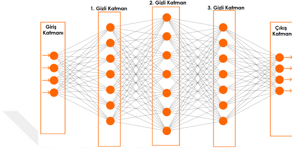
Şekil 2.3. İki den fazla gizli katmana sahip DNN yapısı
