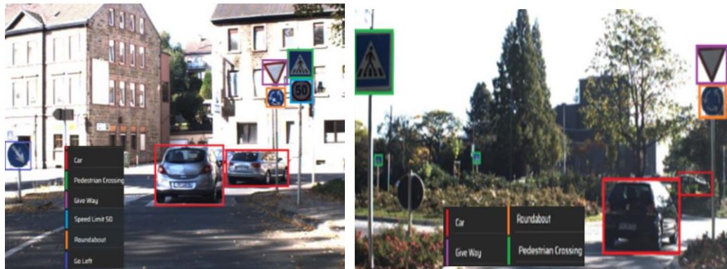
Şekil 3.11. Araç dışı ADAS uygulaması için insan, araç ve trafik işaretlerinin etiketlenmesi
