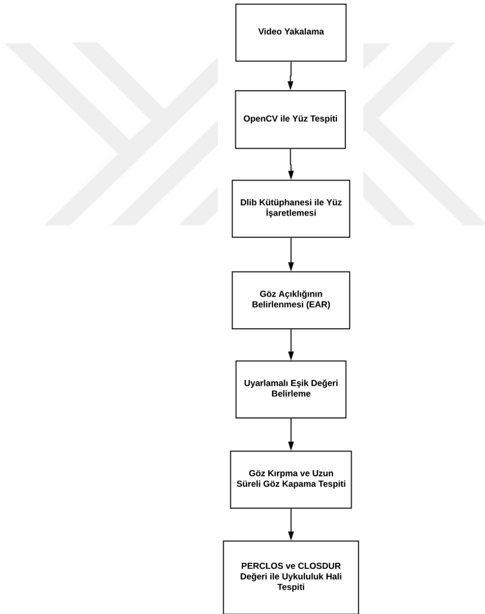
Şekil 3.2. Önerilen Sistemin Blok Şeması
