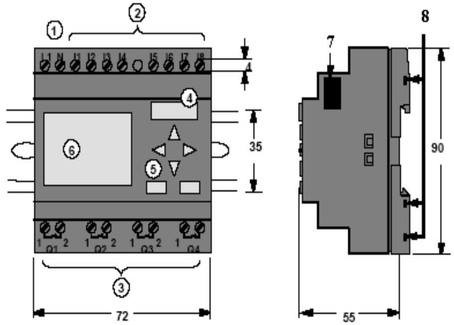
1.Güç girişi, 2. Girişler, 3.Çıkışlar, 4.Modül yuvası, 5.Kumanda paneli, 6.LCD, 7.Genişletme arayüzü, 8.Mekanik kodlama soketi
