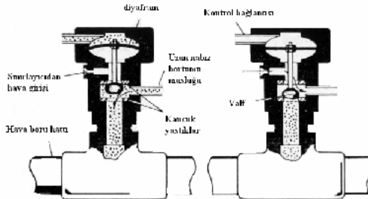
Şekil 1.10 Vaccar pnömatik ara nabız aygıtı (Nalbant, 1987)
