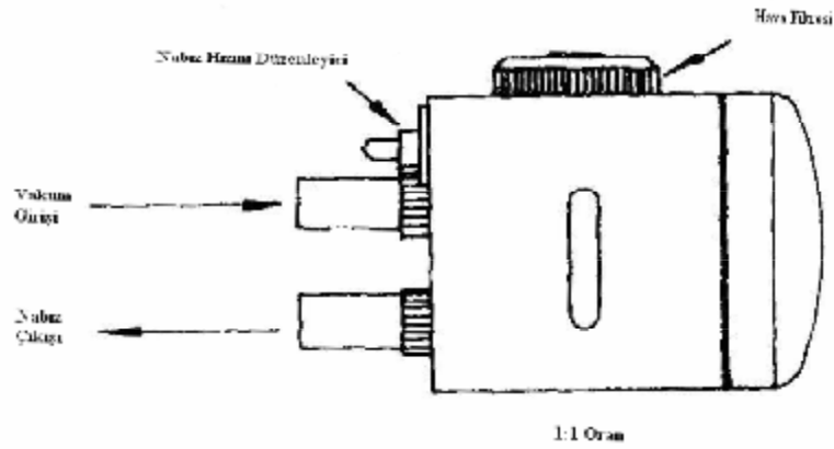
Şekil 1.5 Alfa Laval standart bağımsız nabız aygıtı (Nalbant, 1987)
