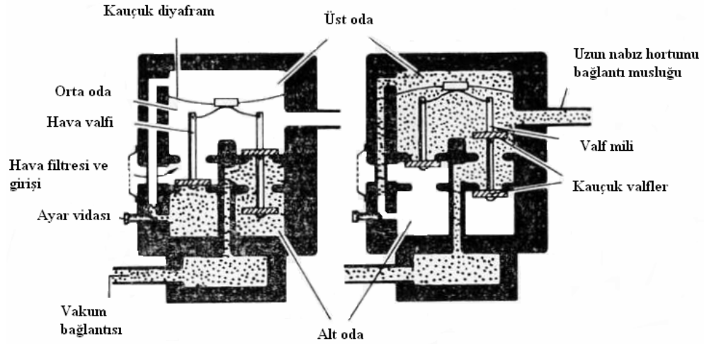
Şekil 1.9 Christensen pnömatik bağımsız nabız aygıtı (Nalbant, 1987)
