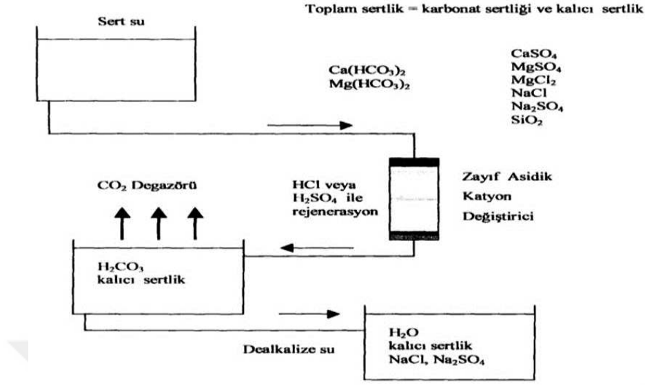
Şekil 3.6. Dealkalizasyon çalışma sistemi (URL-6, 2016)
