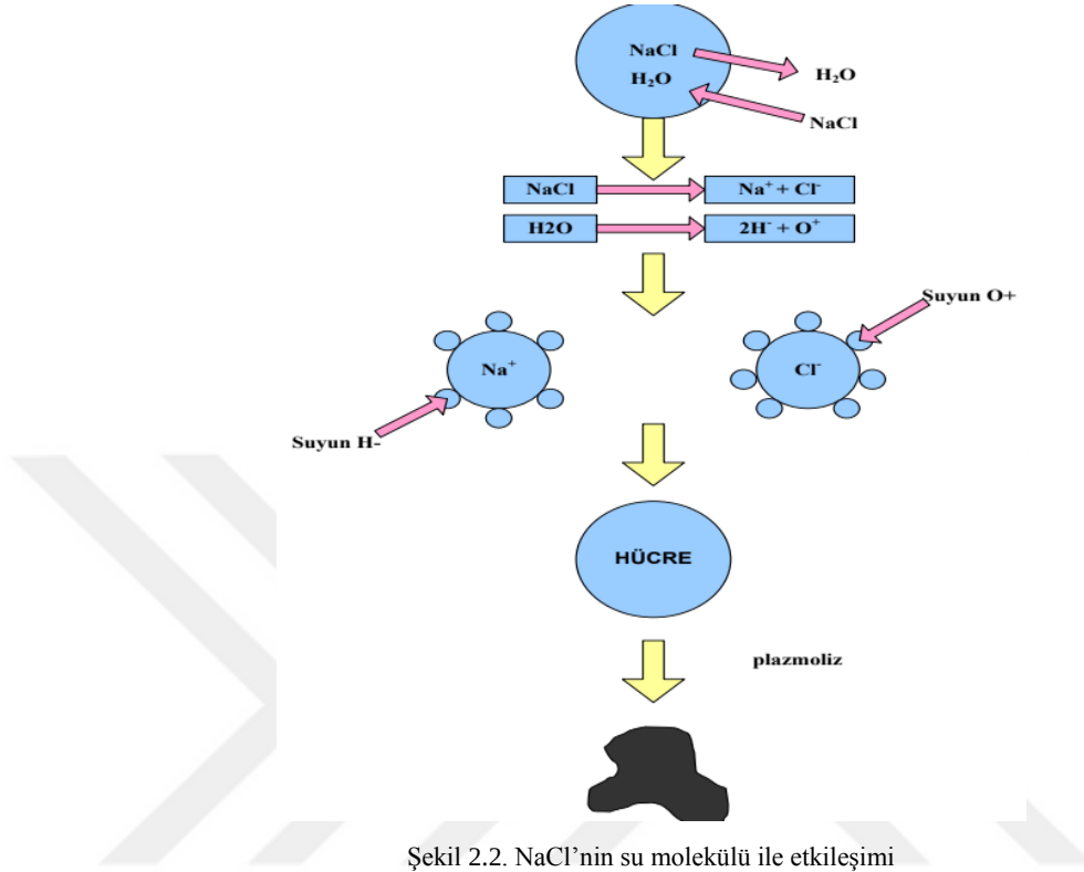
Şekil 2.2. NaCl'nin su molekülü ile etkileşimi
