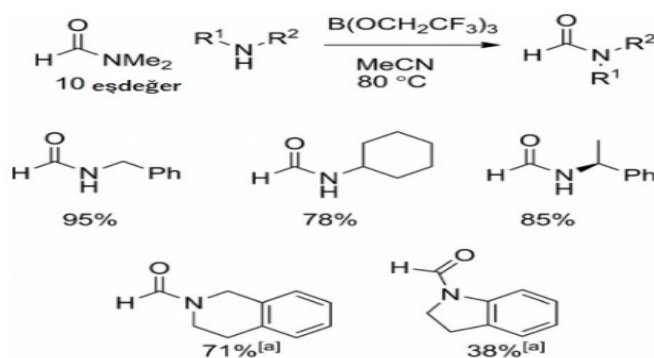
Şekil 2. 22. DMF'nin transamidasyonu yoluyla formamidlerin B(OCH_2CF_3)_3 aracılı sentezi. [a] Reaksiyon 100 °C'de gerçekleştirildi.
