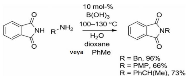
Şekil 2. 23. B(OH) 3 tarafından katalize edilen ftalimidin transamidasyonu.
