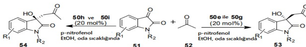
Şekil 2. 63. Katalizör olarak \beta -amino amidlerin kullanıldığı Aldol reaksiyonu.
