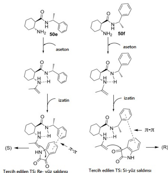
Şekil 2. 63. Katalizör olarak \beta -amino amidlerin kullanıldığı Aldol reaksiyonu.
