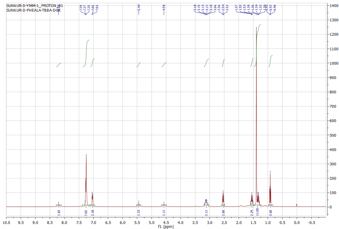
Şekil 4. 10. (1b) maddesine ait ^1\text{H} NMR analizi.
