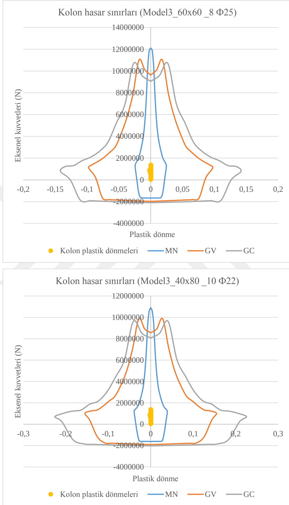
Şekil 3.111. Model3_ref'nin kare (üst) ve dikdörtgen (kare) kolonlarındaki hasarların belirlenmesi
