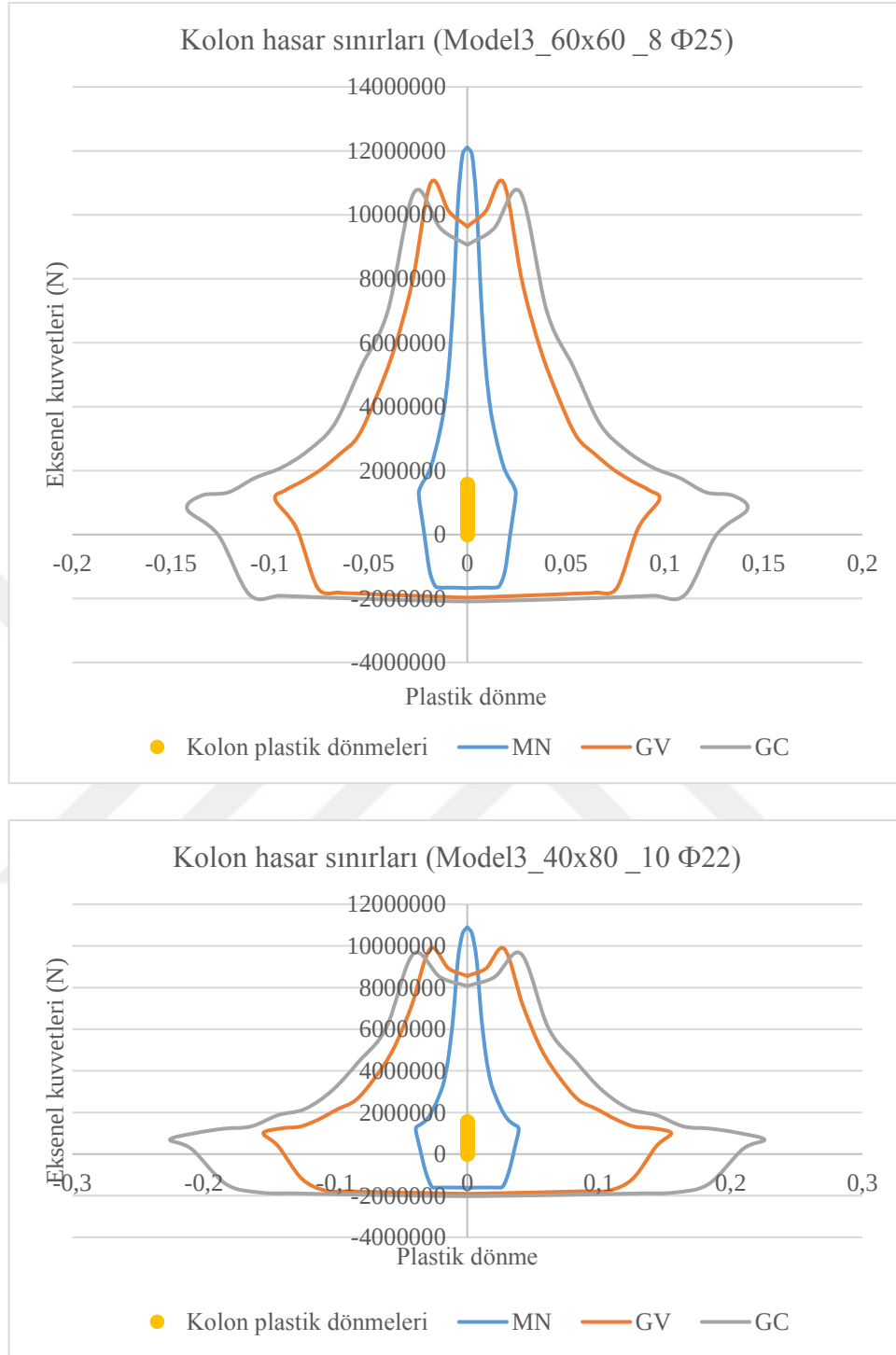
Şekil 3.120. Model3_ref 'nin kare (üst) ve dikdörtgen (alt) kolonlarındaki hasarların belirlenmesi
