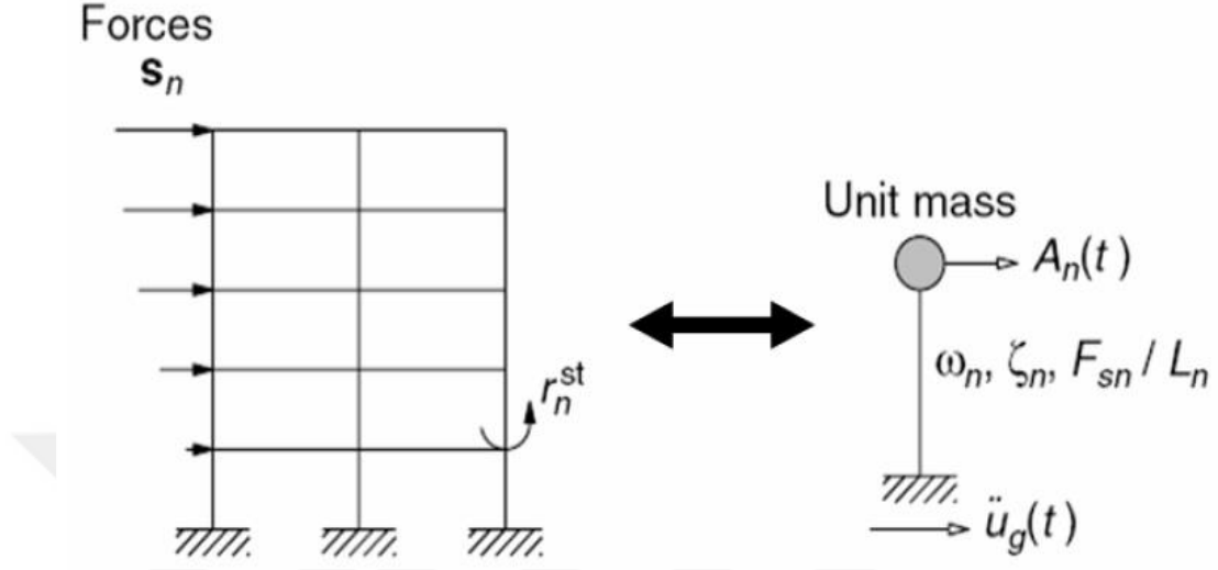
Şekil 2.10. Elastik olmayan ÇSD sistemlerinin MPA'larının kavramsal açıklaması [21]
