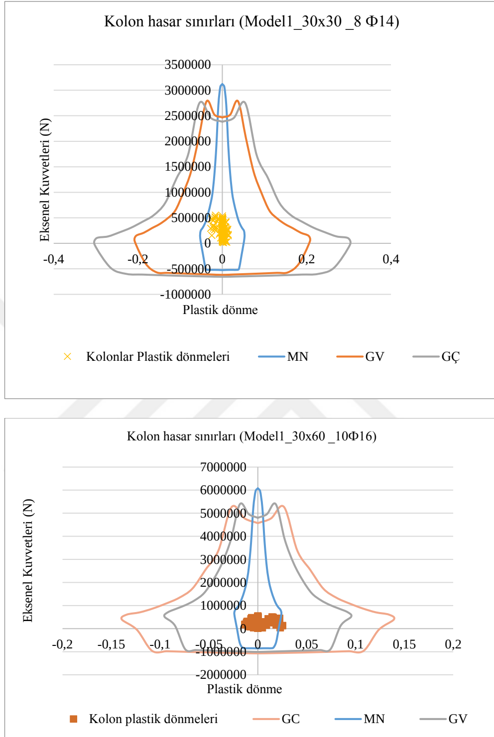
Şekil 3.39. Model1_ref'nin kare (üst) ve dikdörtgen (alt) kolonlarındaki hasarların belirlenmesi
