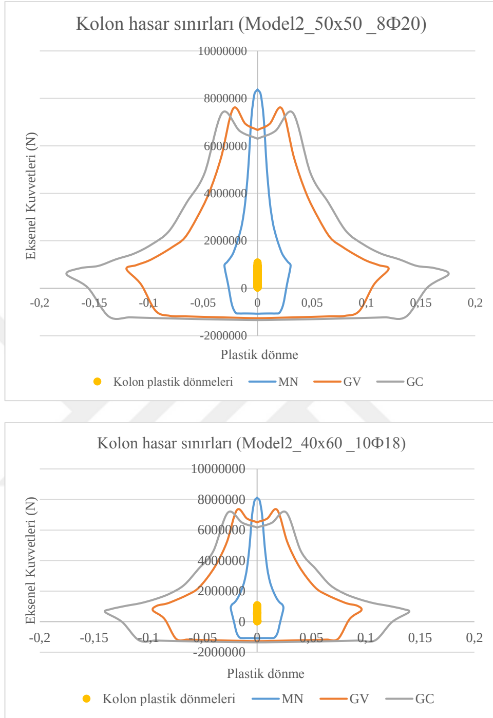
Şekil 3.96. Model2_T2'nin kare (üst) ve dikdörtgen (alt) kolonlarındaki hasarların belirlenmesi
