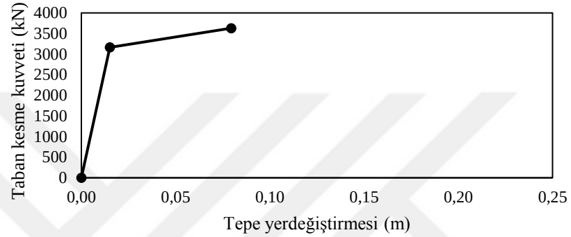
Şekil 3.41. Pozitif (üst) ve negatif (alt) Y yönleri doğrusal eğriler
