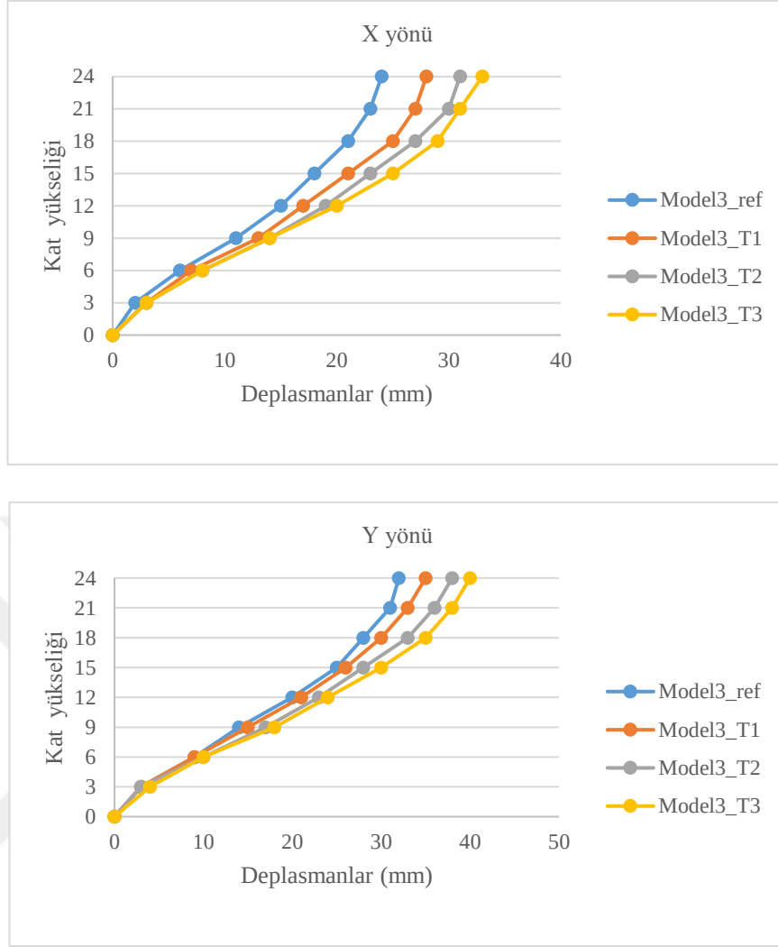
Şekil 4.21. X ve Y yönünde Model3 kat deplasmanlarının karşılaştırılması
