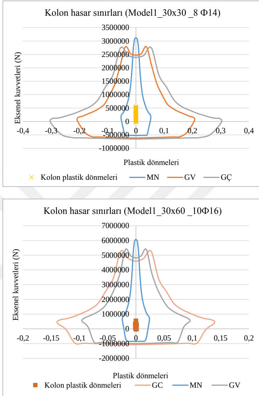
Şekil 3.48. Model1_ref'nin kare (üst) ve dikdörtgen (alt) kolonlarındaki hasarların belirlenmesi
