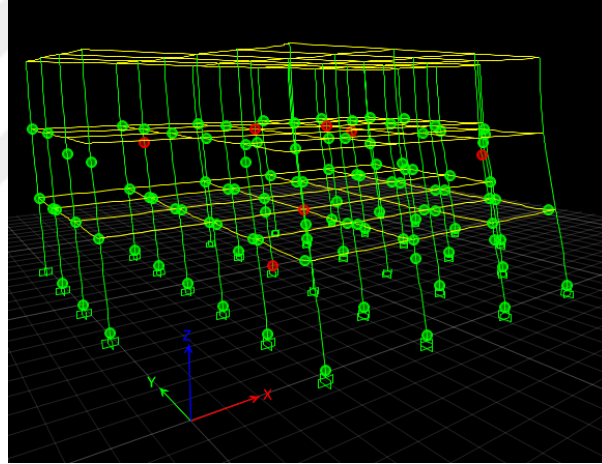
Şekil 3.59. Model1_T2' de oluşan plastik mafsallar
