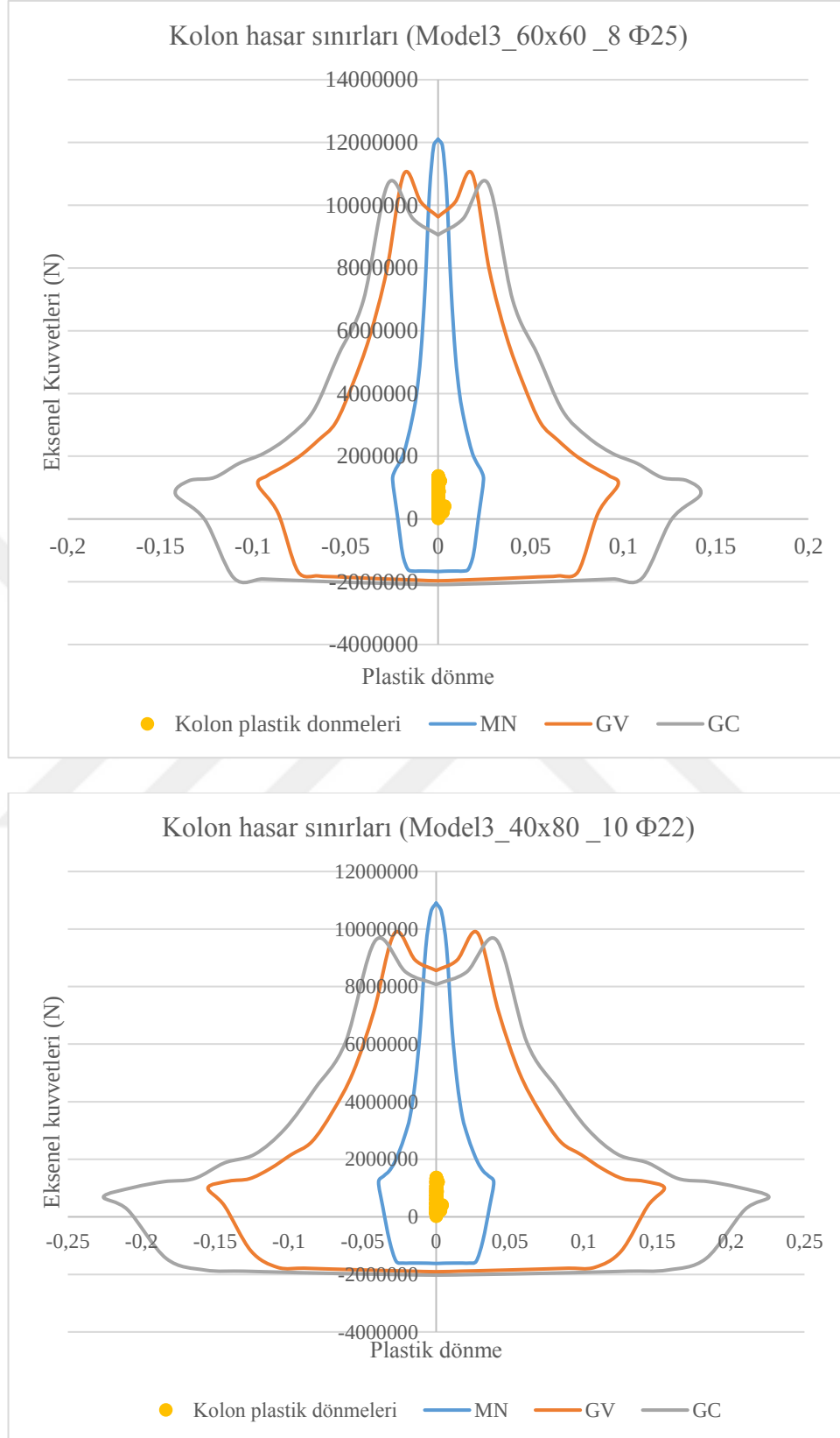
Şekil 3.108. Model3_ref'nin kare (üst) ve dikdörtgen (alt) kolonlarındaki hasarların belirlenmesi
