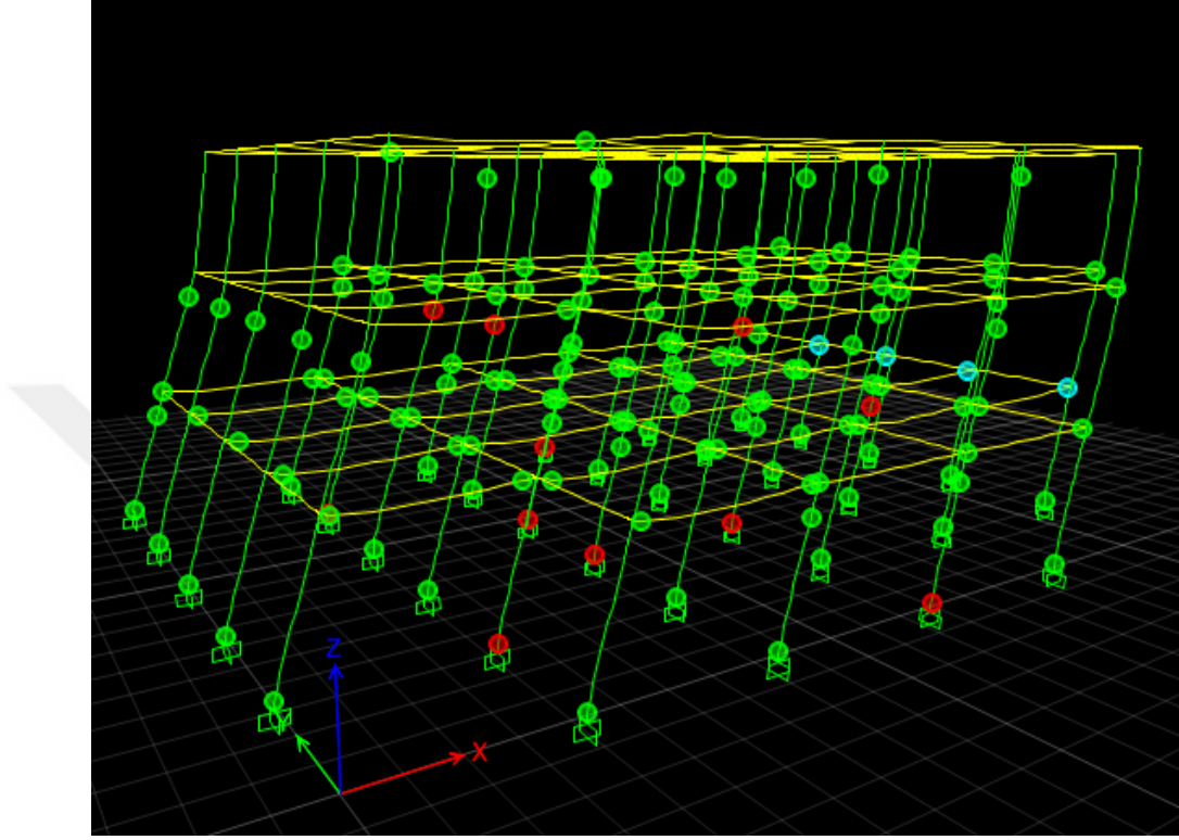
Şekil 3.50. Model1_T1' de oluşan plastik mafsallar
