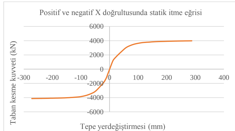
Şekil 3.85. Model2_T1 statik itme eğrisi
