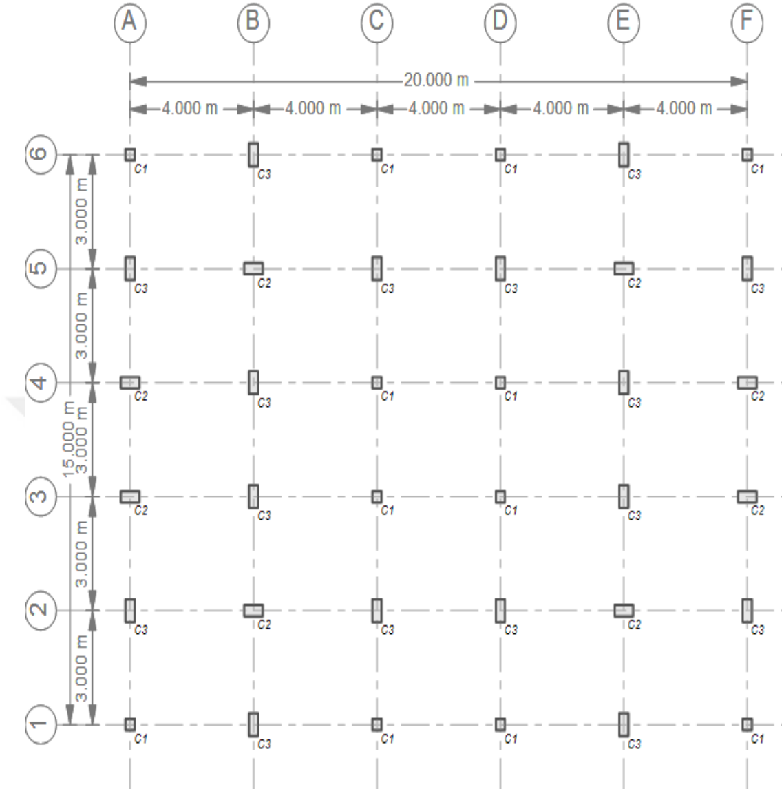
Şekil A.2. Model1_ref kat kalıp planı (kolonlar)
