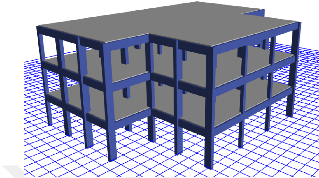
Şekil 3.6. Model 1_T2 modelinin üç boyutlu görünümü
