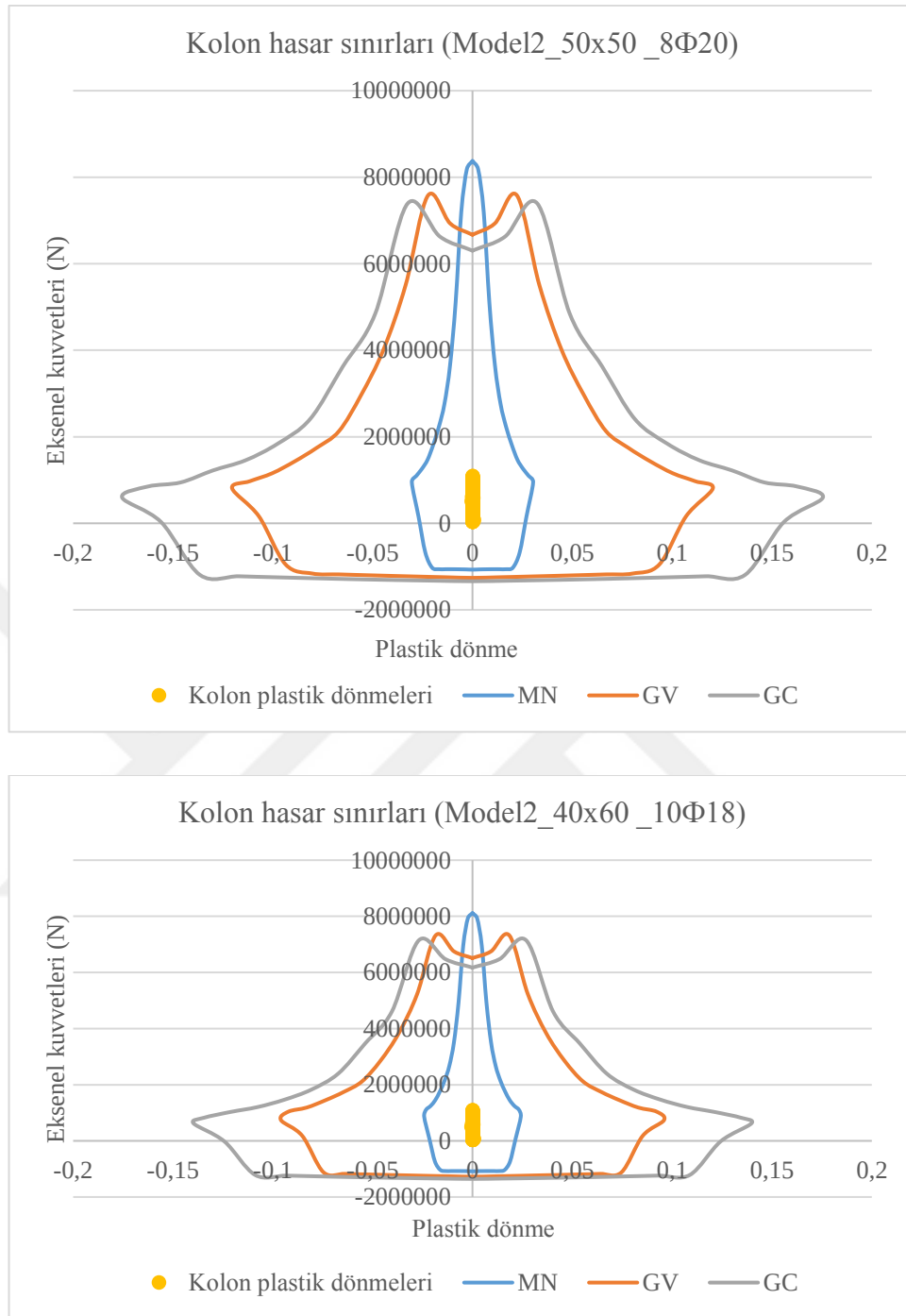
Şekil 3.90. Model2_T1'nin kare (üst) ve dikdörtgen (alt) kolonlarındaki hasarların belirlenmesi
