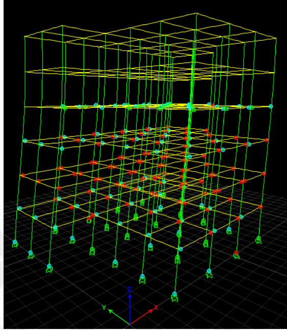
Şekil 3.98. Model2_T3' de oluşan plastik mafsallar
