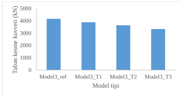
Şekil 4.3. Model3 tipi bina modelleri için taban kesme kuvvetlerinin karşılaştırması
