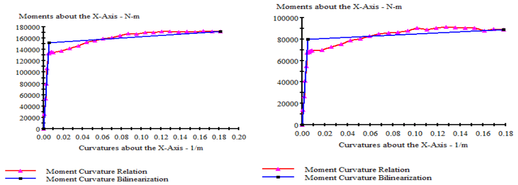
Şekil A.5. Kiriş 4B1S1 xtract programından elde edilen moment – eğrilik bağıntısı
