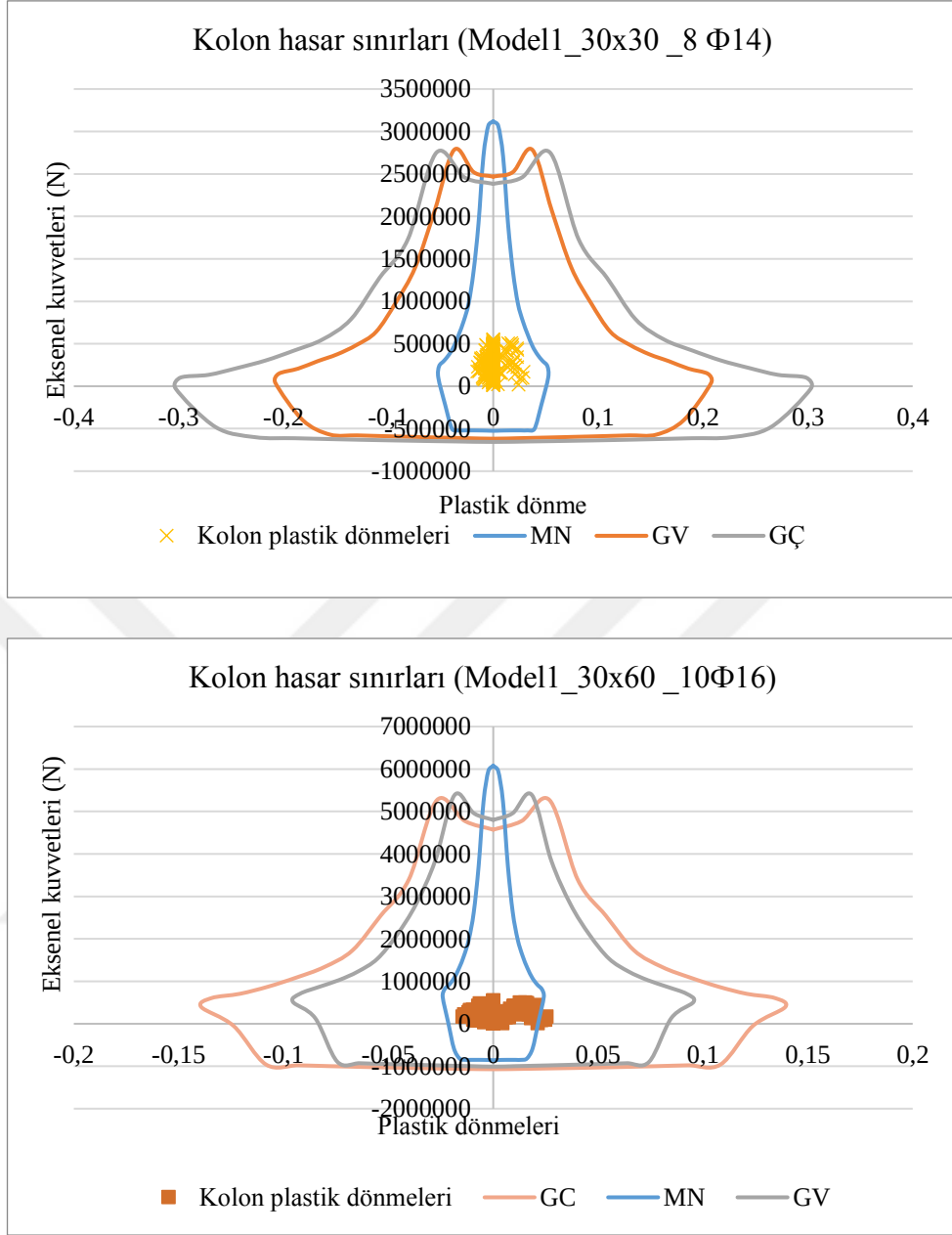
Şekil 3.63. Model1_T3'nin kare (üst) ve dikdörtgen (alt) kolonlarındaki hasarların belirlenmesi
