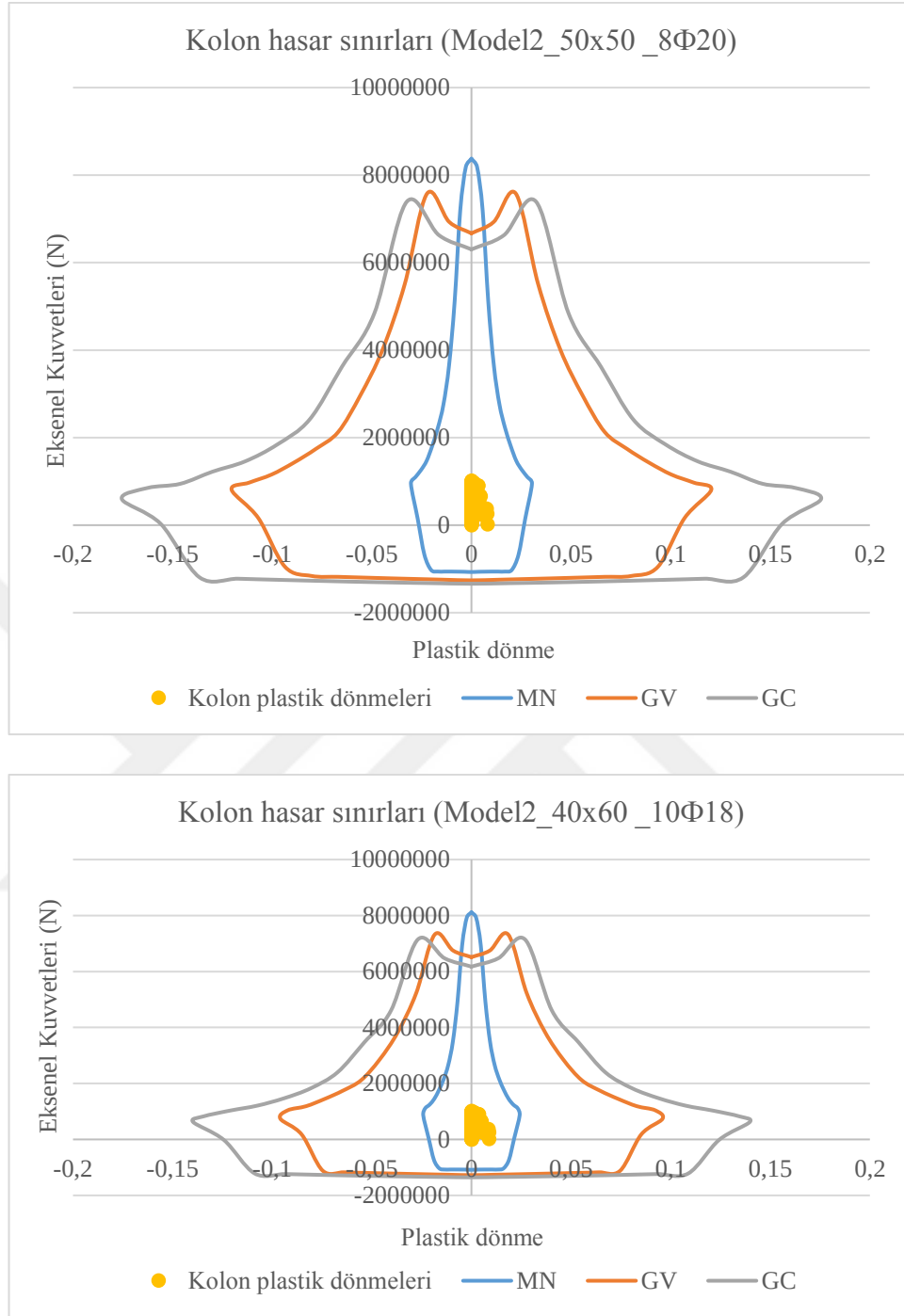
Şekil 3.99. Model2_T3'nin kare (üst) ve dikdörtgen (alt) kolonlarındaki hasarların belirlenmesi
