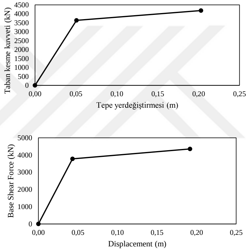
Şekil 3.68. Pozitif (üst) ve negatif (alt) X yönleri doğrusal eğriler
