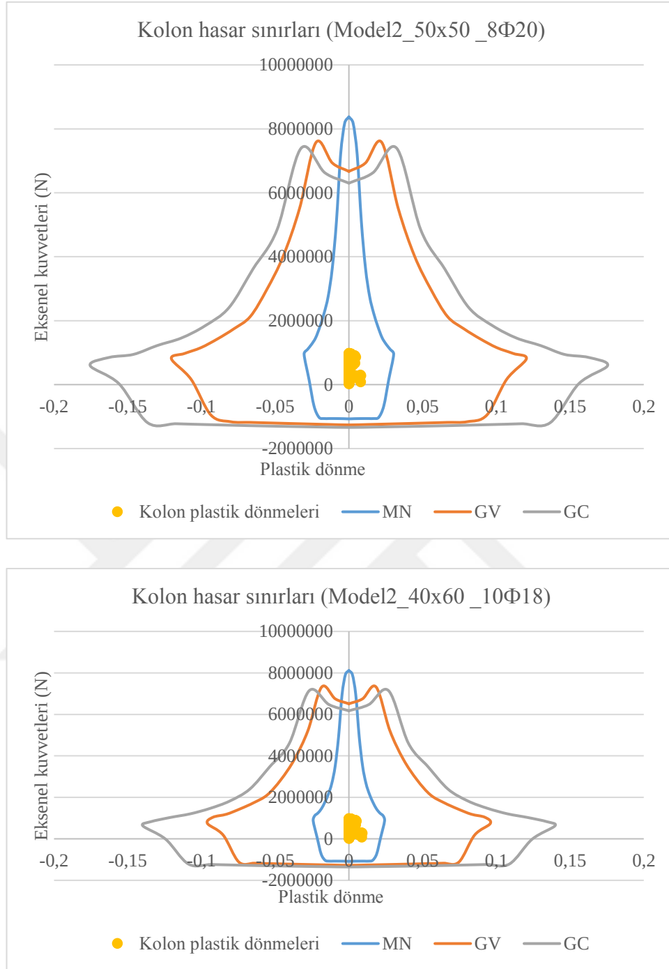
Şekil 3.87. Model2_T1'nin kare (üst) ve dikdörtgen (alt) kolonlarındaki hasarların belirlenmesi
