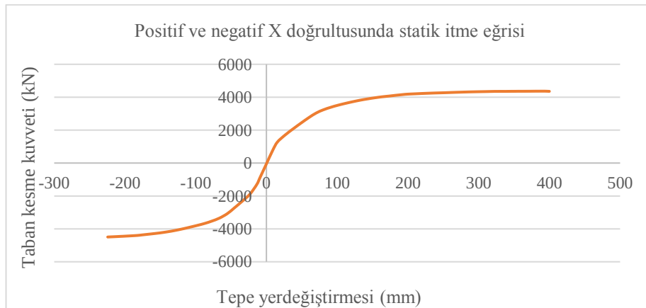
Şekil 3.121. Model3_T1 statik itme eğrisi
