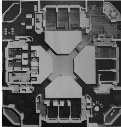
Şekil 6.7. Eskan Kuleleri kat planı. Her katta dört daire ve her dairede üç oda bulunmaktadır[68]
