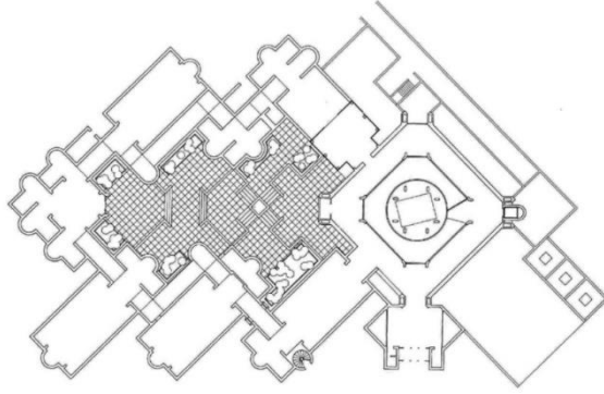
Şekil 5.37. Tahran Çağdaş Sanat Müzesinin planı [8]
