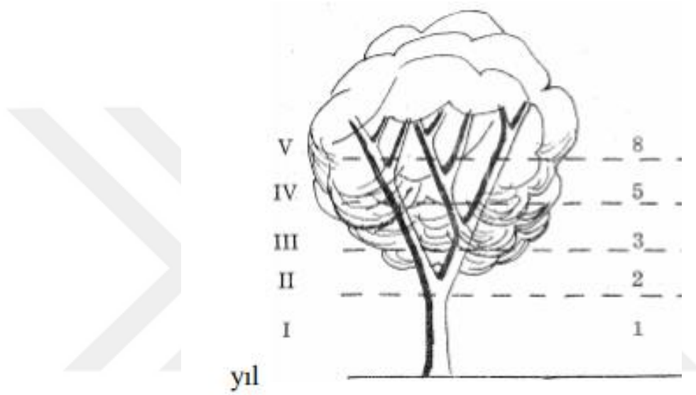
Şekil 2.2: Fibonacci Ağacı
