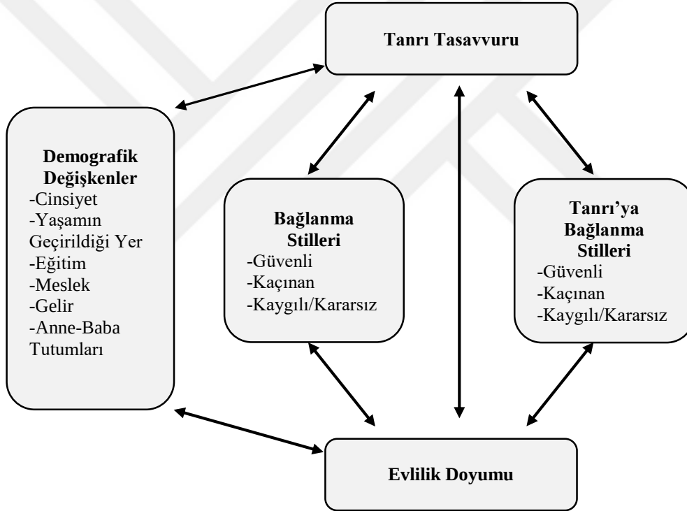
Şekil 1: Araştırma Modeli
