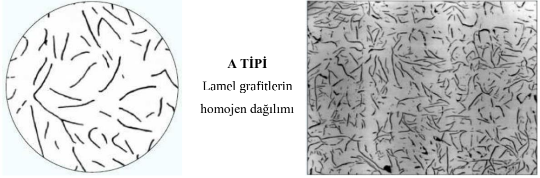
Şekil 2.2. Lamel grafitli dökme demir (A tipi)
