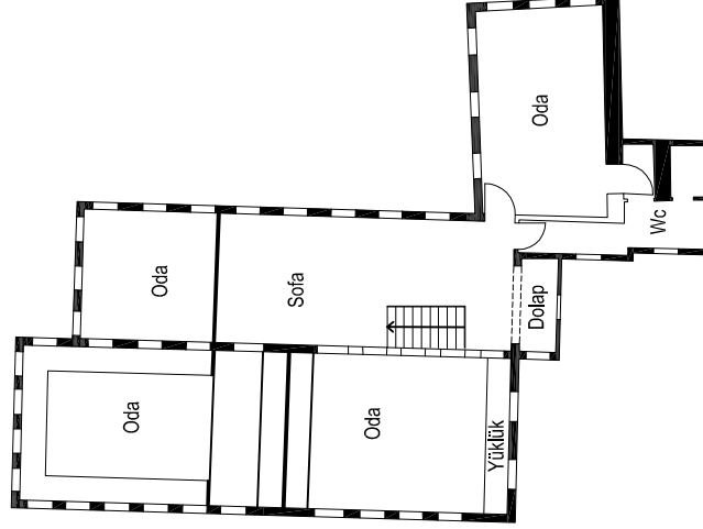
1. Kat Planı
