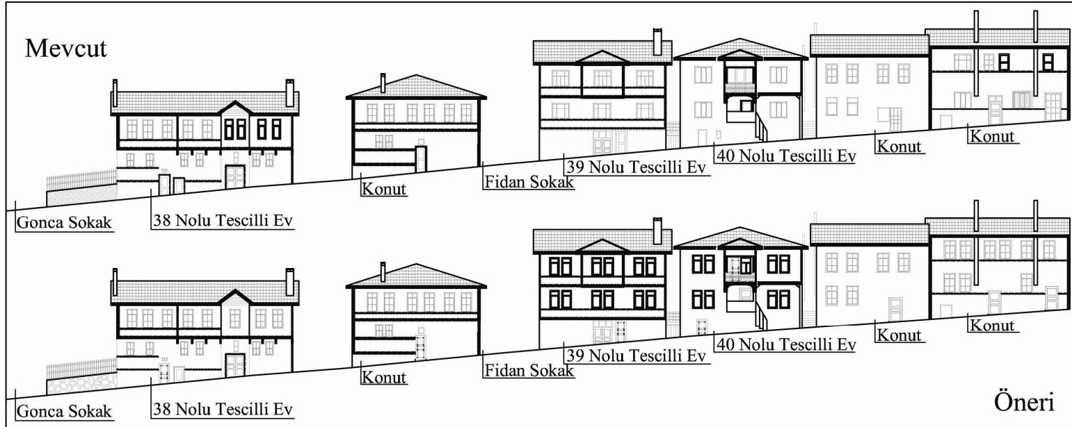
Şekil 5.8 Mimar Sinan Caddesi kuzeybatı yönü mevcut ve öneri silüeti (Çizen: Hava Kan 2009).
