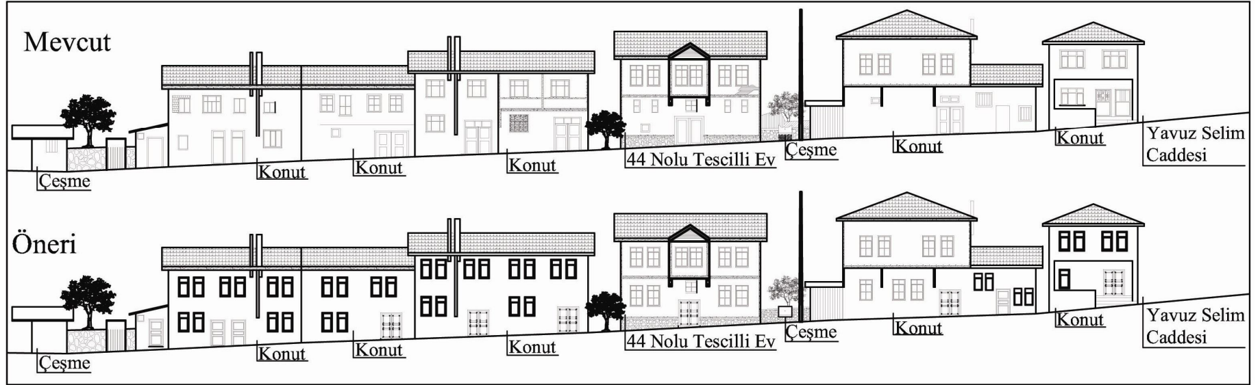
Şekil 5.12 Mimar Sinan Caddesi kuzeybatı mevcut ve öneri silüeti (Çizen: Hava Kan 2009).
