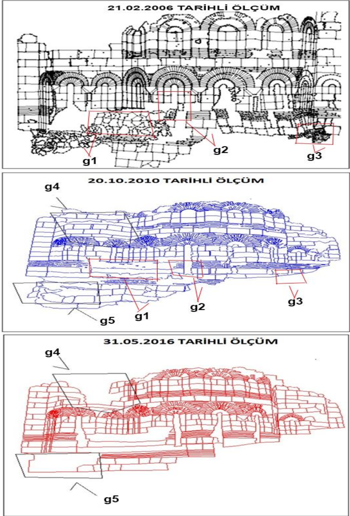
Şekil 13. Çanlı Kilise Güney Cephesi
