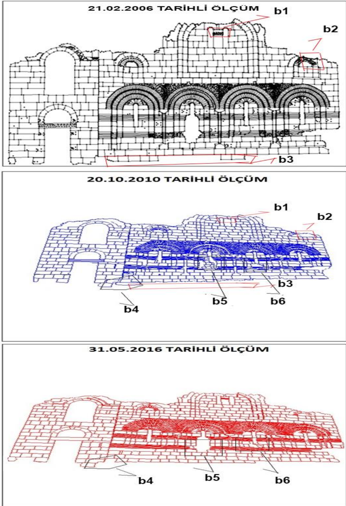
Şekil 12. Çanlı Kilise Batı Cephesi
