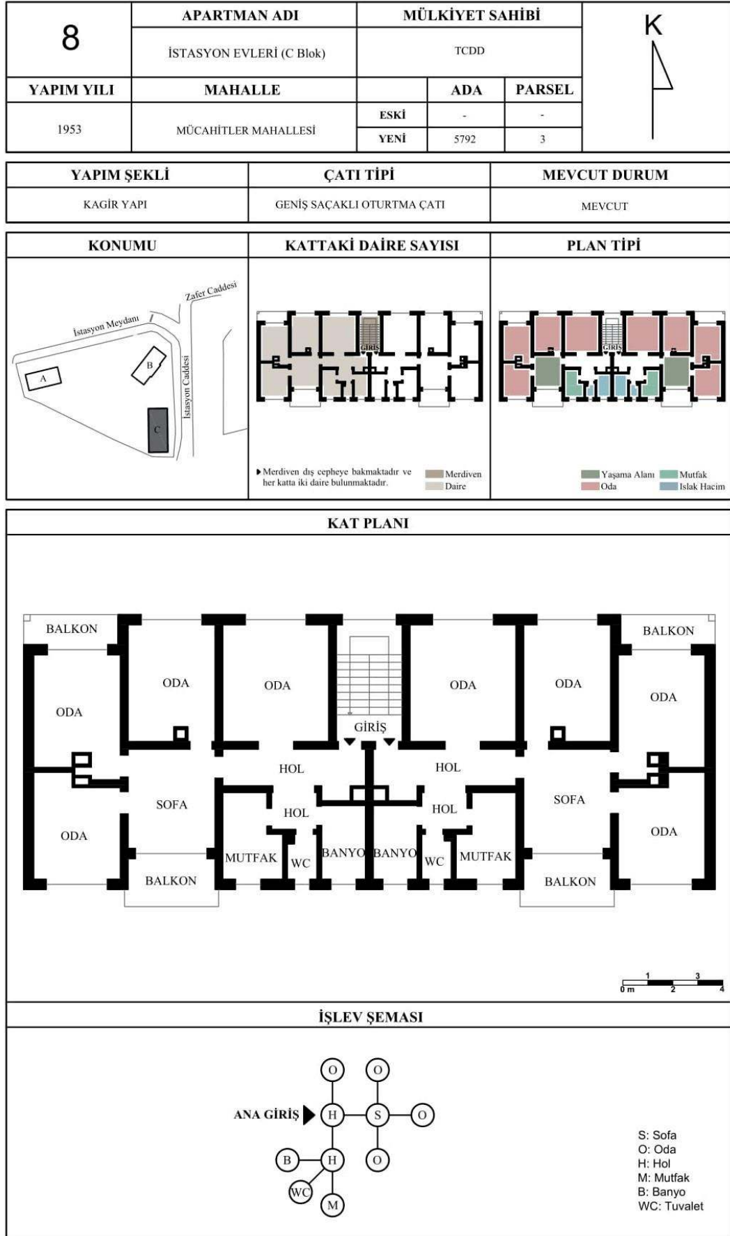
Şekil 4.27: İstasyon Evleri 5792 Ada 3 Parsel C Blok Plan Şeması (Rölöve: Açıklol, 2020)
