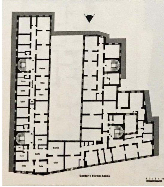
Şekil 2.32: Naib Bey Apartmanı Planı (Öncel, 2014)
