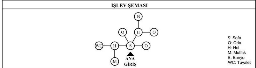
Şekil 4.17: Mahmut Ersoy Apartmanı Plan Şeması (Plan krokisi Haluk Tazebay ile çıkarılmıştır.)
