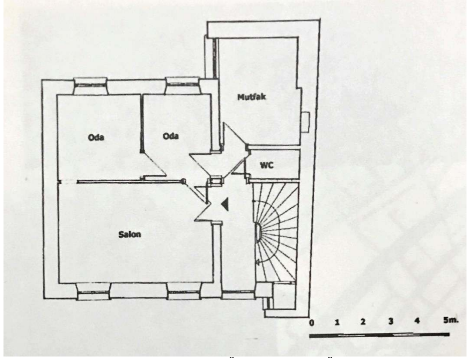
Şekil 2.29: Ara Tip Konut Örneği Kat Planı (Öncel, 2014)
