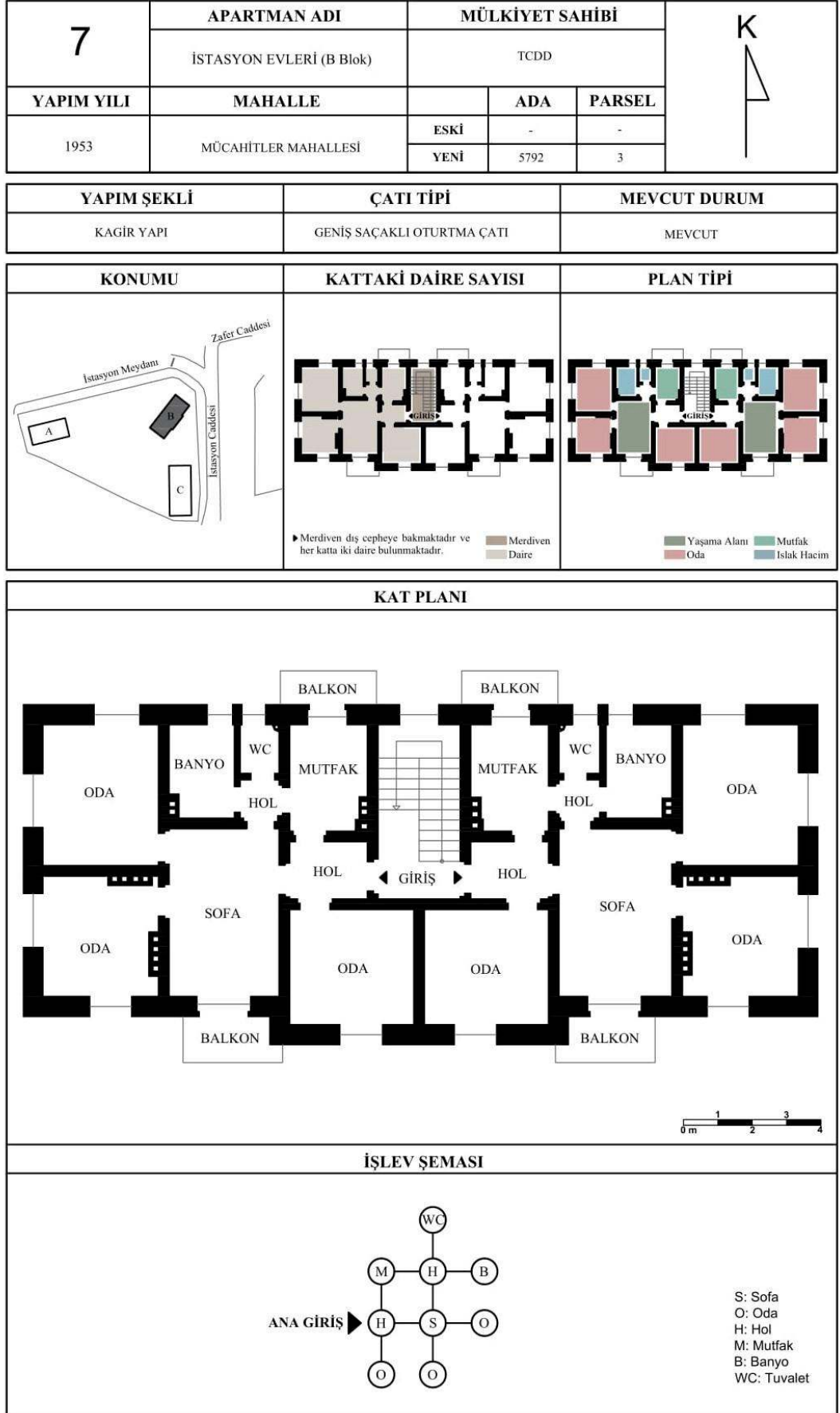
Şekil 4.25: İstasyon Evleri 5792 Ada 3 Parsel B Blok Plan Şeması (Rölöve: Açıklol, 2020)
