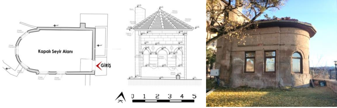
Resim 3.74. Plan, batı ve kuzey cephe, 2020
