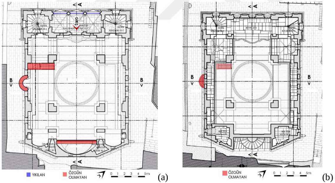
Şekil 3.23. Kilise kat planları, 2020 (KVBM) a) Zemin kat planı b) Üst kat (galeri) planı
