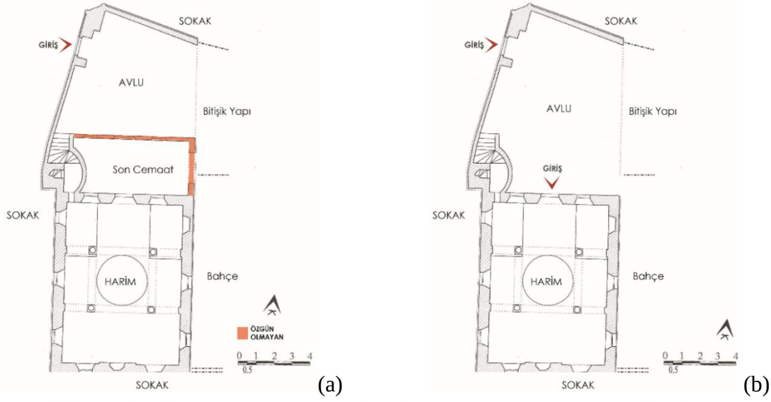
Şekil 3.20. Ali Saip Paşa Cami planı 40 a) Restorasyon öncesi kat planı b) Günümüz kat planı (özgün şema)
