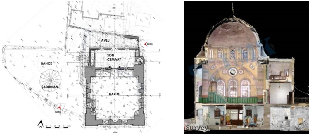
Şekil 3.4. Zemin kat planı ve 3D kesit 19
