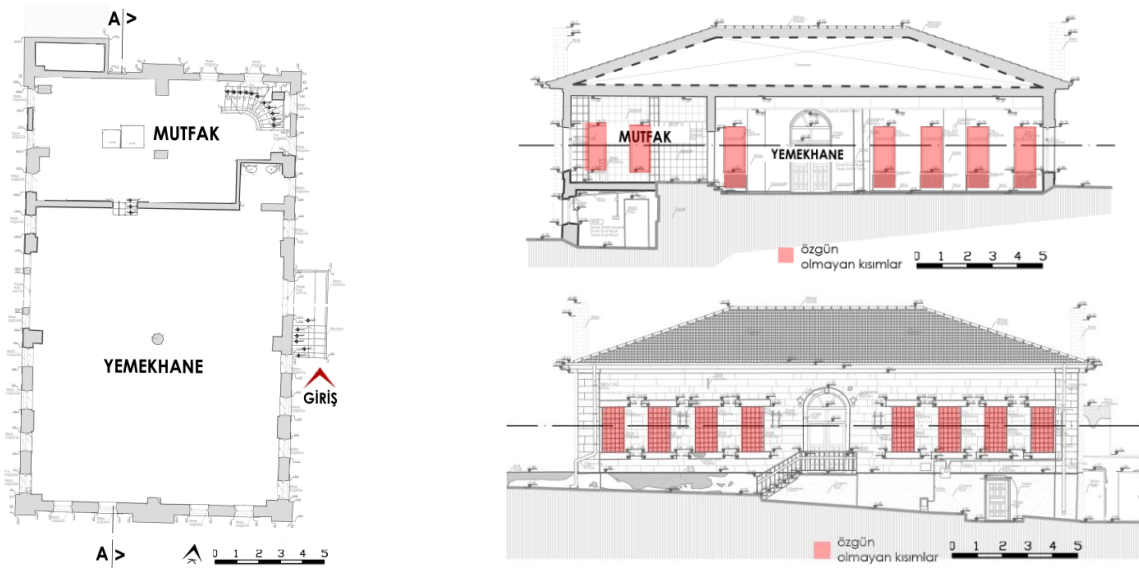
Şekil 3.41. Plan, kesit ve güney cephe 79 , 2020
