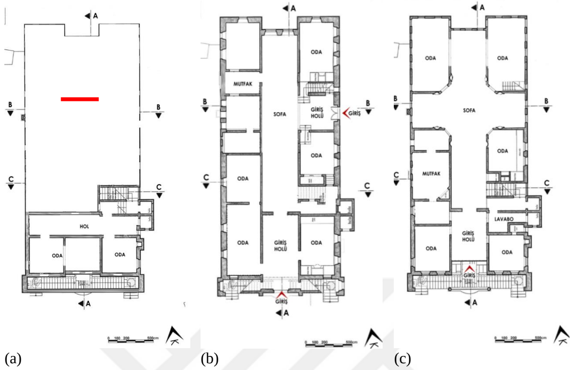
Şekil 3.16. Kat planları, 2020 35 a) Bodrum kat planı b) Zemin kat planı c) Birinci kat planı
