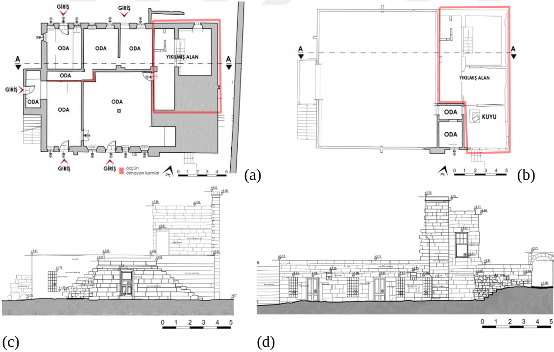
Şekil 3.38. Büyük Hastane plan ve cephe, 2020 72 a) Bodrum kat planı b) Zemin kat planı c) Batı cephe d) Güney cephe
