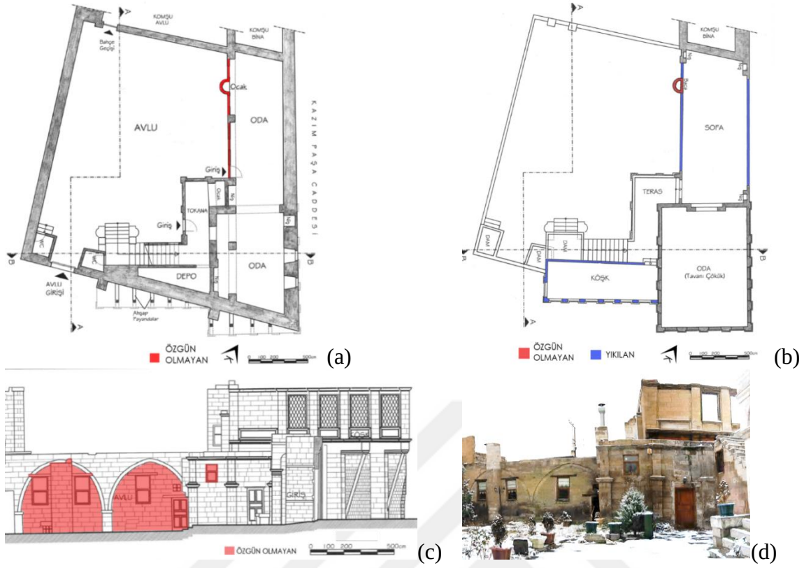
Şekil 3.17. Kat planları ve batı cephe 36 , 2020 a) Zemin kat planı b) Birinci kat planı c) A-A kesiti d) Batı cephe
