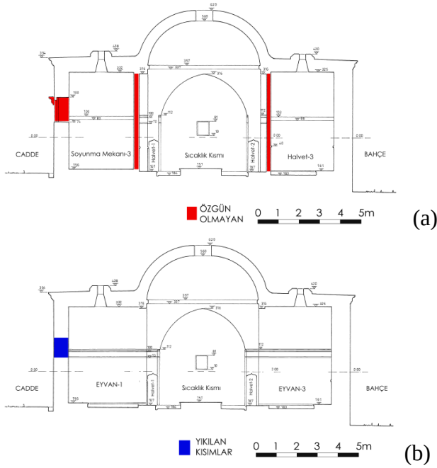
Şekil 3.6. A-A kesiti (KVBM Arşivi, 1981) a) 1981 yılı b) Restitüsyon projesi
