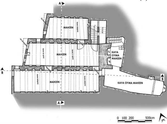
Şekil 3.25. Okutan Konağı kat planları 48 a) Birinci kat planı b) Zemin kat planı c) Bodrum kat planı
