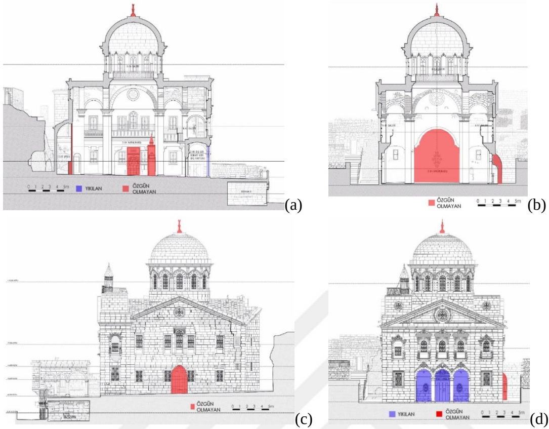
Şekil 3.24. Panagia Kilisesi kesit ve cepheleri, 2020 (KVBM) a) A-A kesiti b) B-B kesiti c) Güneybatı cephe d) Kuzeybatı cephe
