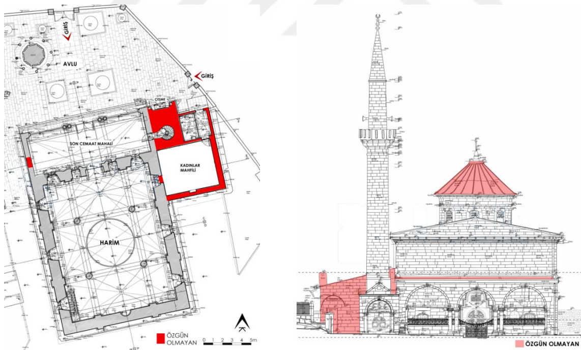
Şekil 3.13. Plan ve kuzey görünüş, 2020 31
