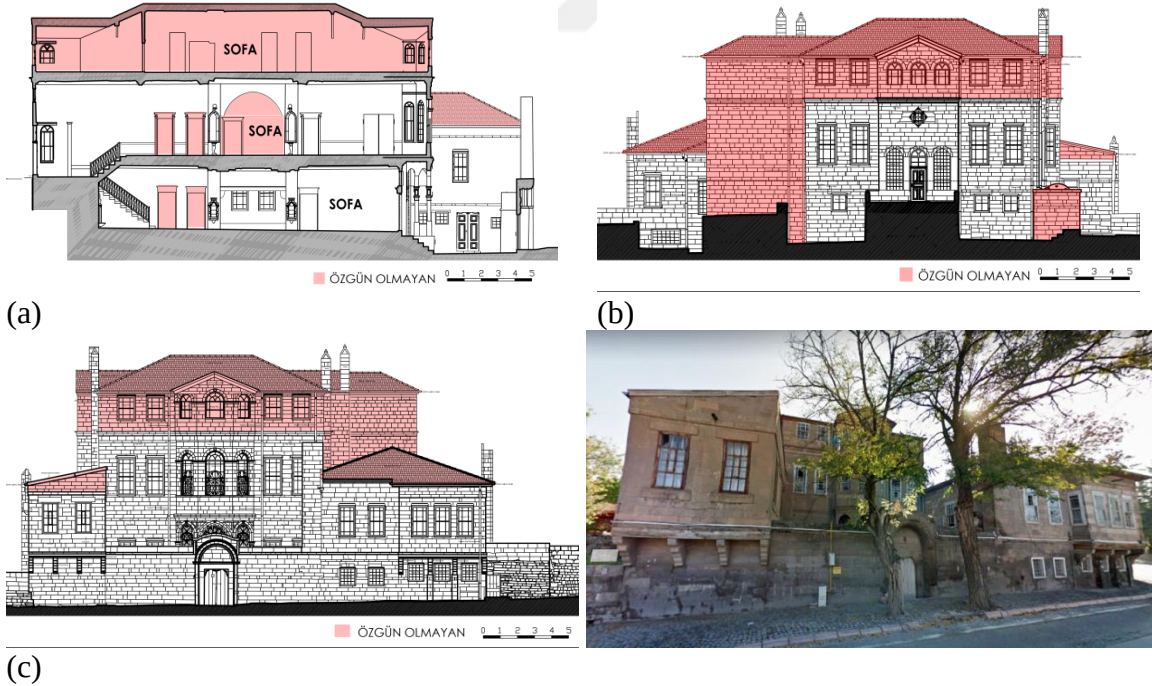
Şekil 3.34. Kesit ve cepheler, 2020 a) A-A kesiti b) Güneydoğu cephesi c) Kuzeybatı cephesi (Atatürk Caddesi'nden görünüm)
