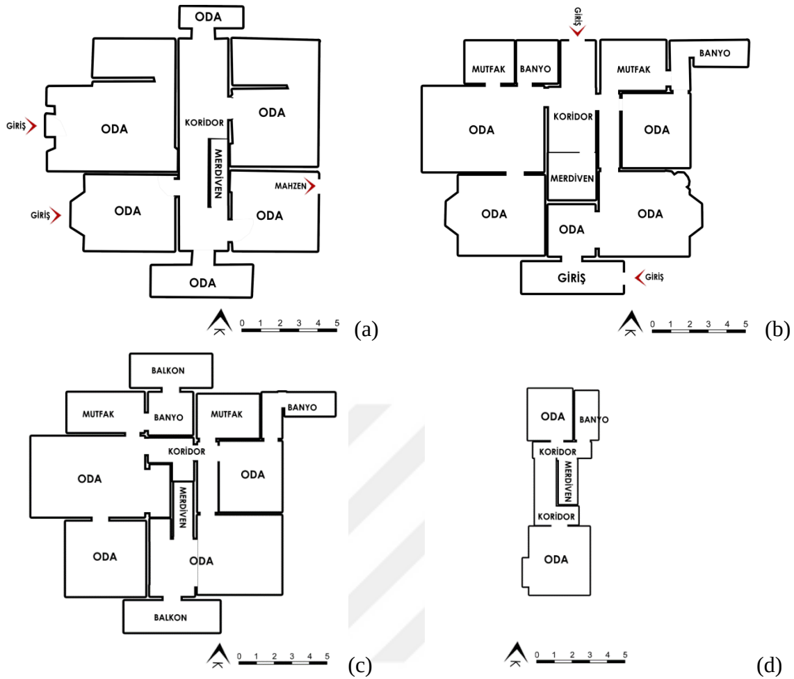
Şekil 3.40. Birinci ve çatı kat plan krokileri, 2020 76 a) Bodrum kat krokisi b) Zemin kat krokisi c) Birinci kat krokisi d) Çatı katı krokisi
