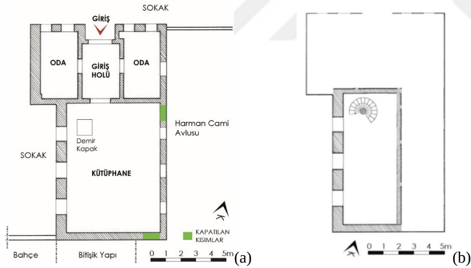
Şekil 3.14. Kat planı, 2020 a) Zemin kat planı b) Bodrum kat planı
