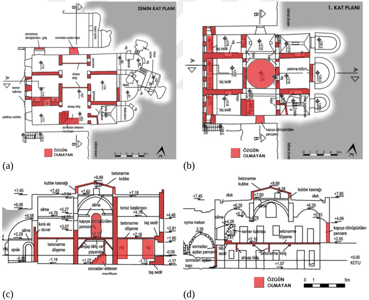
Şekil 3.10. Kat planları ve kesitler 24 a) Zemin kat planı b) Birinci kat planı c) A-A kesiti d) B-B kesiti
