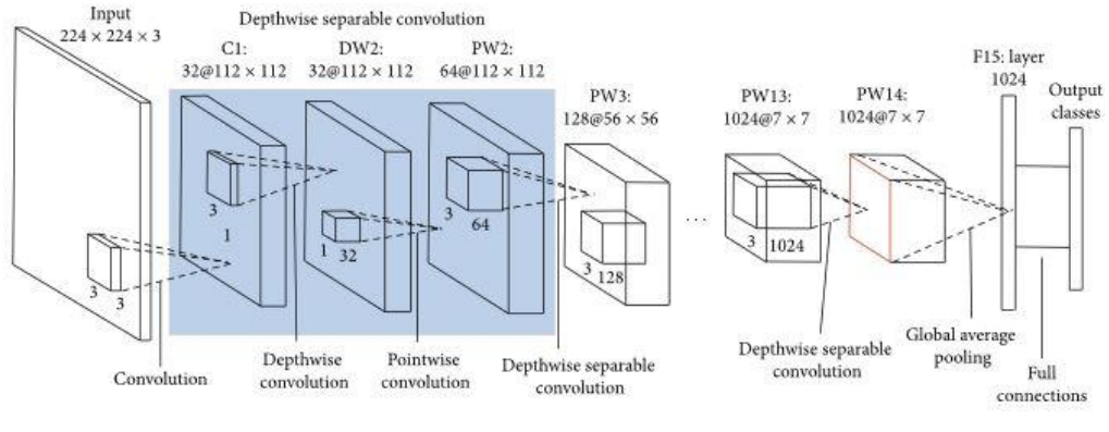
Şekil 3.4. MobileNet ağ mimarisi (Singhal, 2020)
