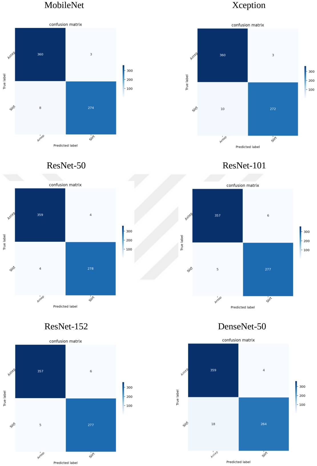
Şekil 4.4. Modellerin karışıklık matrisi grafikleri
