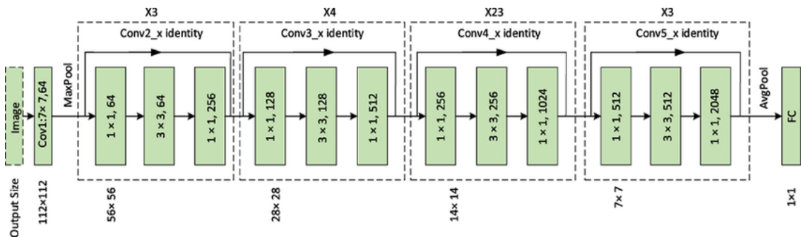
Şekil 3.6 ResNet 101 Mimarisi
