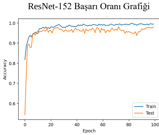
Şekil 4.2. Modellerin başarı performansları ve iterasyon değerleri
