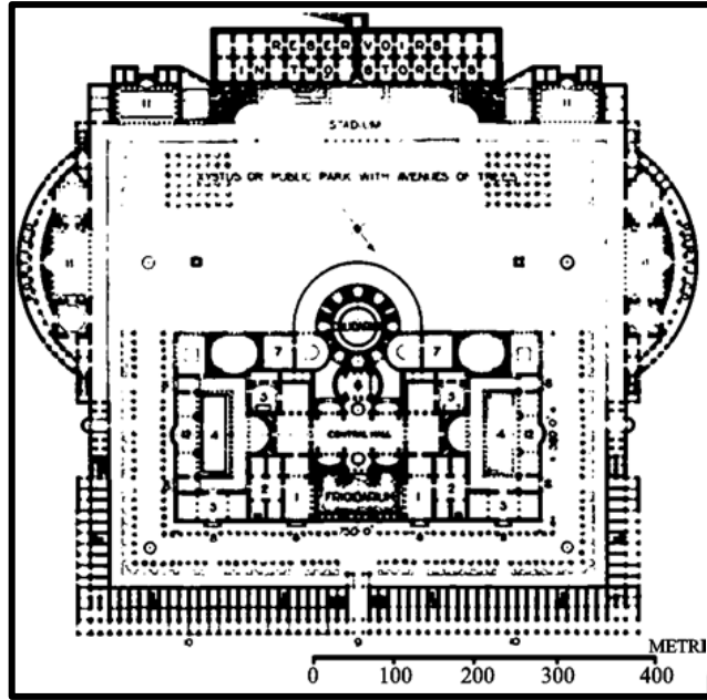
Şekil 2.2. Caracalla Hamamı Plan Şeması (Eyice,1997)
