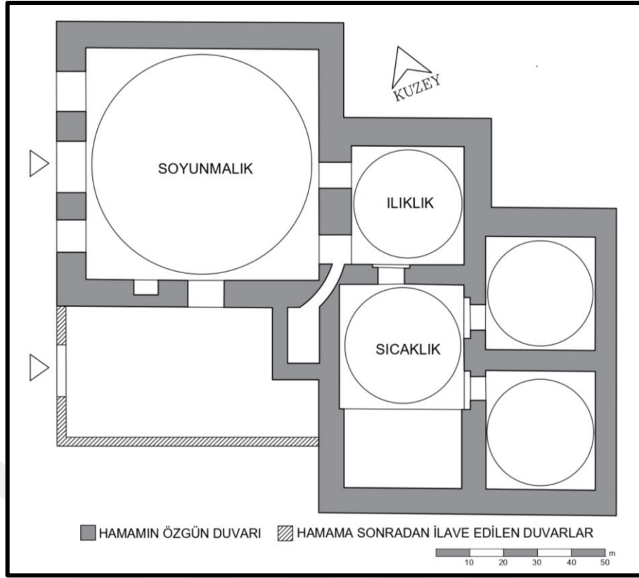
Şekil 3.54. Yıldırım Hamamı'nın Günümüzdeki Durumunun Planı (Asiltürk, alan çalışması ile çizilmiştir.)
