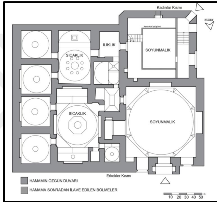
Şekil 3.4. Çakırağa (Çakır) Hamamı'nın Günümüzdeki Durumunun Planı (Asiltürk, alan çalışması ile çizilmiştir.)
