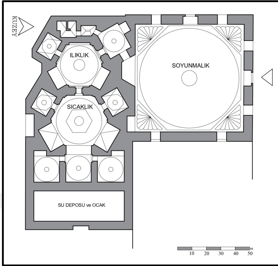
Şekil 3.88. İncirli Hamamı Restitüsyon Planı (Asiltürk, K.T.V.K.K. Arşivinden alınarak çizilmiştir.)
