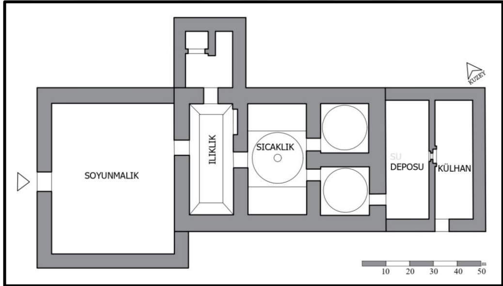
Şekil 4.109. Kiremitçi Sinan Bey Hamamı Restitüsyon Planı (Asiltürk, E. Şehitoğlu ve E. Ayverdi'den alınarak çizilmiştir.)
