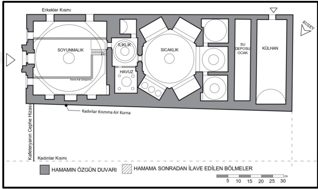
Şekil 3.39. Nasuhpaşa Hamamı'nın Günümüzdeki Planı (Asiltürk, alan çalışması ile çizilmiştir.)
