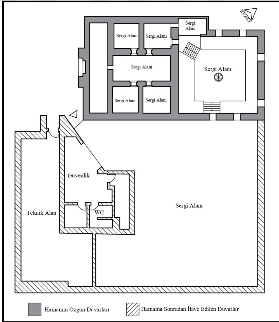
Şekil 3.205. Umurbey Hamamı Restorasyon Planı (Yangın Kaçış Planından alınarak çizilmiştir.)
