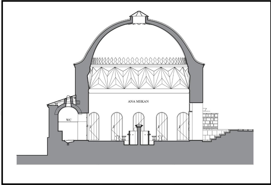
Şekil 3.70. Cık Cık Hamamı Restorasyon Projesi A-A Kesiti (Asiltürk, Bursa Büyükşehir Belediyesi Arşivinden alınarak çizilmiştir.)
