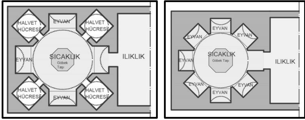
Şekil 2.14. Sekizgen yıldızvari sıcaklıklı plan tipi (Eyice, 1997; Düzenleyen: Demir, 2019)
