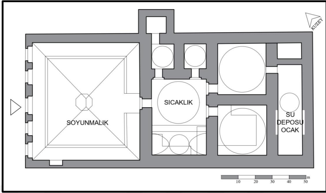
Şekil 3.211. Yeşil Hamamı Planı (Şehitoğlu ve E. H. Ayverdi'den alınarak çizilmiştir.)
