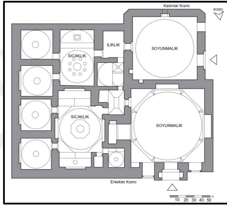
Şekil 3.3. Çakırağa (Çakır) Hamamı Restitüsyon Planı (Şehitoğlu ve E. H. Ayverdi'den alınarak çizilmiştir.)
