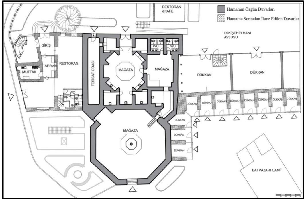
Şekil 3.216. Batpazarı (Davutpaşa) Hamamı Restorasyon Planı (Asiltürk, Bursa Büyükşehir Belediyesi Arşivinde alınarak çizilmiştir.)
