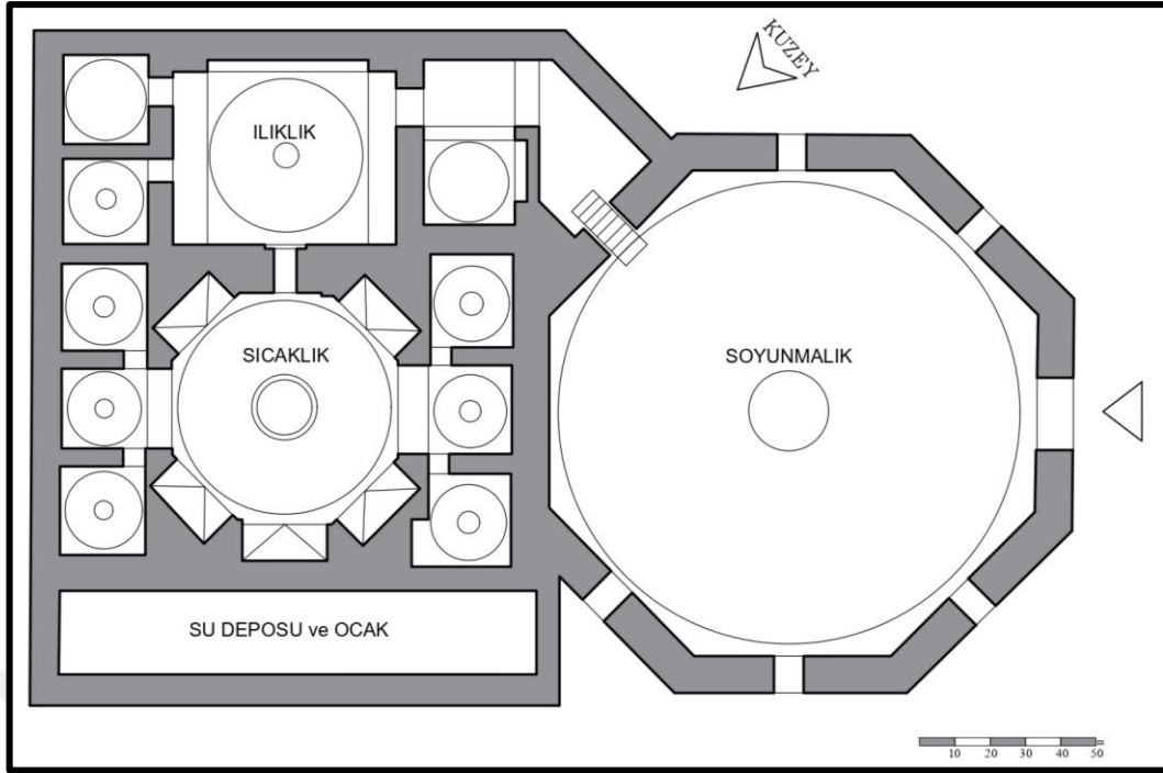
Şekil 3.214. Batpazarı (Davutpaşa) Hamamı Restitüsyon Planı (Asiltürk, Şehitoğlu'ndan alınarak çizilmiştir.)
