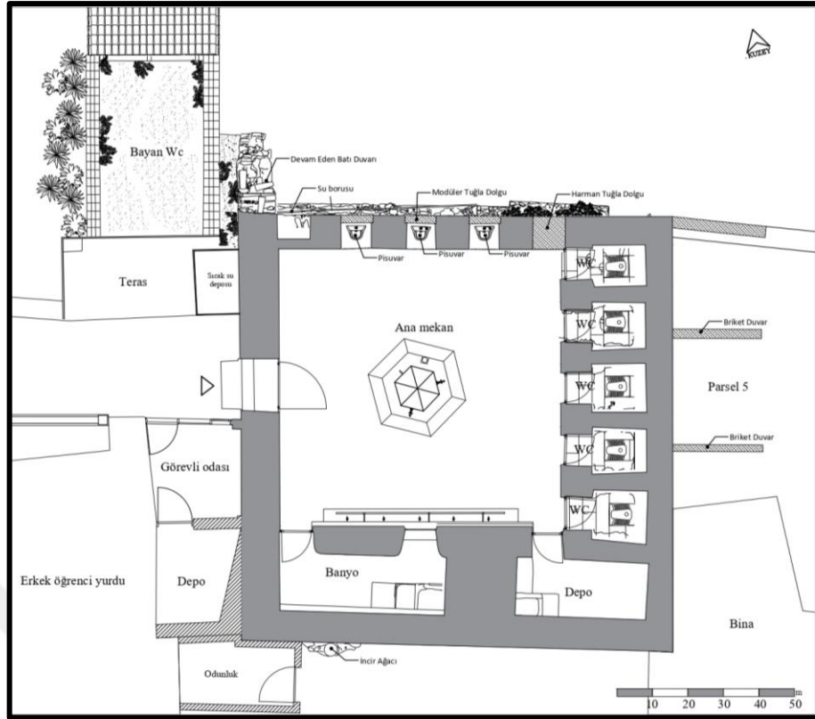
Şekil 3.66. Cık Cık Hamamı 2010 Yılı Rölöve Planı (Asiltürk, Bursa Büyükşehir Belediyesi Arşivinden alınarak çizilmiştir.)
