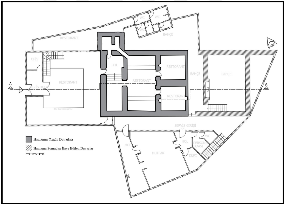
Şekil 3.111. Kiremitçi Sinan Bey Hamamı Restorasyon Planı (Asiltürk, Bursa Büyükşehir Belediyesi Arşivinde alınarak çizilmiştir.)
