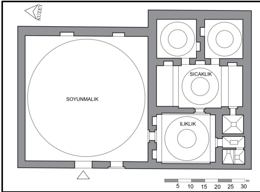
Şekil 3.29. Haydarhane Hamamı Restitüsyon Planı (Asiltürk, Şehitoğlu'ndan alınarak çizilmiştir.)
