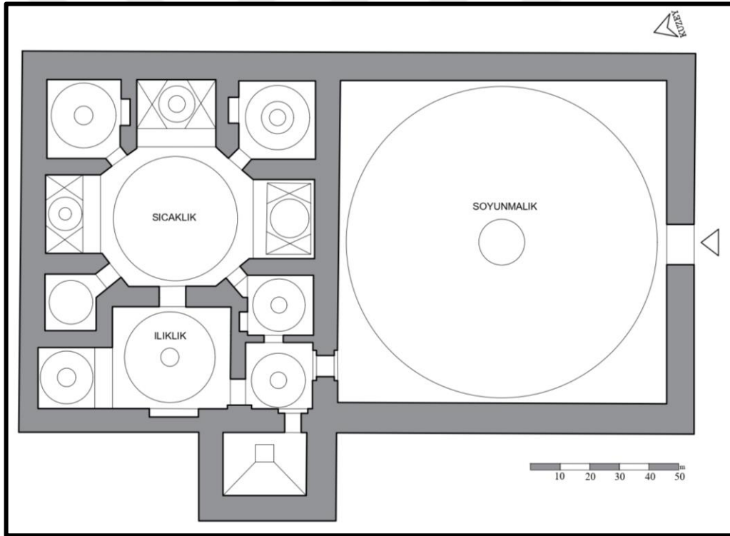
Şekil 3.167. Perşembe (Kadı) Hamamı Restitüsyon Planı (Asiltürk, E. Şehitoğlu ve E. Ayverdi'den alınarak çizilmiştir.)
