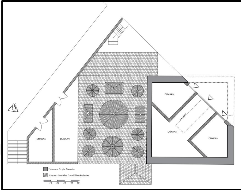
Şekil 3.172. Perşembe (Kadı) Hamamı'nın Üst Kotunun Günümüzdeki Planı (Asiltürk, Alan çalışması ile çizilmiştir.)
