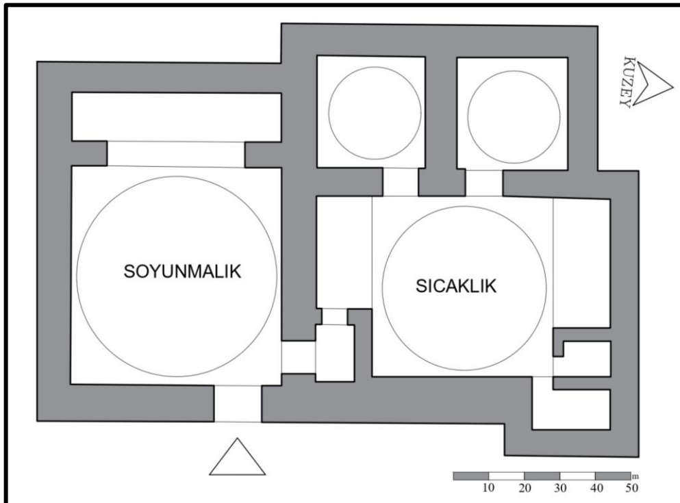
Şekil 3.187. Şengül Hamamı Restitüsyon Planı (Asiltürk, E. Şehitoğlu ve E. Ayverdi'den alınarak çizilmiştir.)
