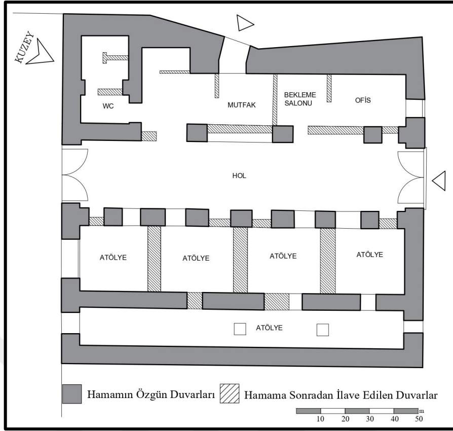
Şekil 3.126. Muallimzade Hamamı'nın Günümüzdeki Durumunun Planı (Asiltürk, Tahliye planından alınarak çizilmiştir.)
