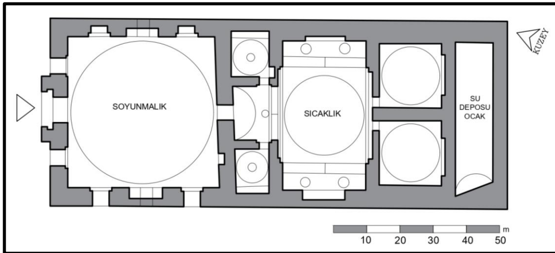
Şekil 3.59. Başçı İbrahim Hamamı’nın Restitüsyon Planı (Asiltürk, Şehitoğlu’ndan alınarak çizilmiştir.)
