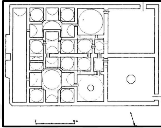
Şekil 2.4. Konya Sahip Ata Hamamı Plan Şeması (Karpuz,2009)
