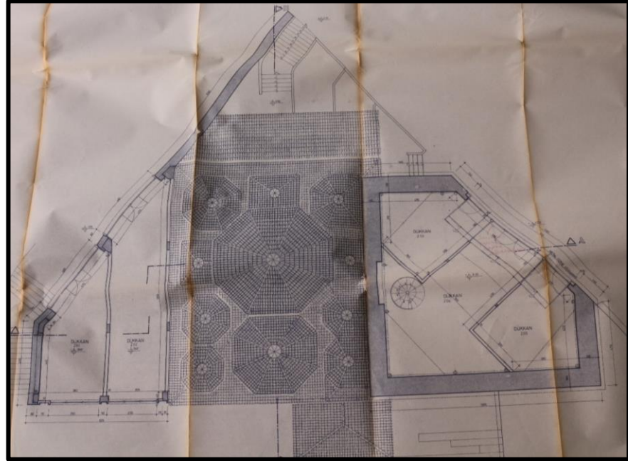
Şekil 3.169. Perşembe (Kadı) Hamamı'nın 1991 Yılında Çizilen Üst Kotunun Restorasyon Planı (K.T.V.K.K. Arşivi, 2023)
