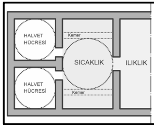
Şekil 2.21. Ortası kubbeli, enine sıcaklıklı ve çift halvetli plan tipi (Eyice, 1997; Düzenleyen: Demir, 2019).
