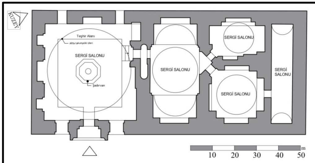
Şekil 3.82. Çandarlı İbrahimpasha Hamamı Restorasyon Planı (Bursa K.T.V.K.K arşivinden alınarak çizilmiştir.)
