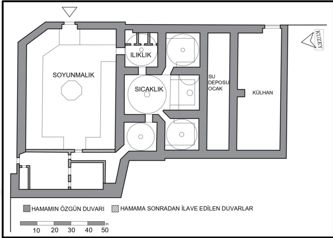
Şekil 3.22. Eski Orhan Hamamı'nın Planı (Asiltürk, Şehitoğlu'ndan geliştirerek çizilmiştir.)
