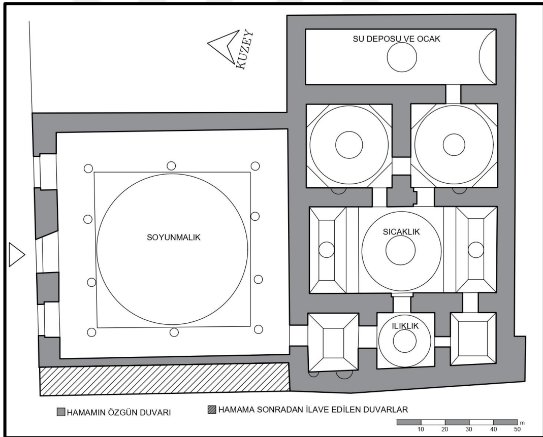
Şekil 3.50. Yahudiler Hamamı Planı (Asiltürk, Şehitoğlu'ndan alınarak çizilmiştir.)
