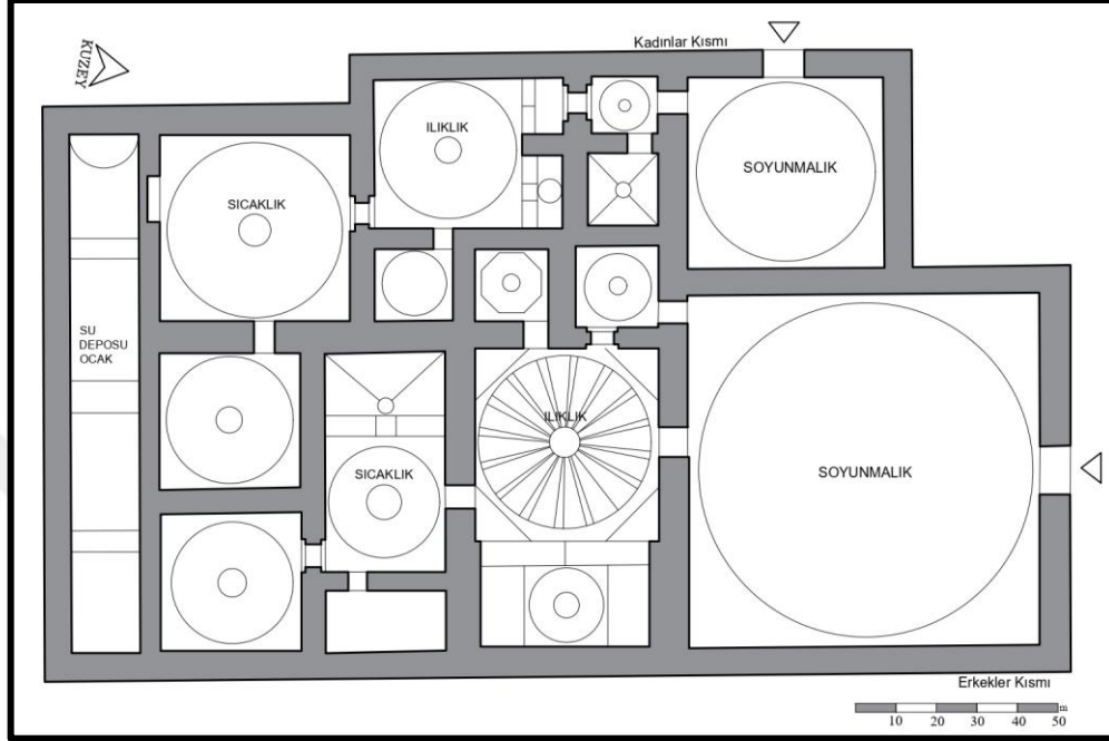
Şekil 3.193. Tavukpazarı (Meyhaneli) Hamamı Restitüsyon Planı (Asiltürk, E. Şehitoğlu ve E. Ayverdi'den alınarak çizilmiştir.)
