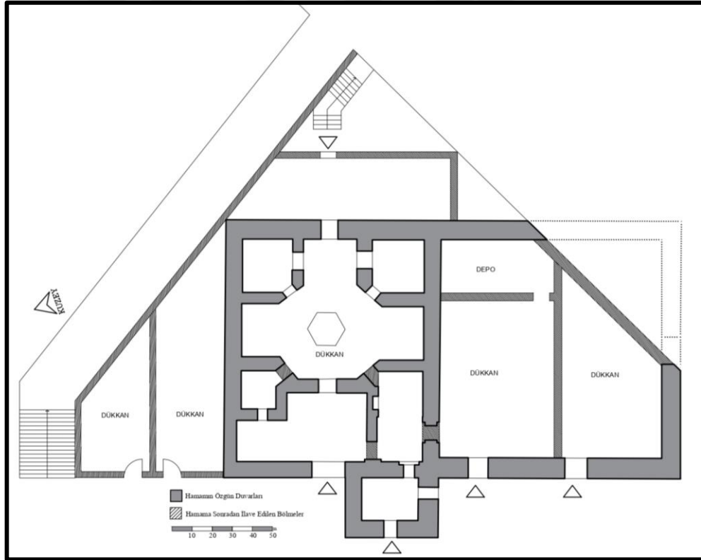
Şekil 3.171. Perşembe (Kadı) Hamamı'nın Alt Kotunun Günümüzdeki Planı (Asiltürk, Alan çalışması ile çizilmiştir.)
