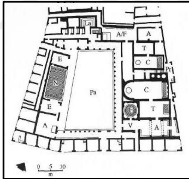
Şekil 2.1. Pompei Stabia Hamamı (Eyice,1997)
