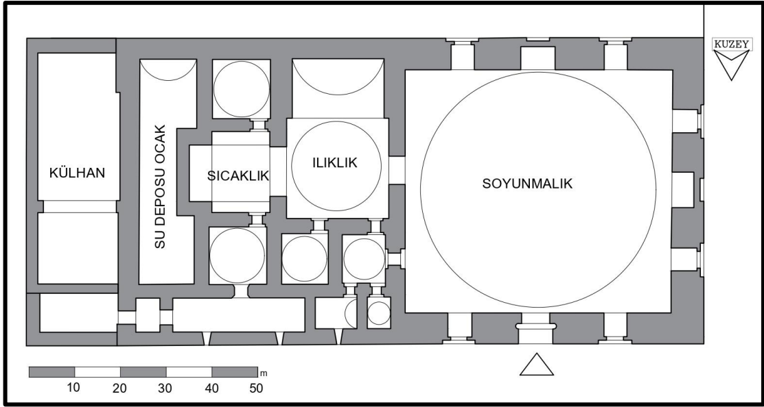
Şekil 3.15. Demirtaş Hamamı'nın Restitüsyon Planı (Şehitoğlu'ndan geliştirilerek çizilmiştir.)
