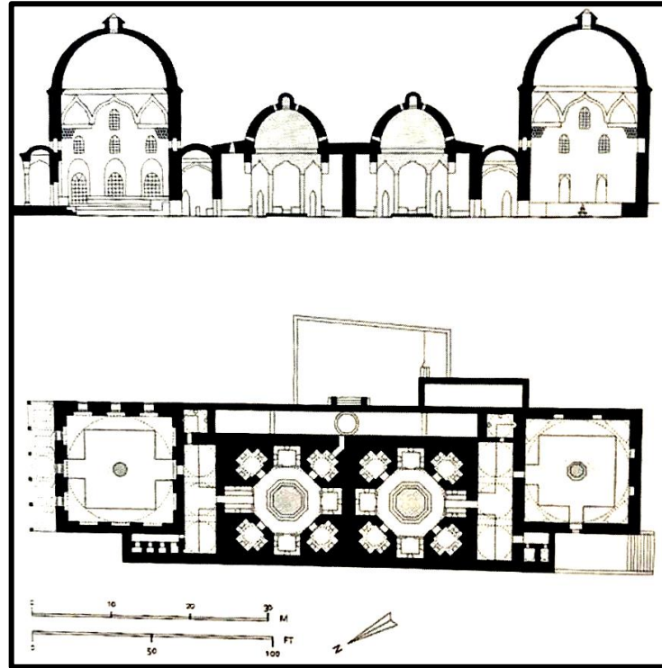
Şekil 2.6. Haseki Hürrem Sultan Hamamı Planı ve Kesiti (Yegül, 2012)
