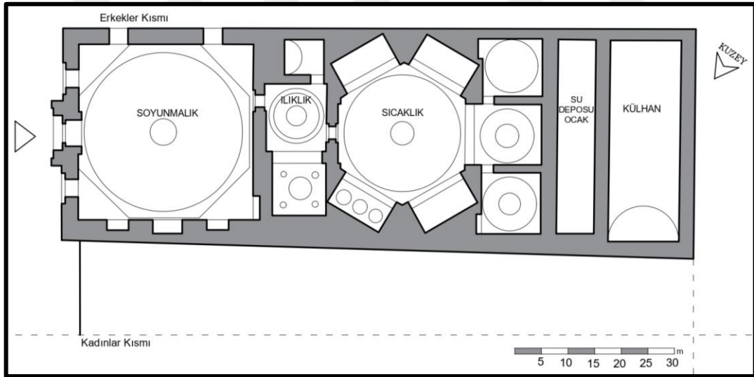
Şekil 3.38. Nasuhpaşa Hamamı Planı (Asiltürk, Şehitoğlu'ndan geliştirerek çizilmiştir.)
