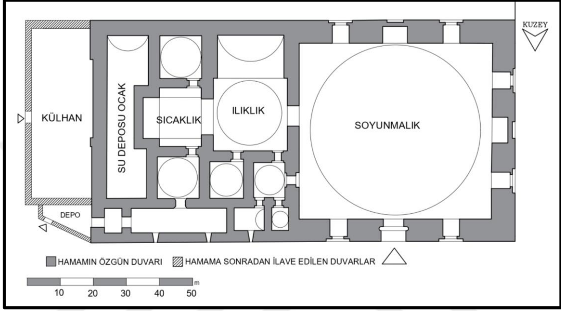
Şekil 3.17. Demirtaş Hamamı'nın Günümüzdeki Durumunu Planı (Asiltürk, alan çalışması ile çizilmiştir.)
