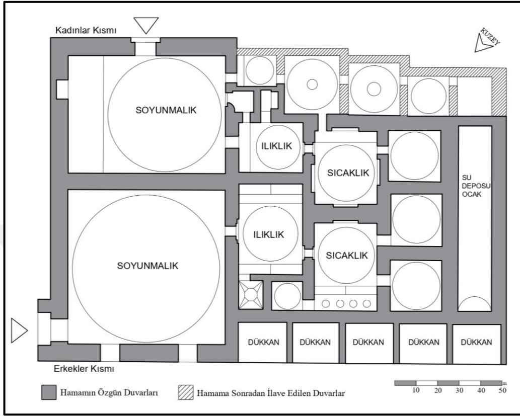
řekil 3.101. Kayhan Hamamı 2010 Yılı R l ve Planı (Asilt rk, E. řehitođlu ve E. Ayverdi'den alınarak  izilmiřtir.)
