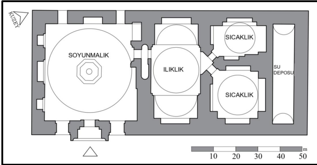
Şekil 3.81. Çandarlı İbrahimpasha Hamam Rölöve Planı (Bursa K.T.V.K.K arşivinden alınarak çizilmiştir.)
