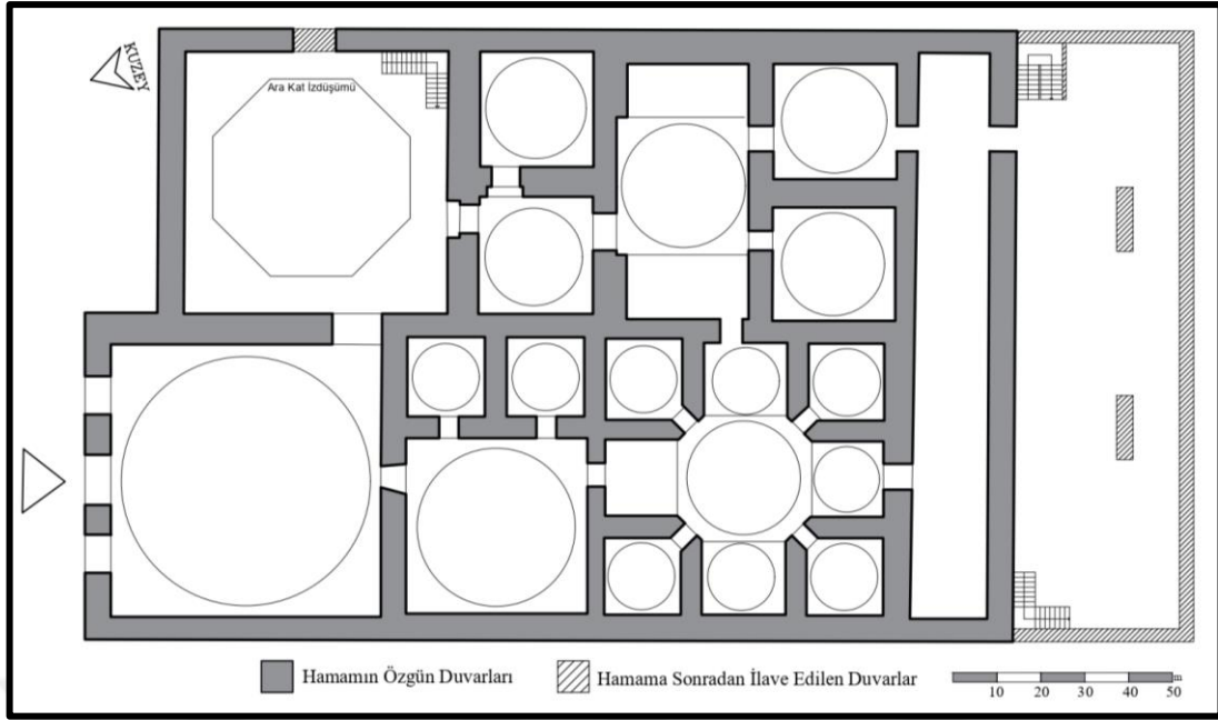
Şekil 3.143. Nalıncılar Hamamı'nın Günümüzdeki Planı (Asiltürk, Alan çalışması ile çizilmiştir.)
