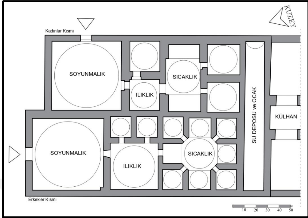
Şekil 3.142. Nalıncılar Hamamı Restitüsyon Planı (Asiltürk, E. Şehitoğlu ve E. Ayverdi'den alınarak çizilmiştir.)
