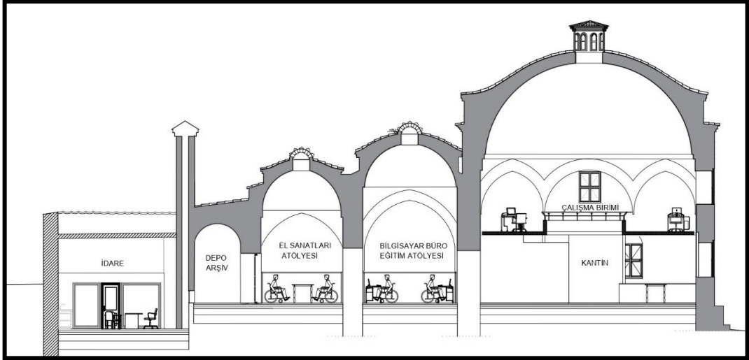
Şekil 3.134. Muradiye Hamamı Restorasyon Projesi A-A Kesiti (Bursa Büyükşehir Belediyesi Arşivinden alınarak çizilmiştir.)
