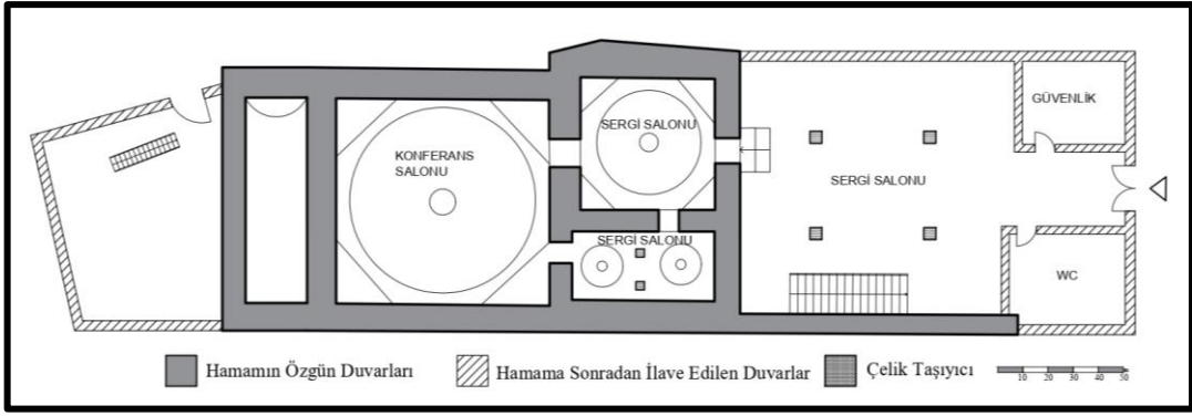
Şekil 3.97. İnebey Hamamı Restorasyon Planı (Asiltürk, Şantiyede bulunan belgeler referans alınarak çizilmiştir.)
