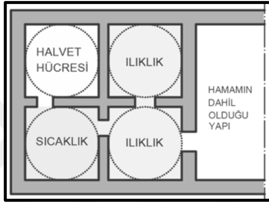
Şekil 2.22. Ilıklık, sıcaklık ve halvetin eş odalar halinde olduğu plan tipi (Eyice, 1997; Düzenleyen: Demir, 2019)
