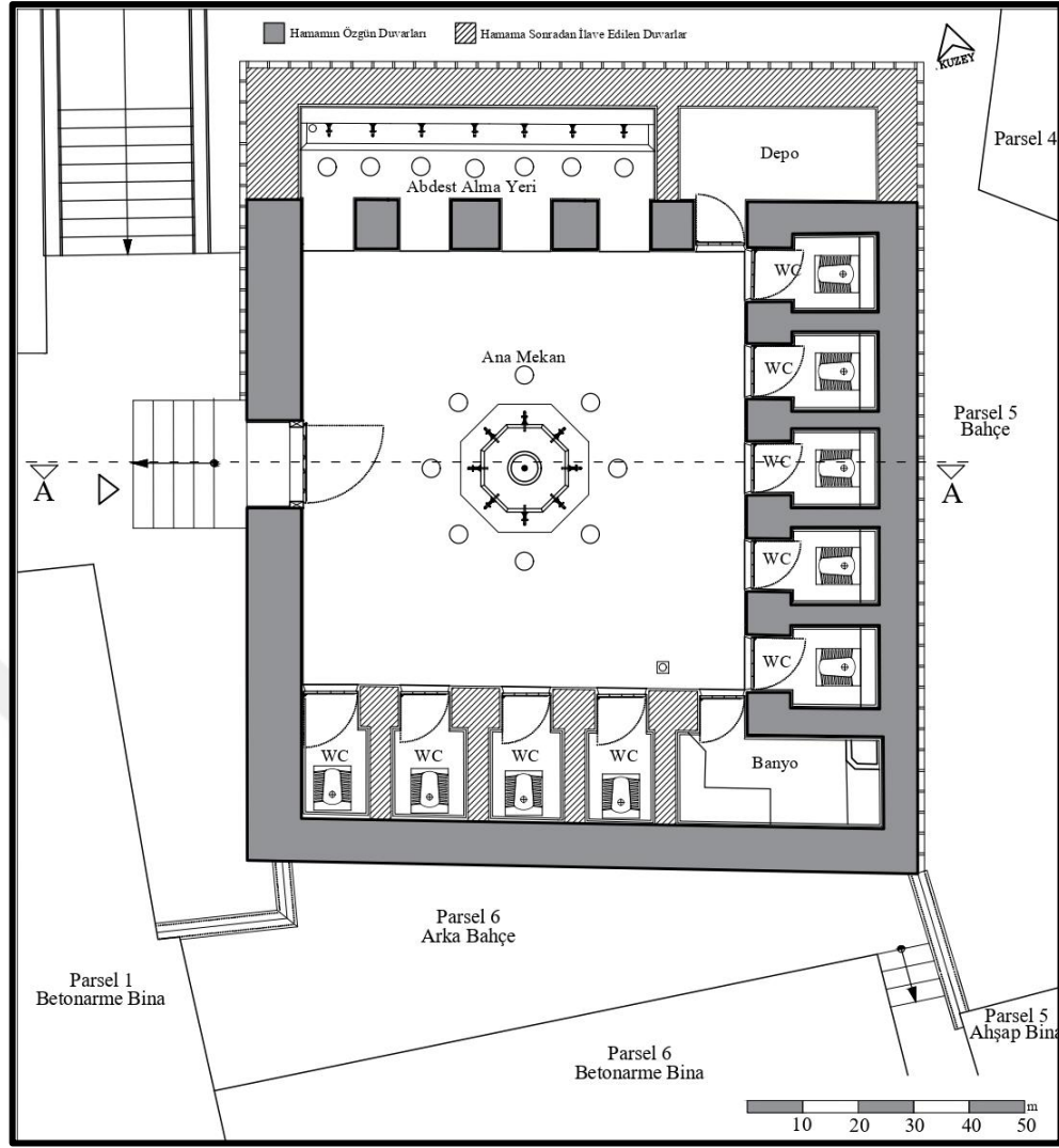
Şekil 3.69. Cık Cık Hamamı Restorasyon Planı (Asiltürk, Bursa Büyükşehir Belediyesi Arşivinden alınarak çizilmiştir.)
