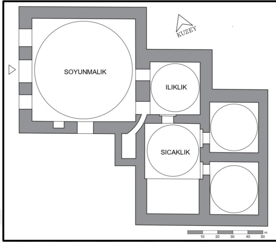
Şekil 3.53. Yıldırım Hamamı'nın Planı (Asiltürk, Şehitoğlu ve E. H. Ayverdi'den alınarak çizilmiştir.)
