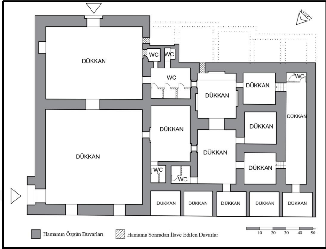
Şekil 3.104. Kayhan Hamamı Restorasyon Planı (Asiltürk, K.T.V.K.K. Arşivinden alınarak çizilmiştir.)
