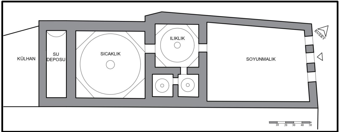
Şekil 3.96. İnebey Hamamı Restitüsyon Planı (Asiltürk, E. Şehitoğlu ve E. Ayverdi'den alınarak çizilmiştir.)
