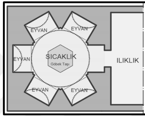
Şekil 2.16. Altıgen yıldızvari sıcaklıklı plan tipi (Eyice, 1997; Düzenleyen: Demir, 2019).
