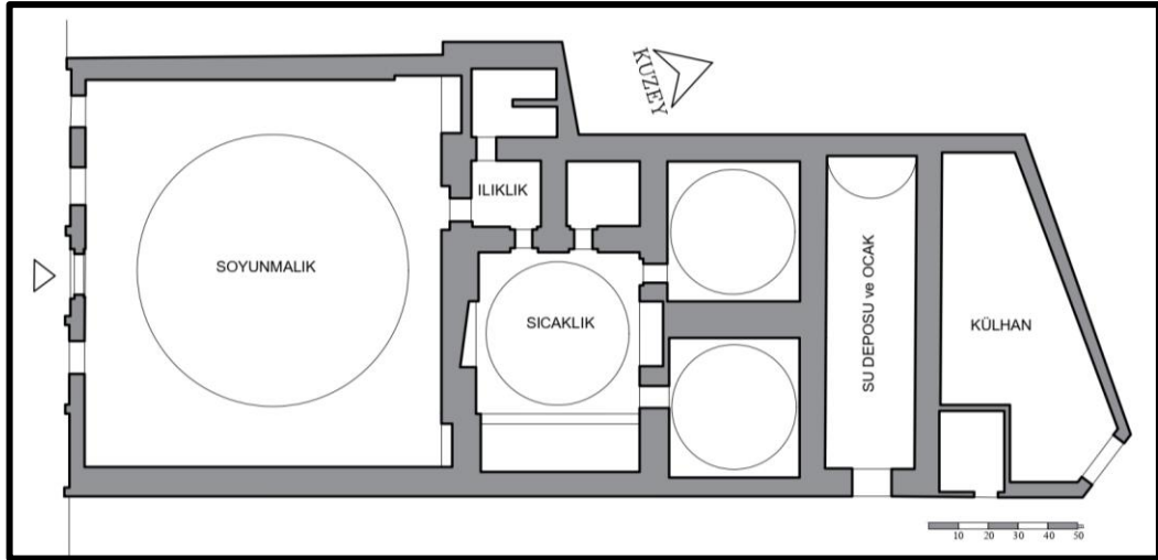
Şekil 3.181. Reyhanpaşa Hamamı Restitüsyon Planı (Asiltürk, E. Şehitoğlu ve E. Ayverdi'den alınarak çizilmiştir.)
