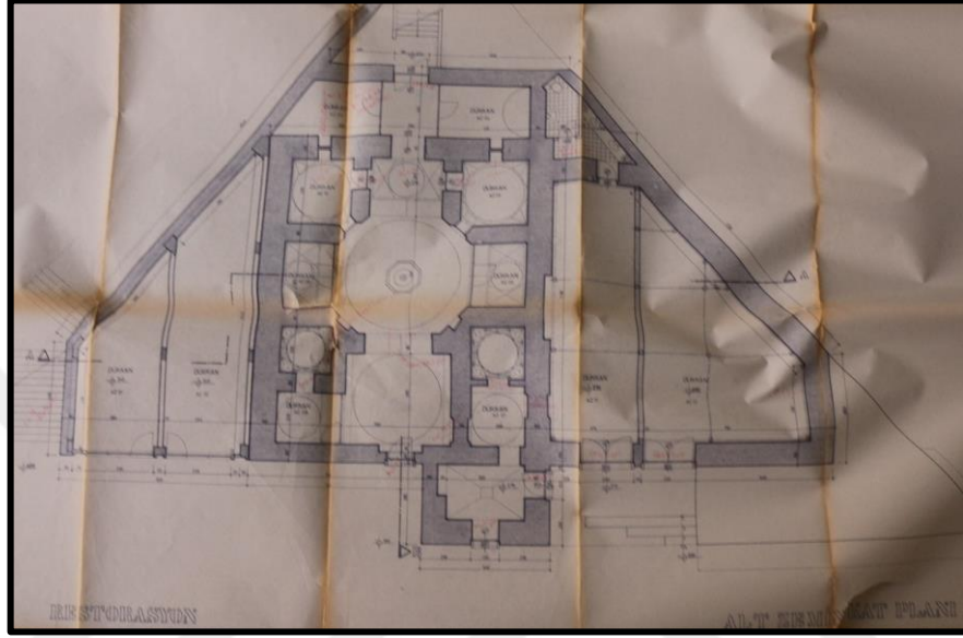
Şekil 3.168. Perşembe (Kadı) Hamamı'nın 1991 Yılında Çizilen Alt Kotunun Restorasyon Planı (K.T.V.K.K. Arşivi, 2023)
