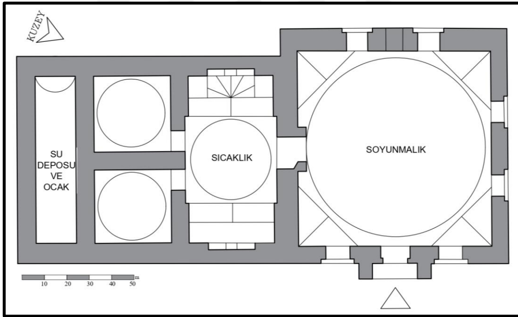
Şekil 3.132. Muradiye (II. Murad) Hamamı Planı (Şehitoğlu ve E. H. Ayverdi'den alınarak çizilmiştir.)
