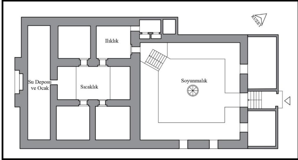
Şekil 3.204. Umurbey Hamamı Planı (Şehitoğlu ve A. Gabriel'den alınarak çizilmiştir.)
