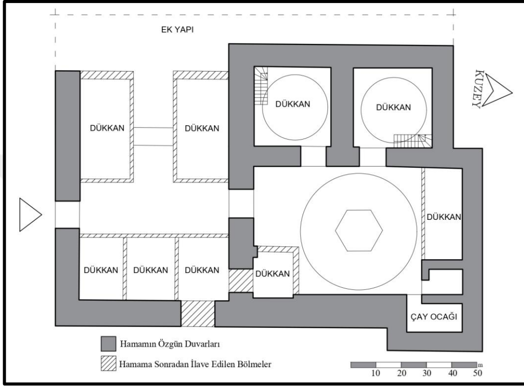
Şekil 3.188. Şengül Hamamı'nın Günümüzdeki Planı (Asiltürk, Alan çalışması ile çizilmiştir.)
