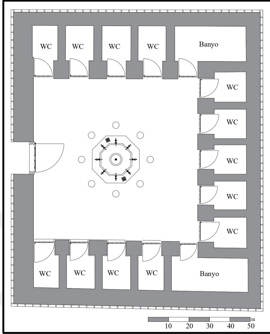
Şekil 3.65. Cık Cık Hamamı Restitüsyon Planı (Asiltürk, Bursa Büyükşehir Belediyesi Arşivi'nden alınarak çizilmiştir.)
