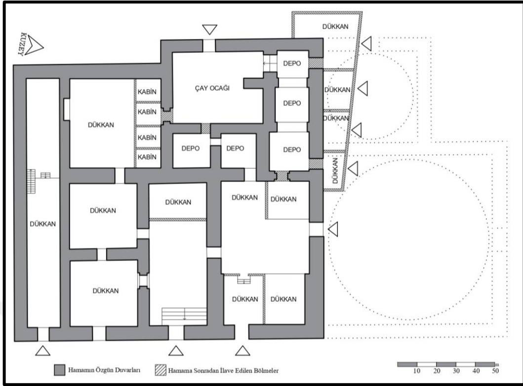
Şekil 3.194. Tavukpazarı (Meyhaneli) Hamamı'nın Günümüzdeki Planı (Asiltürk, Alan çalışması ile çizilmiştir.)
