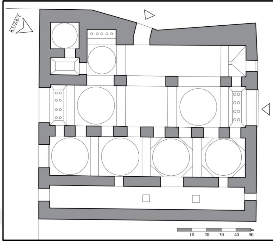
Şekil 3.125. Muallimzade Hamamı Restitüsyon Planı (Asiltürk, E. Şehitoğlu'ndan alınarak çizilmiştir.)
