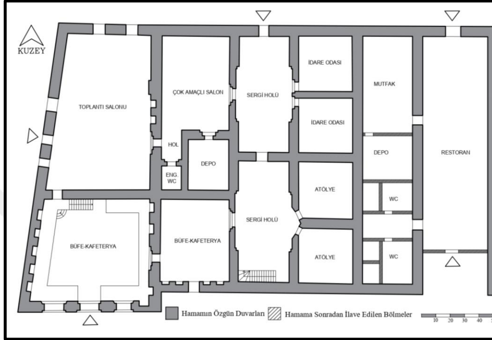
Şekil 3.162. Ördekli Hamamı Restorasyon Planı (Asiltürk, Bursa Büyükşehir Belediyesi arşivinden alınarak çizilmiştir.)
