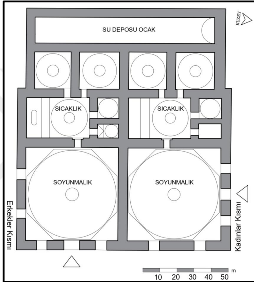
Şekil 3.11. Dayıoğlu Hamamı Planı (Şehitoğlu ve E. H. Ayverdi'den alınarak çizilmiştir.)
