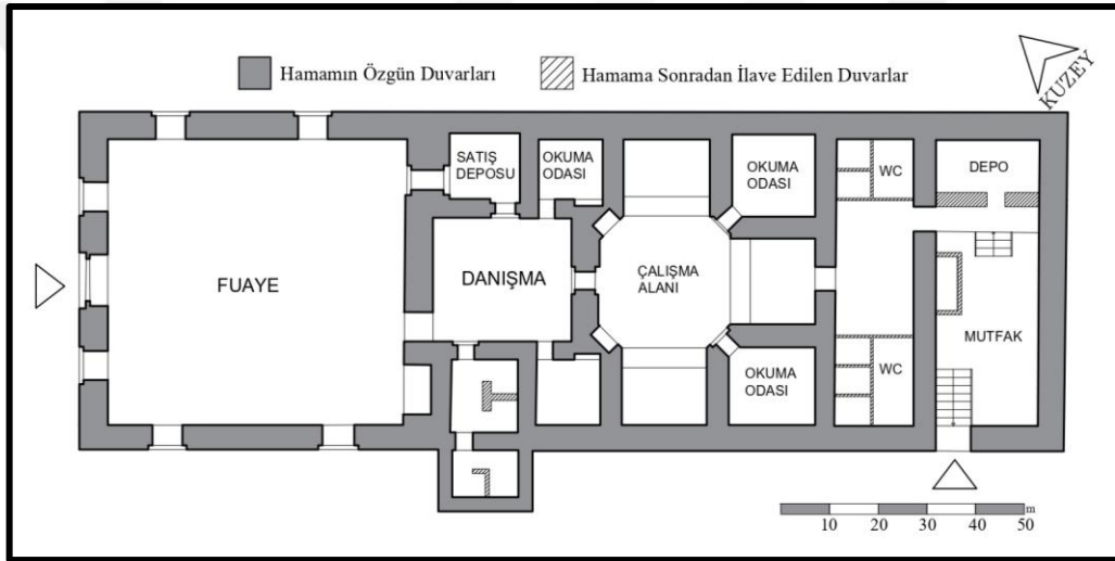
Şekil 3.76. Emir Sultan Hamamı Restorasyon Planı, 2006 (Asiltürk, K.T.V.K.K. Arşivinden alınarak çizilmiştir.)
