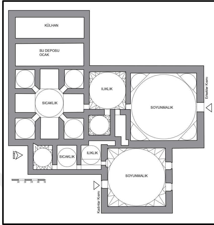
Şekil 3.153. Orhan Gazi Hamamı Planı (Asiltürk, Şehitoğlu ve E. H. Ayverdi'den alınarak çizilmiştir.)
