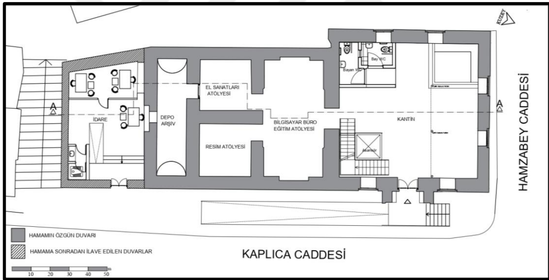
Şekil 3.133. Muradiye Hamamı Restorasyon Projesi Kat Planı (Bursa Büyükşehir Belediyesi Arşivinden alınarak çizilmiştir.)
