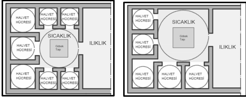
Şekil 2.17. Kare sıcaklık etrafında üç sıra sıralanan halvet hücreli plan tipi (Eyice, 1997; Düzenleyen: Demir, 2019).
