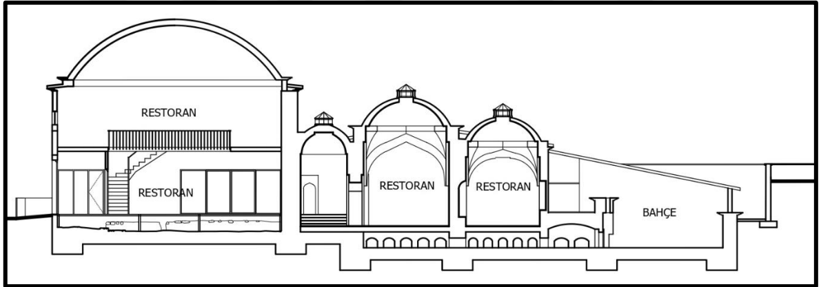
Şekil 3.112. Kiremitçi Sinan Bey Hamamı A-A Kesiti (Asiltürk, Bursa Büyükşehir Belediyesi Arşivinde alınarak çizilmiştir.)
