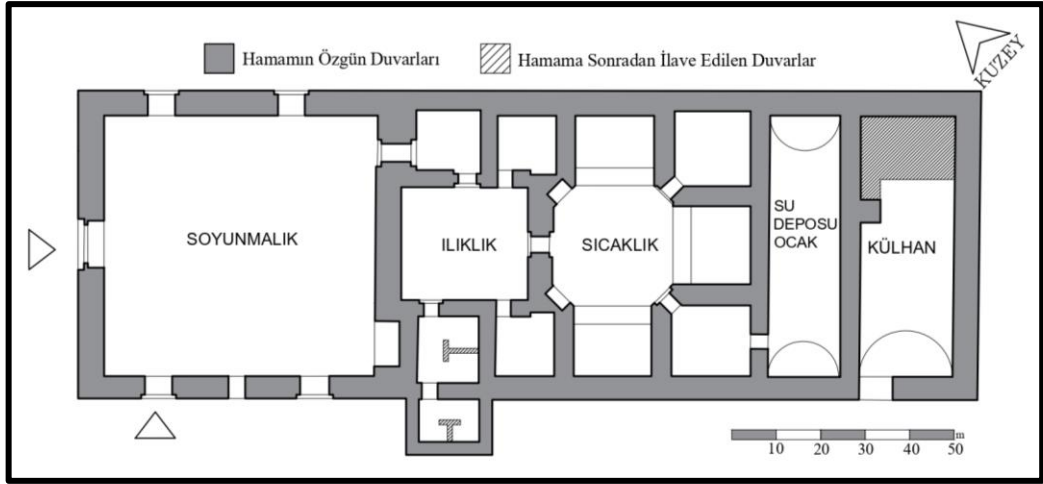
Şekil 3.75. Emir Sultan Hamamı Rölöve Planı (Asiltürk, K.T.V.K.K. Arşivinden alınarak çizilmiştir.)
