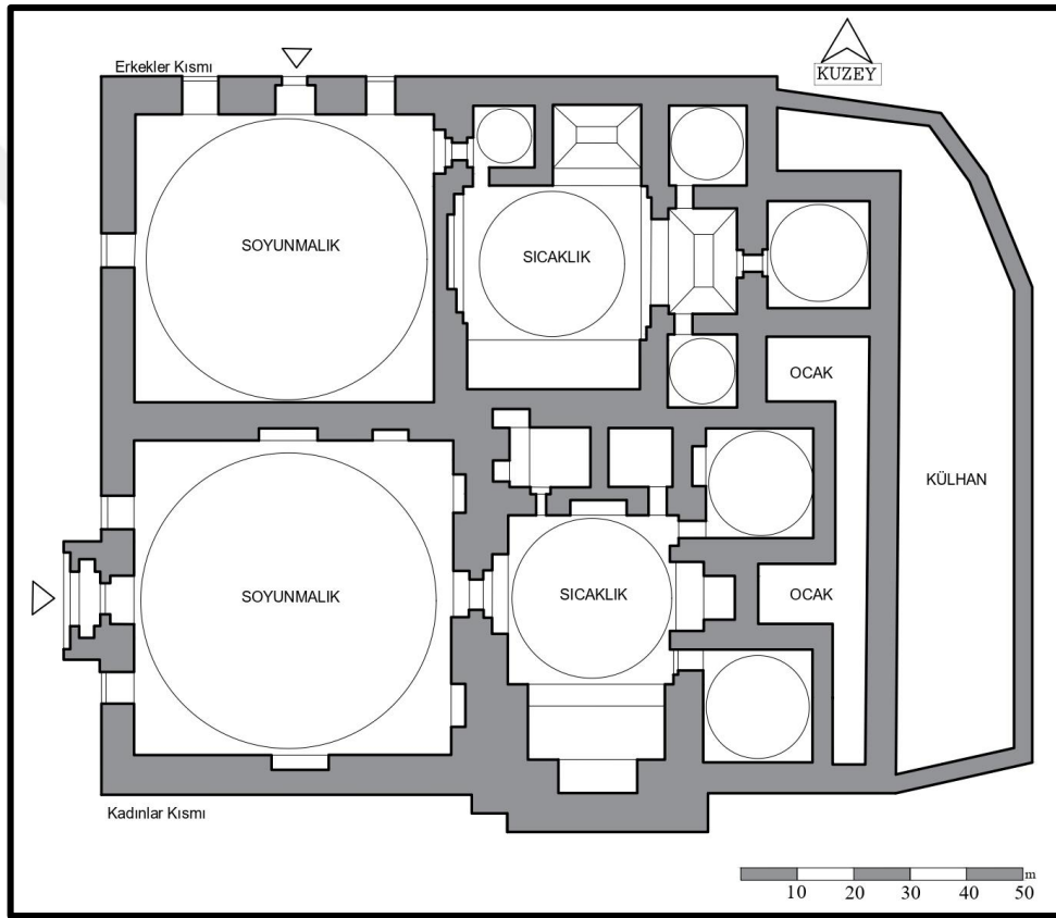
Şekil 3.117. Mahkeme (İbrahimpasha) Hamamı Restitüsyon Planı (Asiltürk, E. Şchitoğlu ve E. H. Ayverdi'den alınarak çizilmiştir.)
