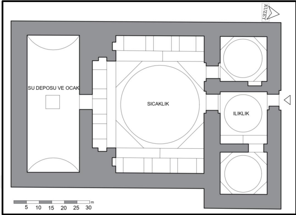
Şekil 3.26. Hanzade (Hançerli Sultan) Hamamı Planı (Asiltürk, Şehitoğlu'ndan alınarak çizilmiştir.)
