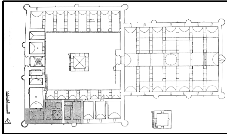
Şekil 2.5. Tuzhisar Sultan Han Planı ve Han İçerisindeki Hamam (Tükel Yavuz, 2012)
