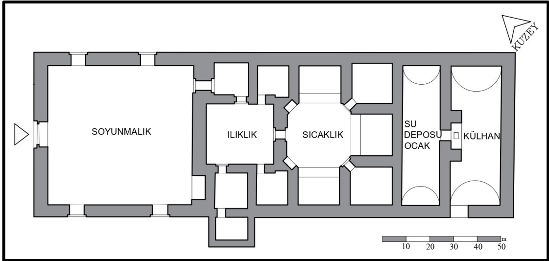
Şekil 3.74. Emir Sultan Hamamı Restitüsyon Planı (Asiltürk, Şehitoğlu ve E. H. Ayverdi'den alınarak çizilmiştir.)
