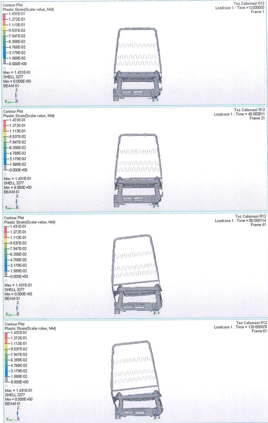
Şekil 6.22. R12' ye göre farklı zamanlarda koltuk üzerinde plastik zorlanma-önden görünüş
