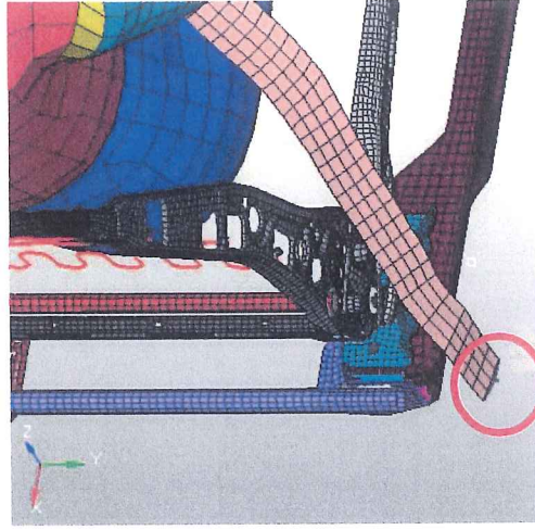
Şekil 6.28. Spring 2 Emniyet kemer bağlantı noktası
