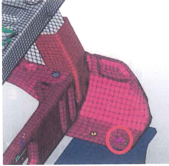
Şekil 6.37. Sol ön zemin bağlantı noktası (Spring 58336)
