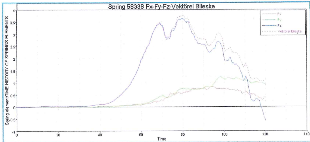
Şekil 6.40. Sol arka zemin bağlantı yayı (öndeki)
