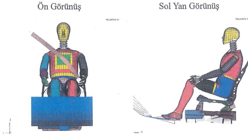
Şekil 6.2. Koltuğa Ait Sonlu Elemanlar Modelinin Farklı Açılardan Gösterimi
