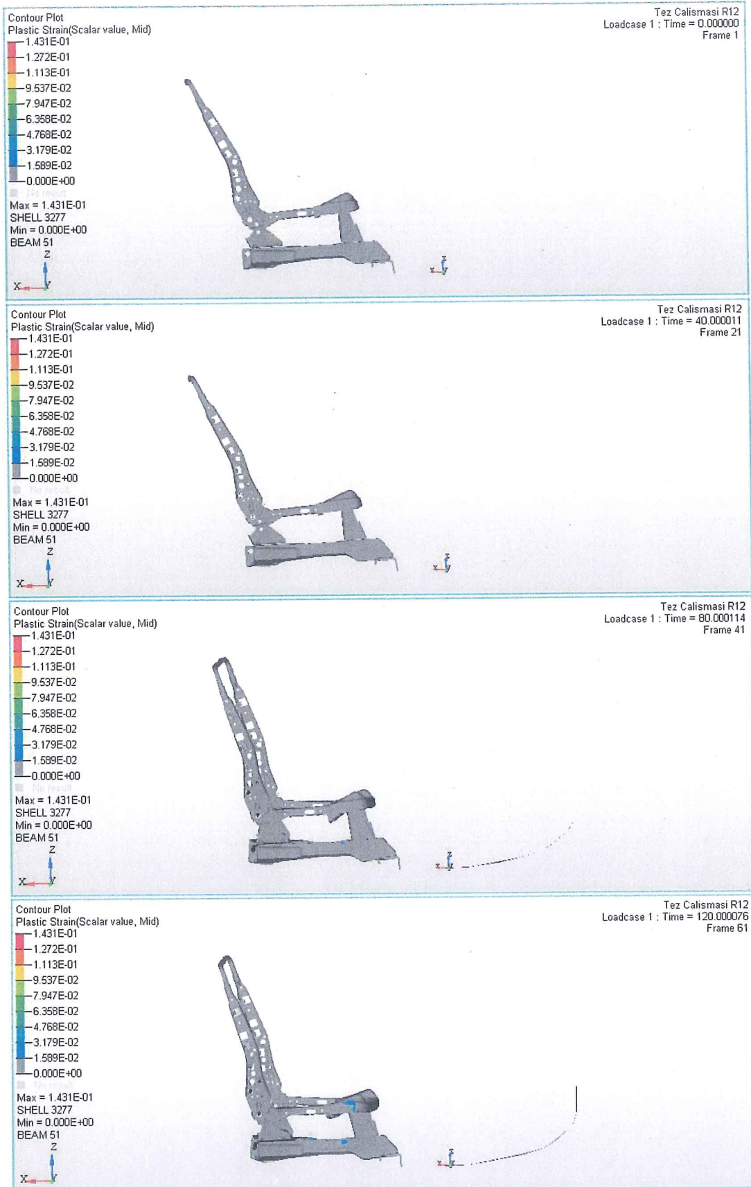
Şekil 6.21. R12' ye göre farklı zamanlarda koltuk üzerinde plastik zorlanma-sağ yan görüntüş
