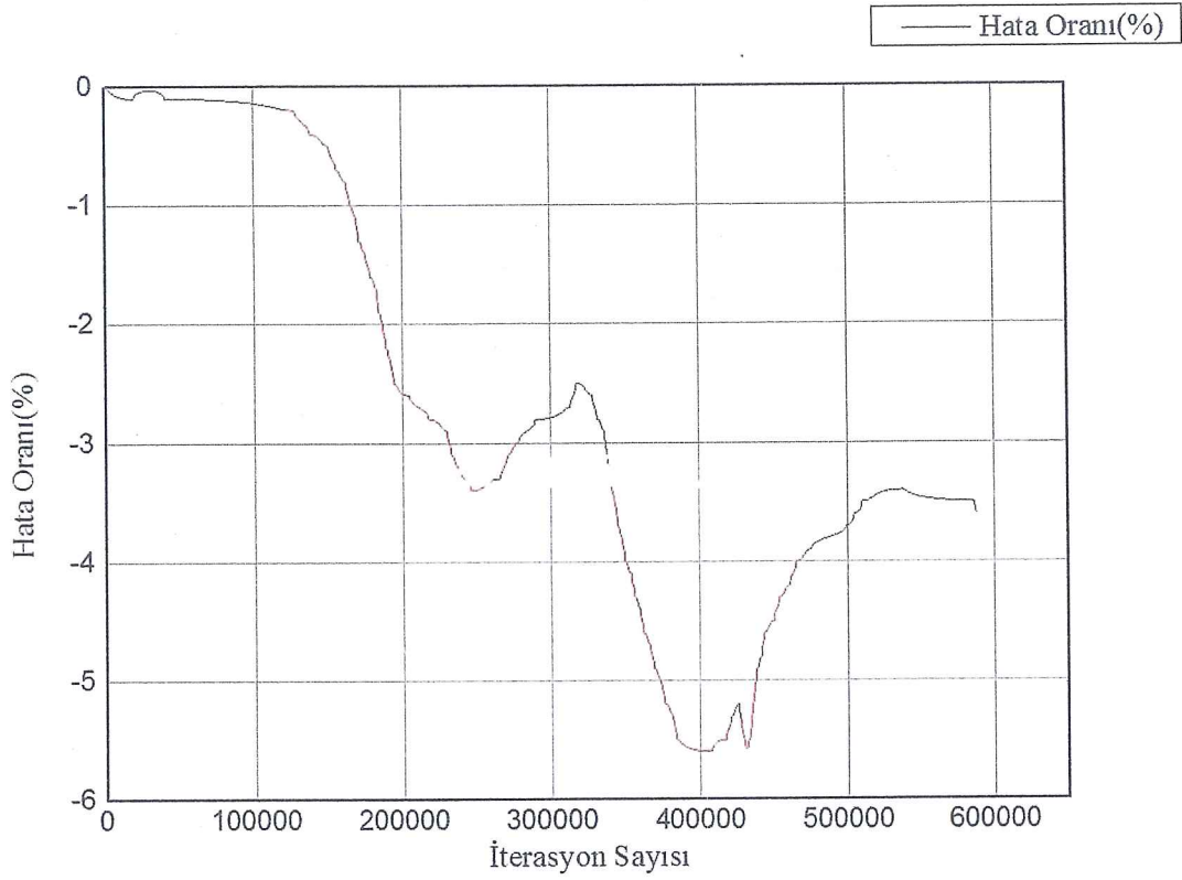
Şekil 6.10. Convergence(yakınsama) Grafiği
