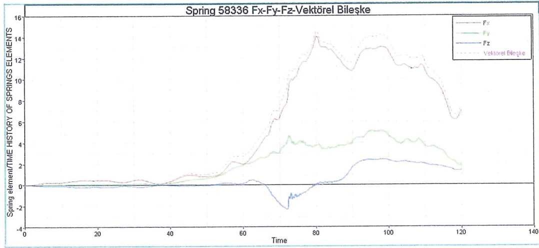
Şekil 6.38. Sol ön zemin bağlantı yayı
