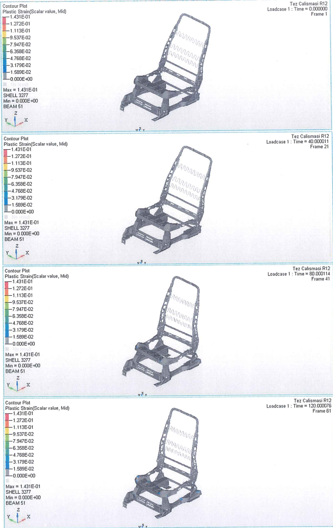
Şekil 6.24. R12' ye göre farklı zamanlarda koltuk üzerinde plastik zorlanma-önden perspektif görünüş
