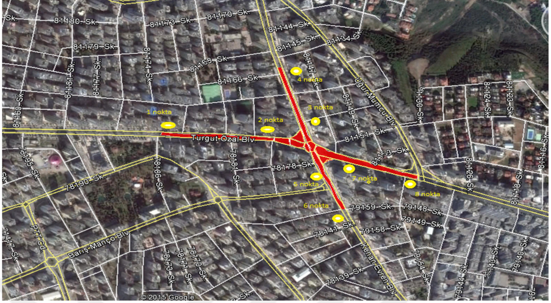
Şekil 4.1. Turgut Özal Bulvarı ve Kenan Evren Bulvarı kesişim kavşağı çevresel gürültü ölçüm noktaları.
