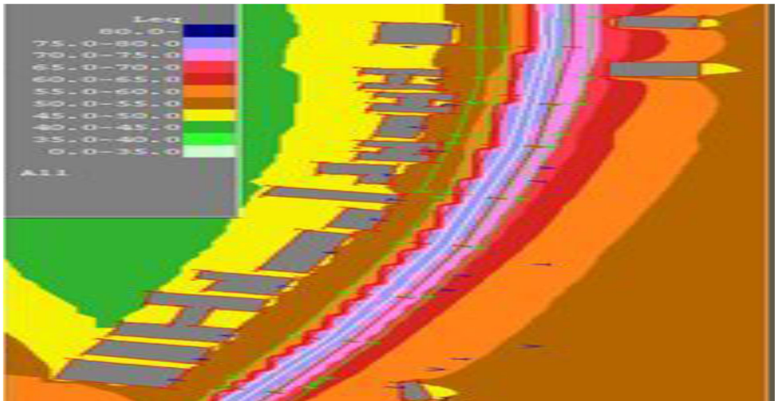
Şekil 2.3. Raylı sisteme ait akustik modelleme (URL-5).
