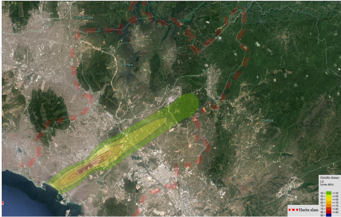
Şekil 2.4. Sabiha Gökçen Hava Meydanı ve 2012'de kalkış L_{den} yüksek ses noktaları.
