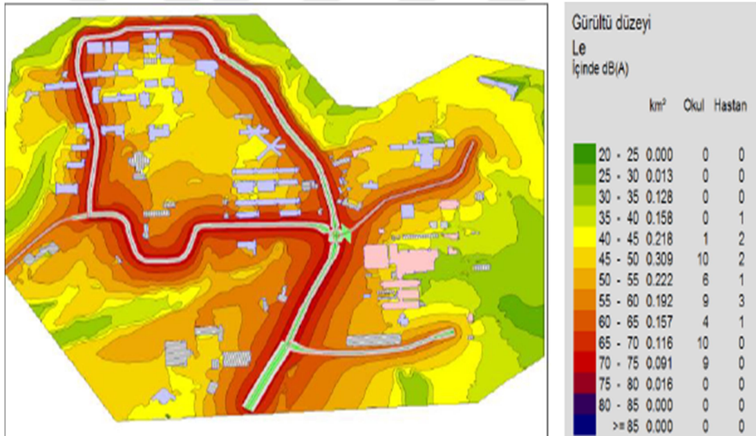
Şekil 2.11. Çukurova Üniversitesi Kampüsü L akşam ızgaralı gürültü haritası (Bıçakçı vd., 2011).
