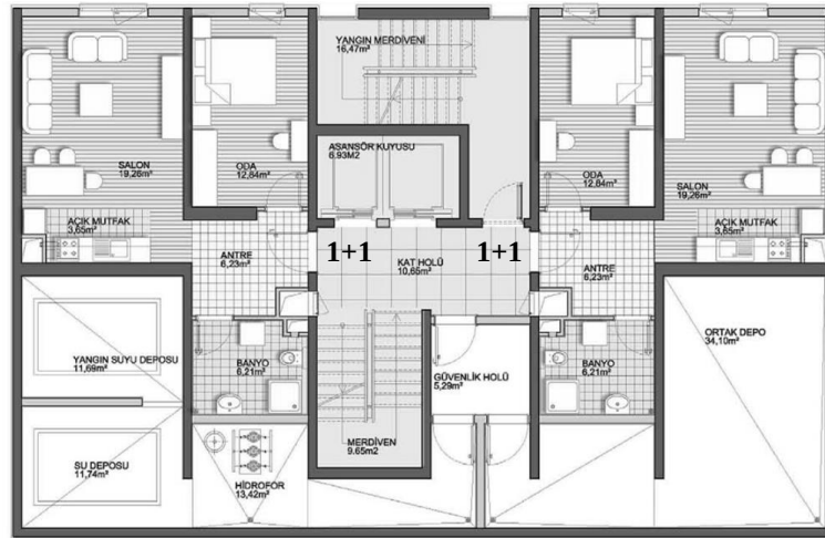
Figure 2.12. B1 Block Floor Plan 1+1 Apartments (TOKİ Kayabaşı Yerleşimi 879-1 ve 876-3 Ada Toplu Konut Projesi, n.d.)
