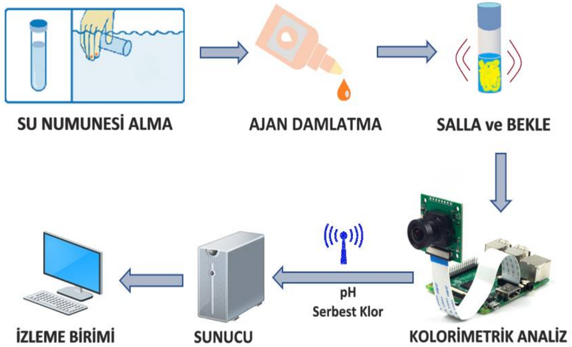
Şekil 3.1 Sistemin blok şeması.
