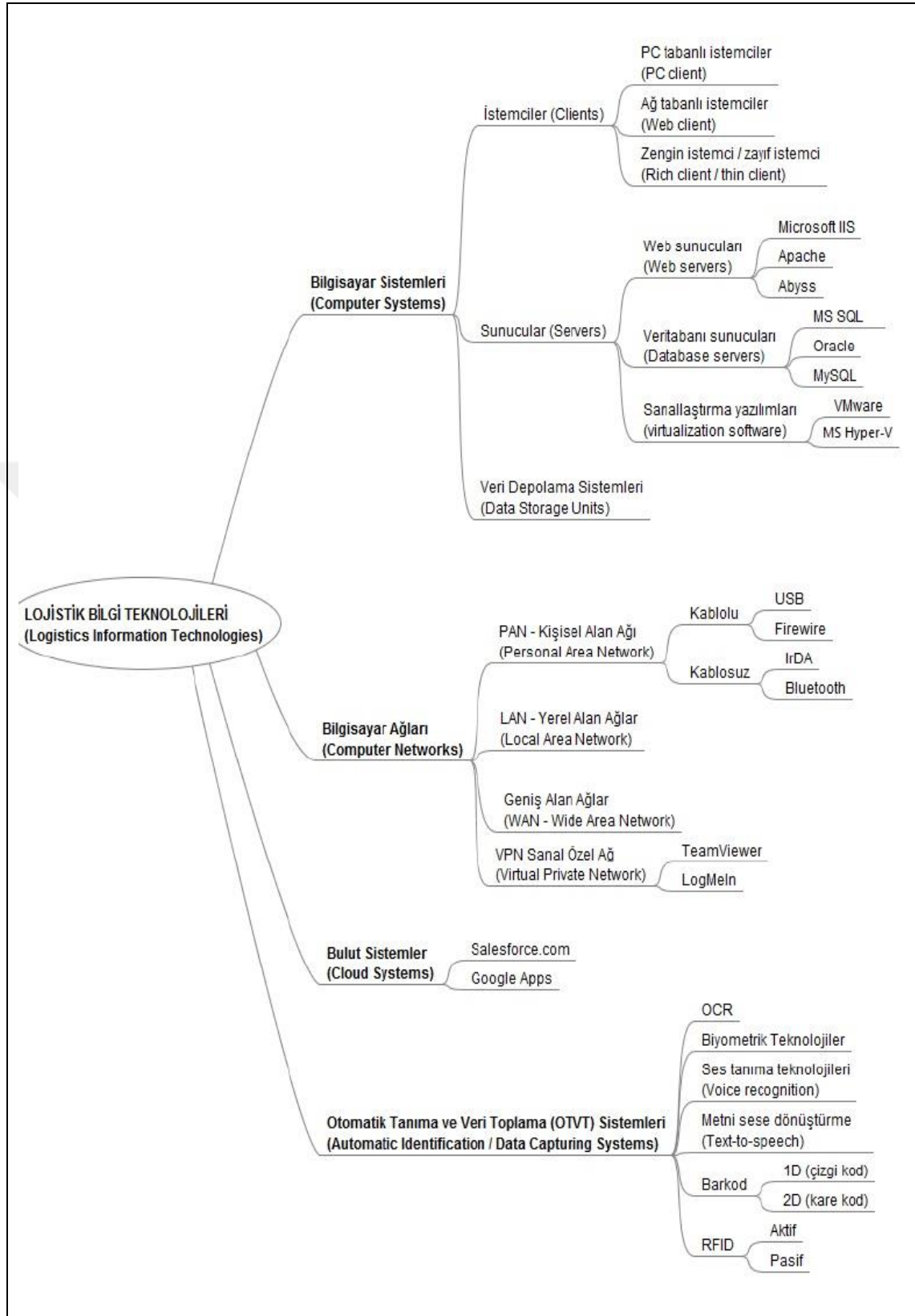
Şekil 6.Lojistik Bilgi Teknolojileri
