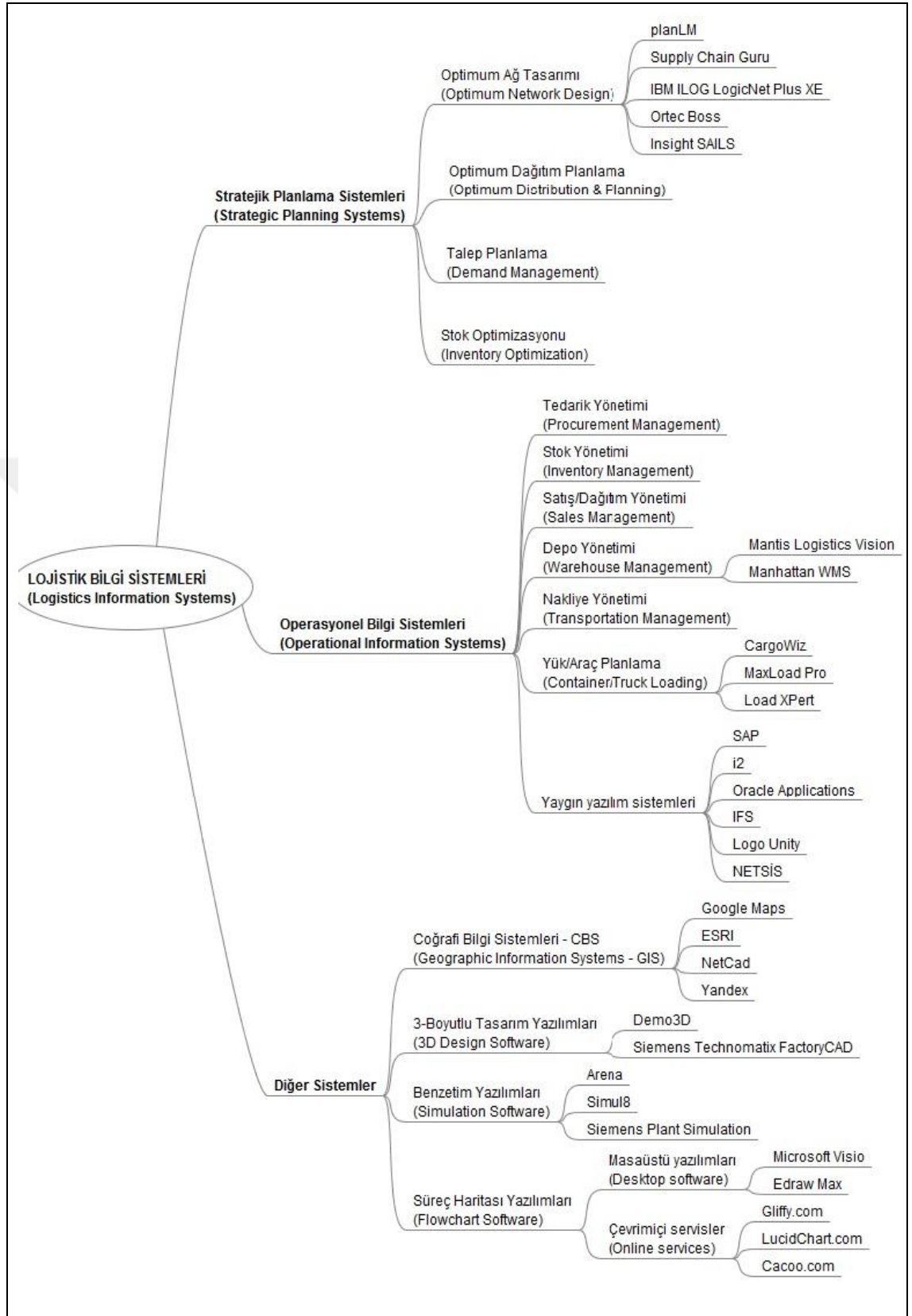
Şekil 4.Lojistik Bilgi Sistemleri
