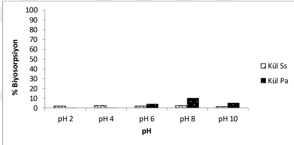
Şekil 4.12. Kül algler ile RBB'nin biyosorpsiyonunda pH etkisi.
