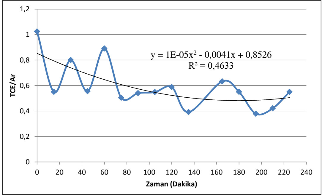
Şekil 4.5b (Yıkanmış, Karbonize) + (Yıkanmış, Taranmış) boyalı yün lifi numunesi-2 için sorpsiyon grafiği
