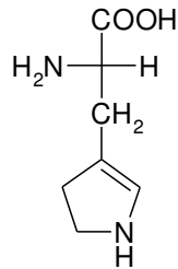
B- [İndolil-(3)]-alanin L (-) Triptofan (Try)
