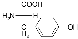
β-(4-hidroksi-fenil)-alanin L(-)-Tirozin (Try)
