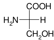
\alpha -Amino- \beta -hidroksi-propionik asit L (-) Serin (Ser)
