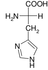
\beta ,[İmidazoli-(4)]-alanin L (-) Histidin (His)
