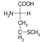
α-Amino-γ-metilmerkpto- bütürük asit L (-) Metionin (Met)
