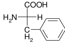
\alpha -Amino- \beta fenil-propionik asit L (-) Fenilalanin (Phe)
