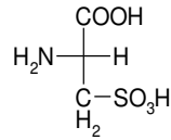
α-Amino-β-sülfonik asit- propiyonik asit L (-) Sistein asidi (CySO 3 H)
