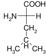
\alpha -Amino-isokaproik asit L (-) Loysin (Leu)
