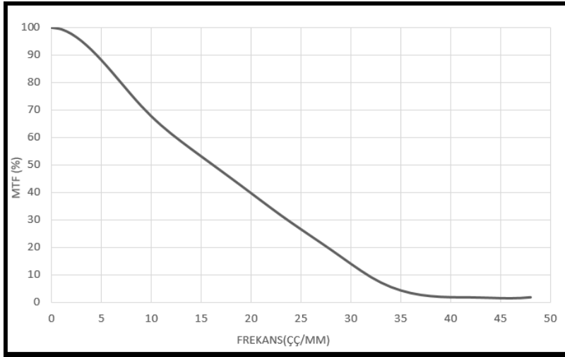
Şekil 3.8. Örnek Modülasyon Transfer Fonksiyonu (MTF) Grafiği
