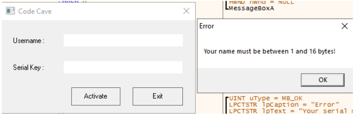
Şekil 6.44. Hata mesajı
