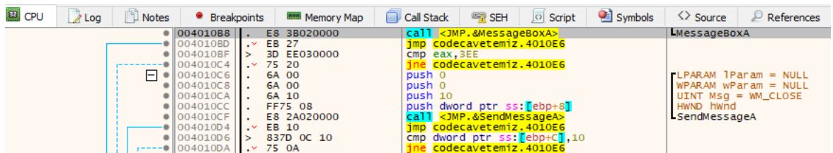
Şekil 6.43. MessageBoxA fonksiyonu
