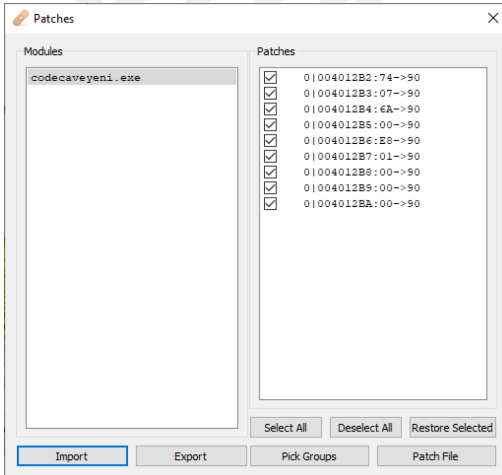
Şekil 6.40. Patch Penceresi
