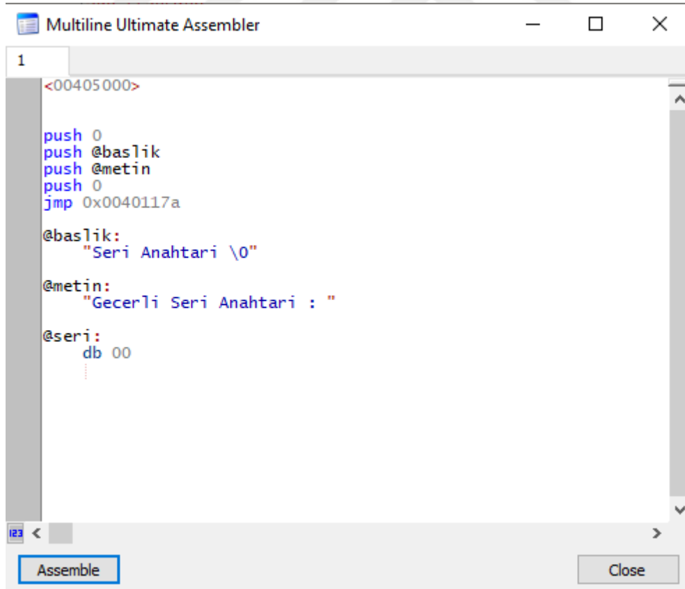
Şekil 6.59. Parametreler
