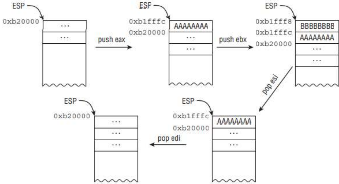
Şekil 2.4. Yığın kullanımı
