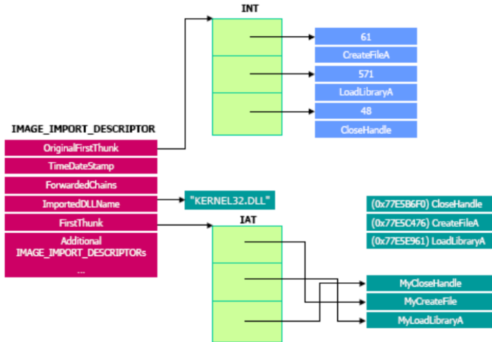
Şekil 3.8. IMAGE_IMPORT_DESCRIPTOR yapısı
