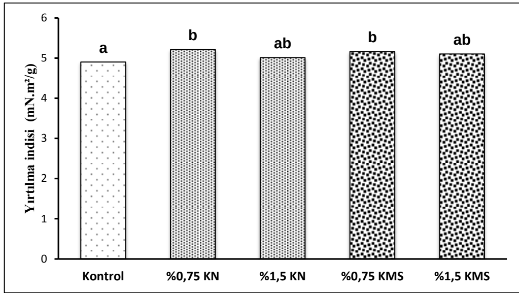
Şekil 55: 100 g/m 2 ’lik deneme kağıtlarına katılan KN ve KMS’nin yırtılma indisi üzerine etkileri.
