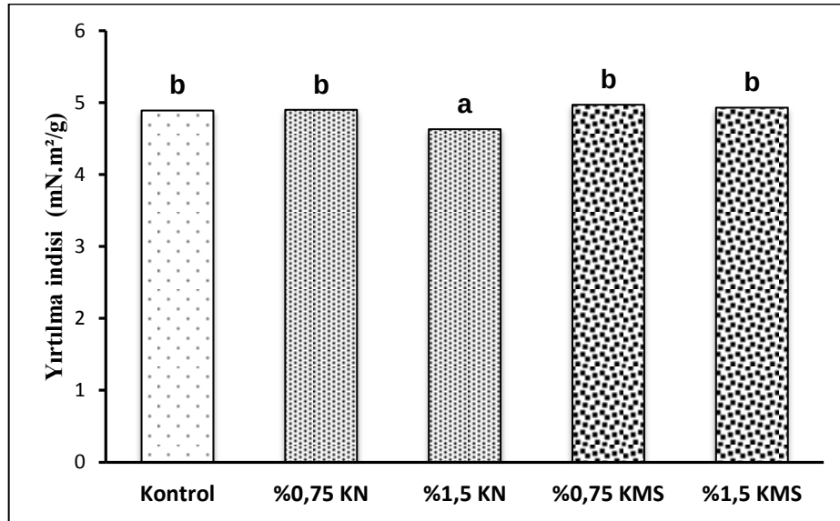
Şekil 52: 85 g/m 2 'lik deneme kağıtlarına katılan KN ve KMS'nin yırtılma indisi üzerine etkileri.
