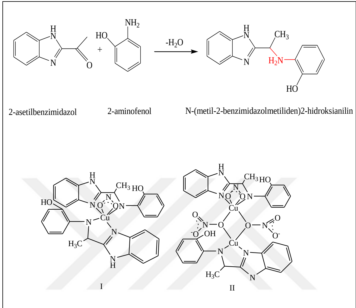
Şekil 2.2. N-(metil-2-benzimidazolmetiliden)-2-hidroksianalin ligantı ve onun Cu(II) Kompleksleri (I. Kompleks Mononükleer, II. Kompleks Binükleer)
