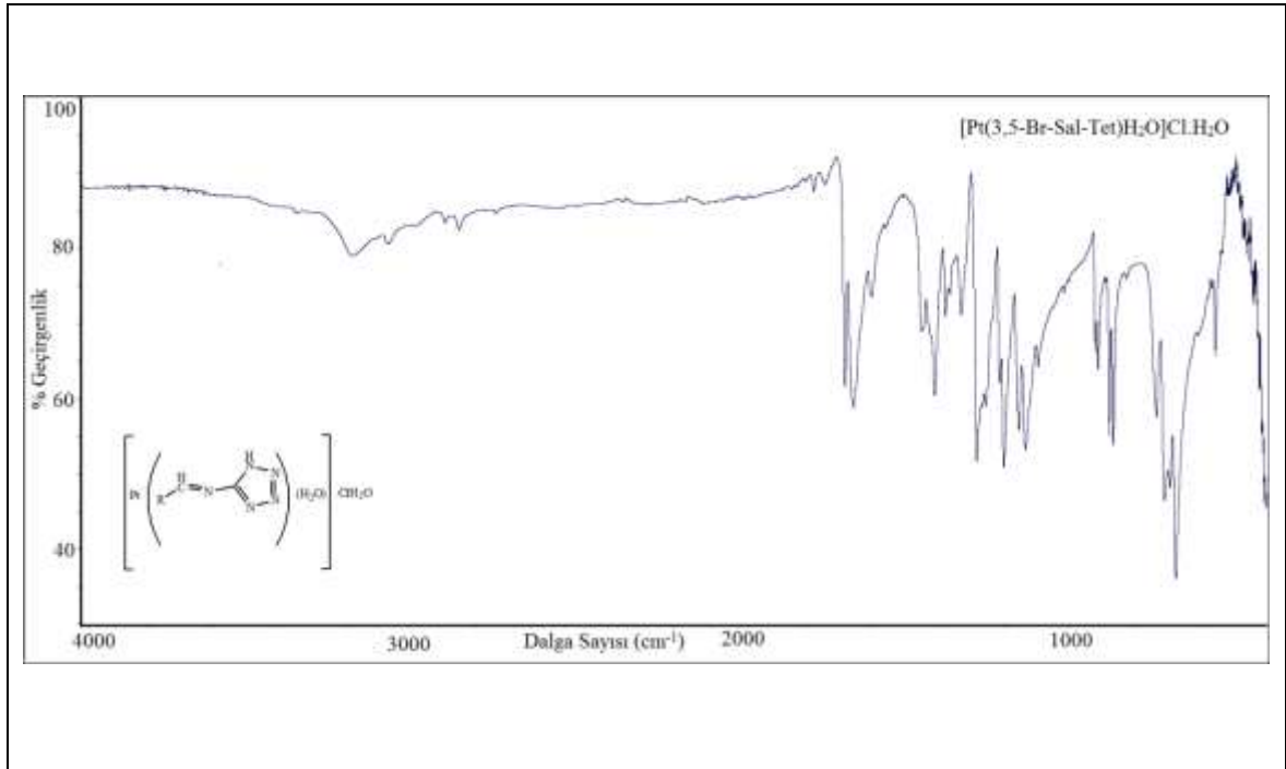
Şekil 5.14. [Pt(3,5-Br-Sal-Tet)H_2O]Cl.H_2O kompleksine ait FT-IR spektrumu
