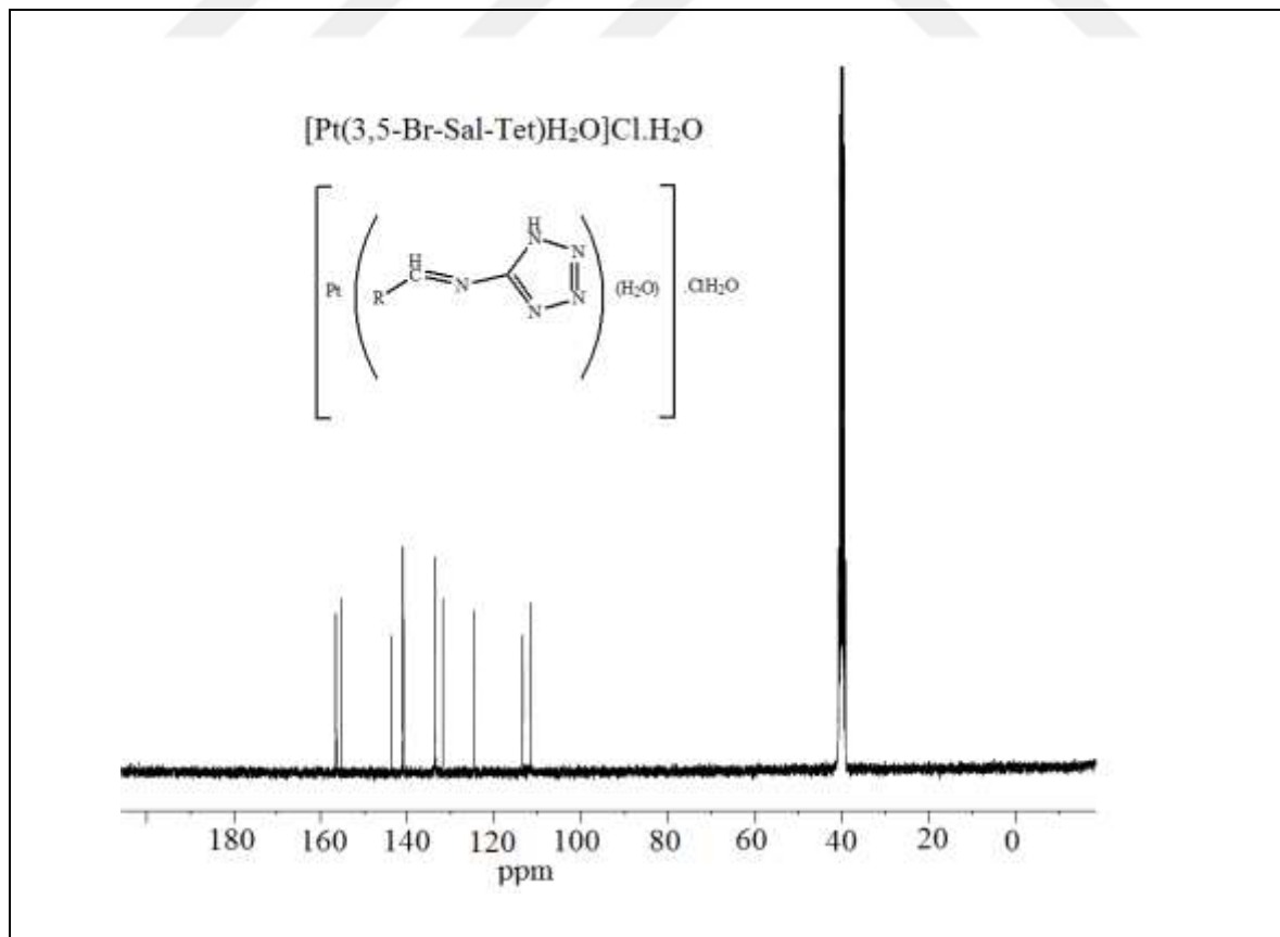
Şekil 5.16. [\text{Pt}(3,5\text{-Br-Sal-Tet})\text{H}_2\text{O}]\text{Cl}\cdot\text{H}_2\text{O} kompleksine ait ^{13}\text{C} -NMR Spektrumu
