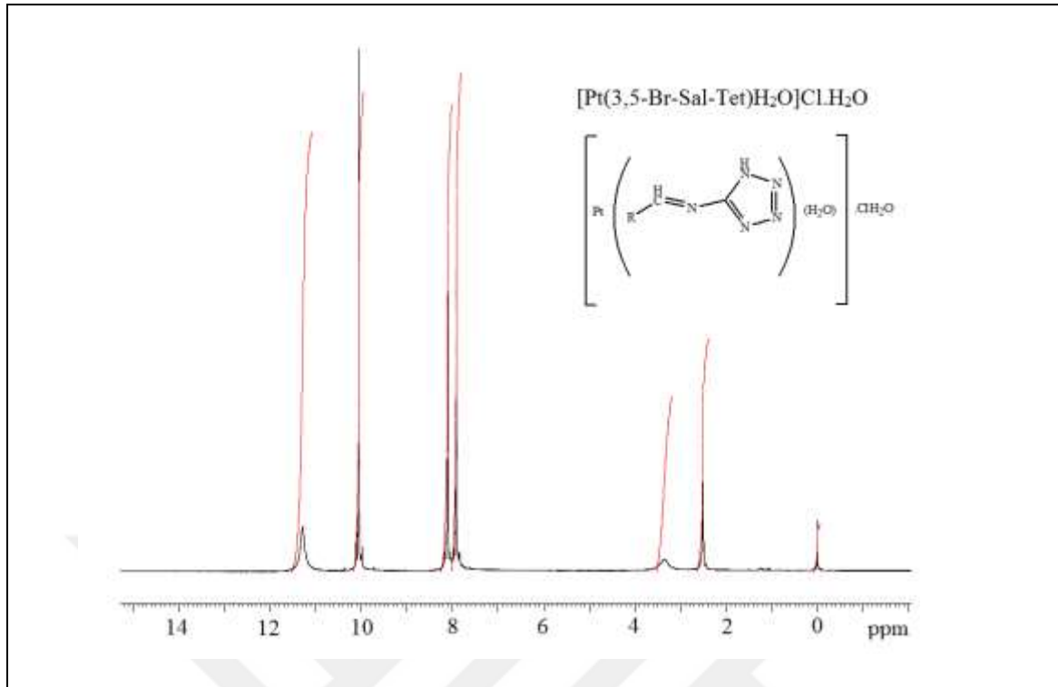
Şekil 5.15. [\text{Pt}(3,5\text{-Br-Sal-Tet})\text{H}_2\text{O}]\text{Cl}\cdot\text{H}_2\text{O} kompleksine ait ^1\text{H} -NMR Spektrumu
