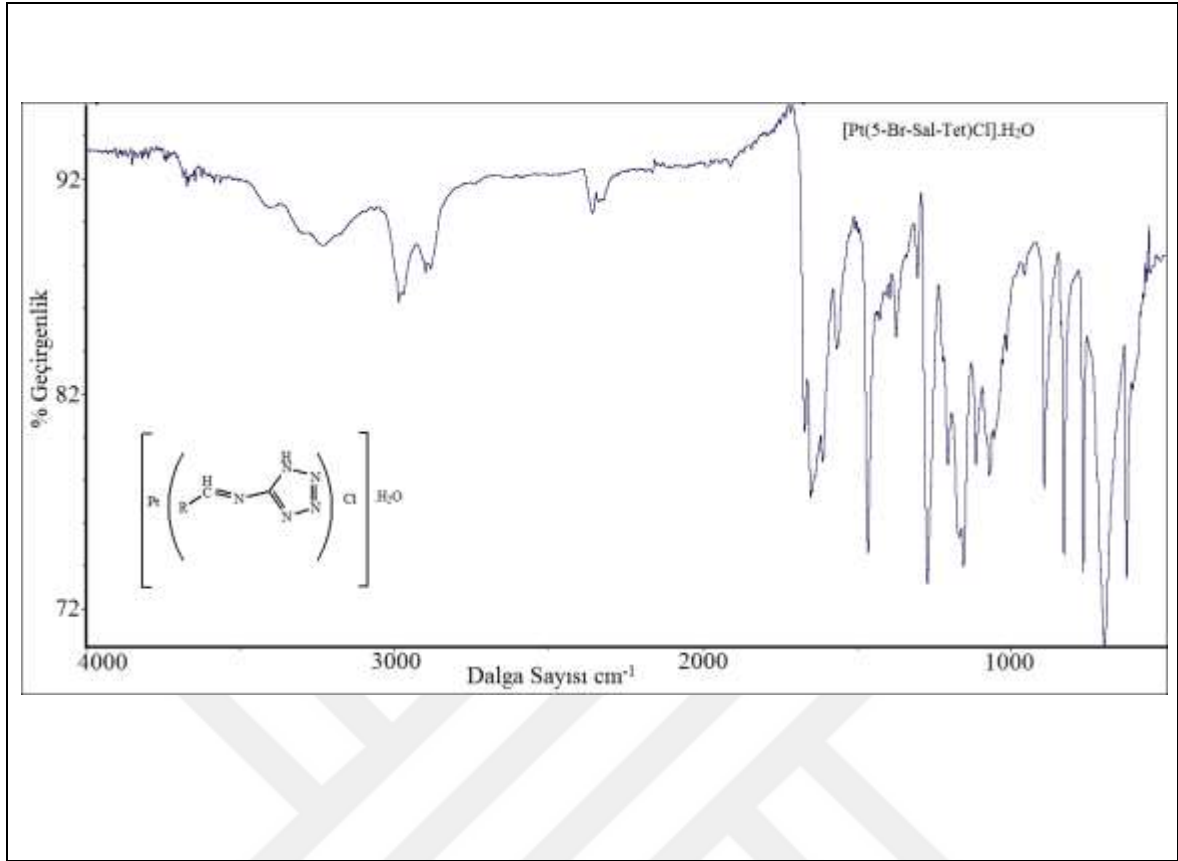
Şekil 5.13. [Pt(5-Br-Sal-Tet)Cl].H_2O kompleksine ait FT-IR spektrumu
