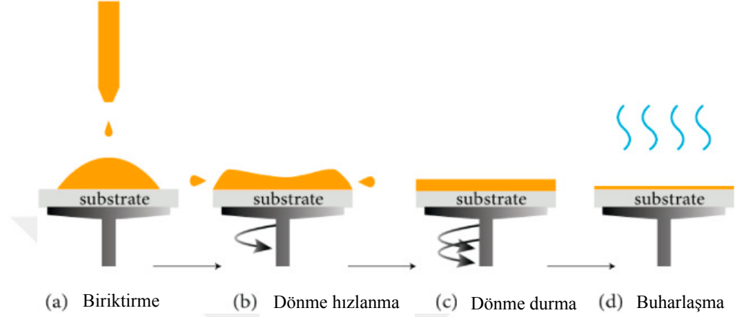
Şekil 2.10. Spin-kaplamanın dört temel aşaması: (a) Biriktirme, (b) Dönme hızlanma, (c) Dönme durma ve (d) Buharlaşma (Chtouki ve ark., 2021)
