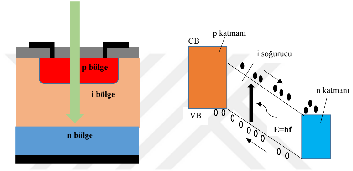
Şekil 2.5. PIN fotodiyotunun şematik çizimleri
