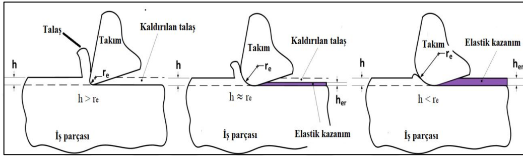
Şekil 2.7 Radyüslü takım ile kesme işleminde malzemede meydana gelen kazınma ve elastik deformasyon (Ding et al. 2011).
