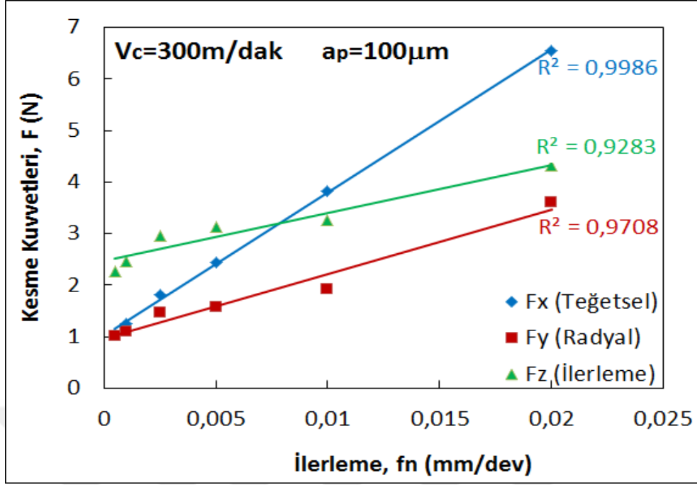
Şekil 4.3 V_C=300 m/dak, a_p=100 \mu m için F_x , F_y ve F_z düzleminde ölçülen kesme kuvvetleri.
