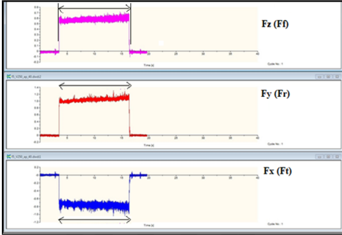
Şekil 3.4 Ölçülen kuvvetlerin ortalama değerinin elde edilmesi.
