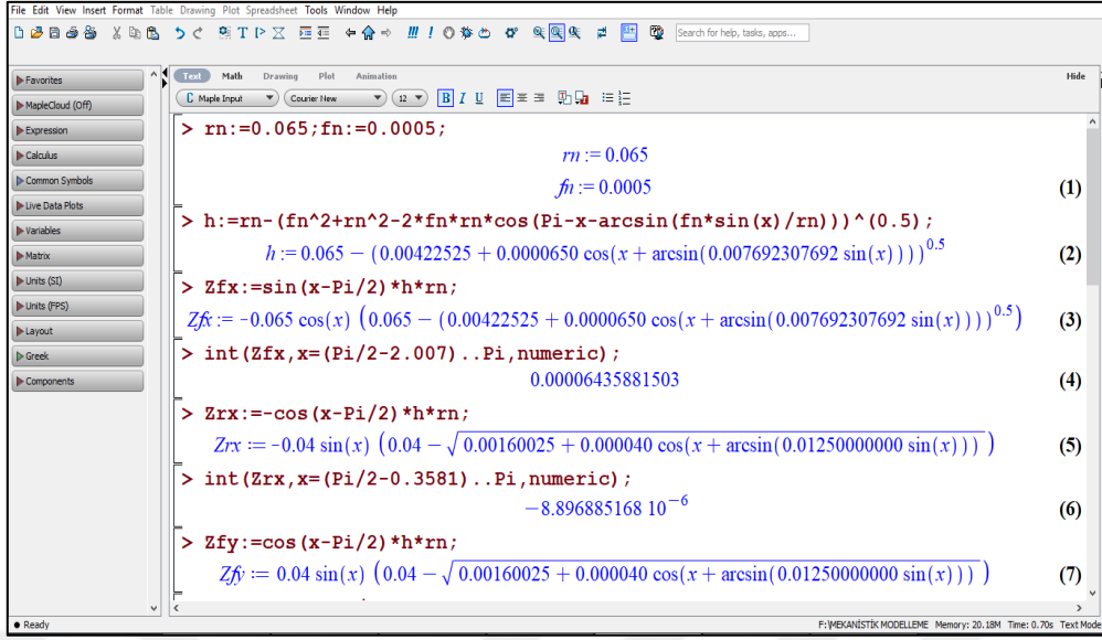
Şekil 3.9 Mapple programı yardımıyla G ve Z katsayılarının hesaplanması.
