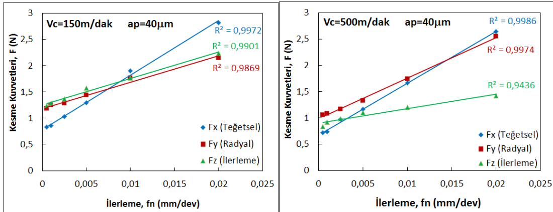
Şekil 4.4 V_C=150 ve 500 m/dak için farklı ilerleme değerlerine bağlı olarak kesme kuvvetlerinin değişimi.
