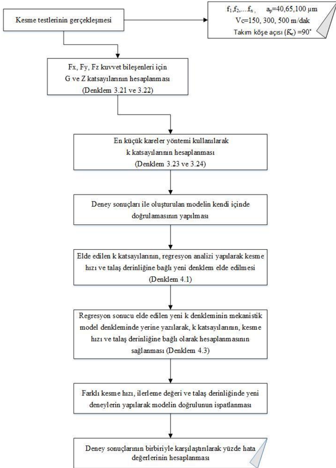
Şekil 3.5 Mekanistik modellemenin oluşturulmasında izlenilen yöntem.
