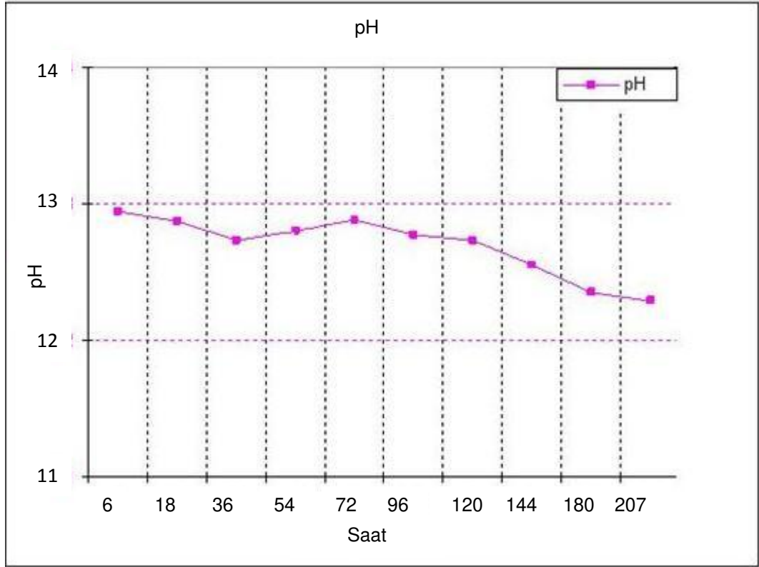
Şekil 5.5 Katkısız \text{TiO}_2 ile yapılan parçalanma deneyine ait pH değişimi
