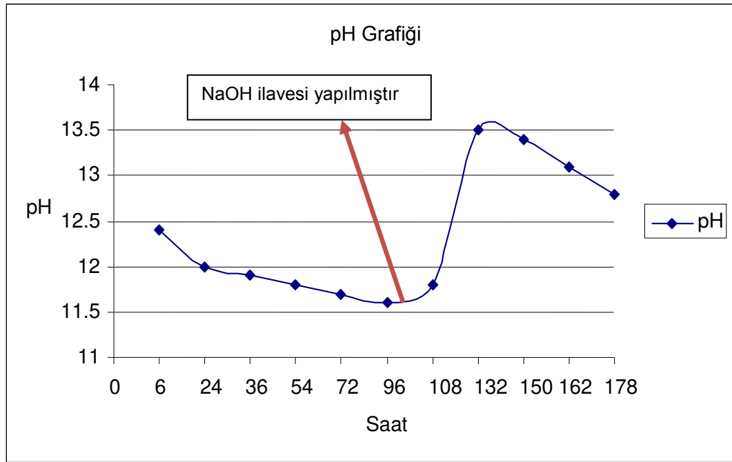
Şekil 5.7 V – \text{TiO}_2 ile yapılan parçalanma deneyine ait pH değişimi
