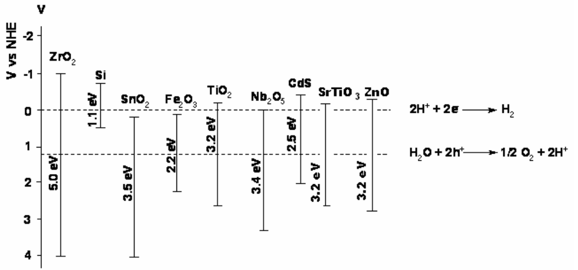
Şekil 2.5 Bazı yarı iletkenlere ait band enerji seviyeleri (Sayılkan, 2007)
