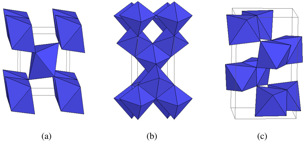
Şekil 2.6 \text{TiO}_2 yarı iletkenine ait kristal formları: (a) rutil, (b) anataz ve (c) brookit (Özyıldız, 2006)
