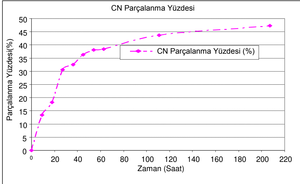
Şekil 5.4 Katkısız \text{TiO}_2 kaplama ile yapılan parçalanma deneyine ait CN parçalanma yüzdesi
