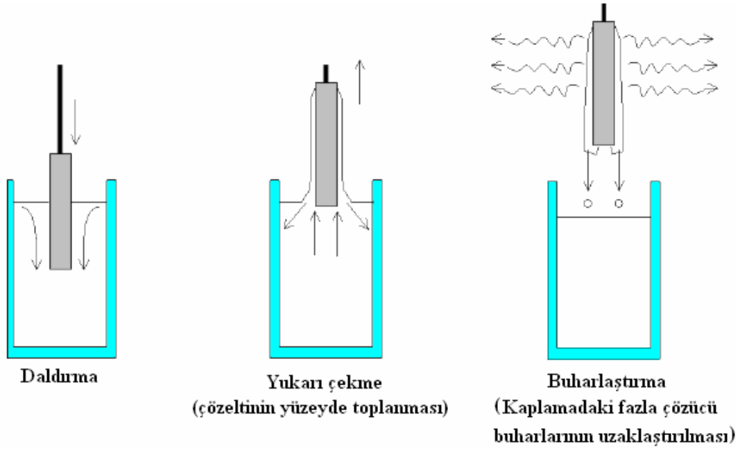
Şekil 2.10 Daldırma Kaplama Tekniğinin şematik gösterimi (Sayılkan, 2007)
