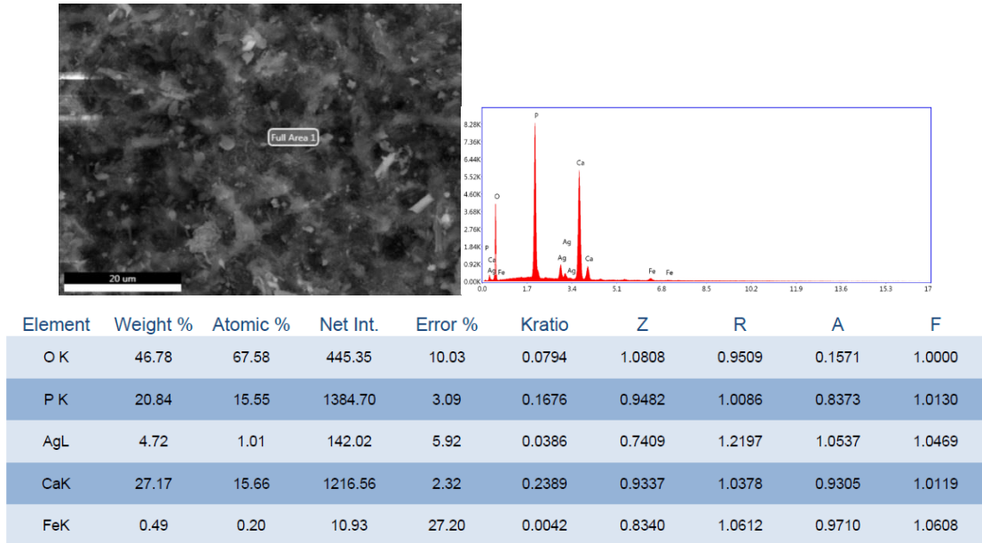
Şekil 6.34. HAP-k ile kumlanmamış Titanyum plaka üzerine 3 mm mesafeden yapılan kaplama sonrası alınan EDX analizi (15000 cm 3 /dak gaz akışıyla) (10 tur)
