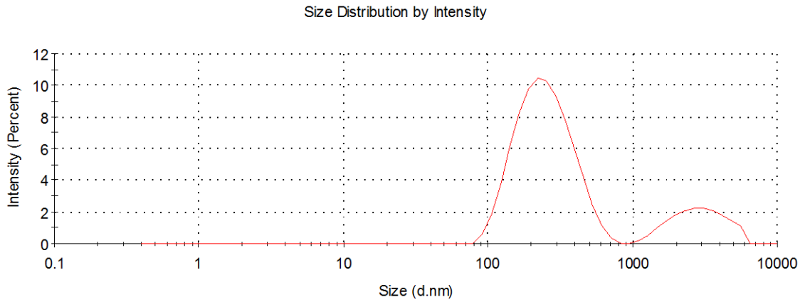
Şekil 6.7. HAP-b tozunun tane boyut dağılımı
