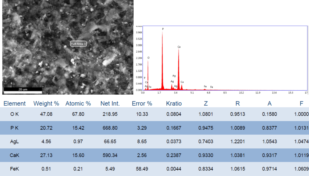
Şekil 6.33. HAP-b ile kumlanmamış Titanyum plaka üzerine 7 mm mesafeden yapılan kaplama sonrası alınan EDX analizi (15000 cm 3 /dak gaz akışıyla) (10 tur)
