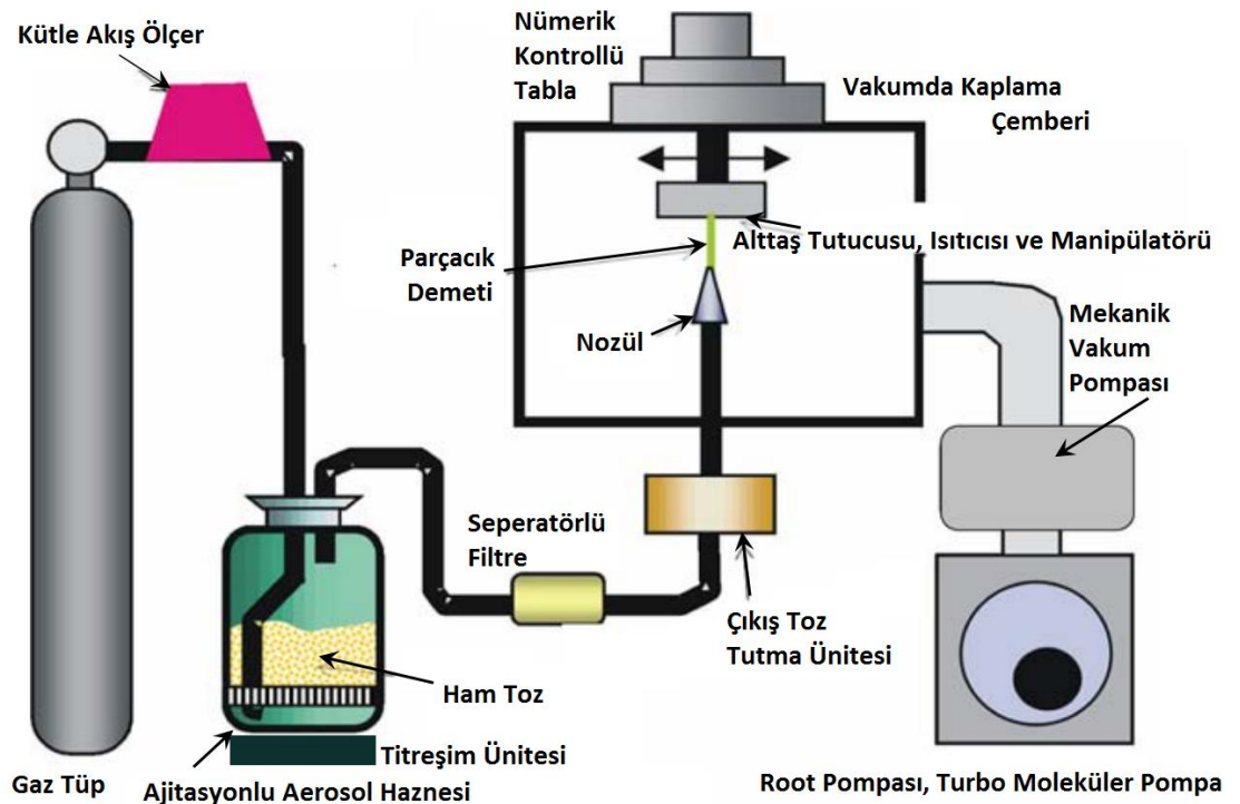
Şekil 3.11. Aerosol Kaplama ünitesinin parçalarıyla birlikte açıklamalı gösterimi [9]
