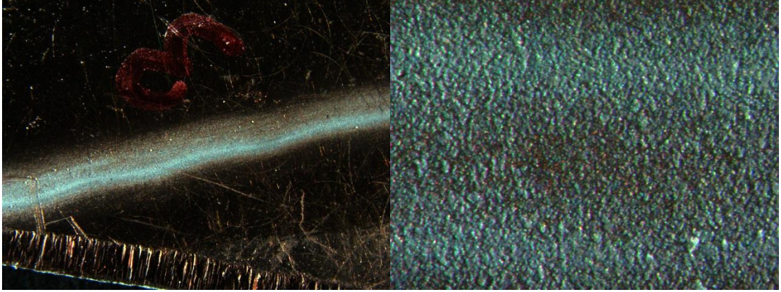
Şekil 5.8. Nozülün 3 tur atmasıyla oluşan yapının 11x ve 30x büyütmedeki optik mikroskop görüntüleri
