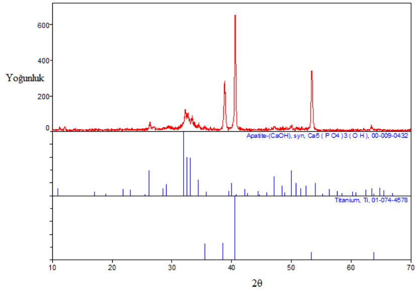
Şekil 6.22. 15000 cm 3 /dak gaz akış hızıyla ve HAP-k ile kaplanmış titanyum numunesinin XRD örgüsü
