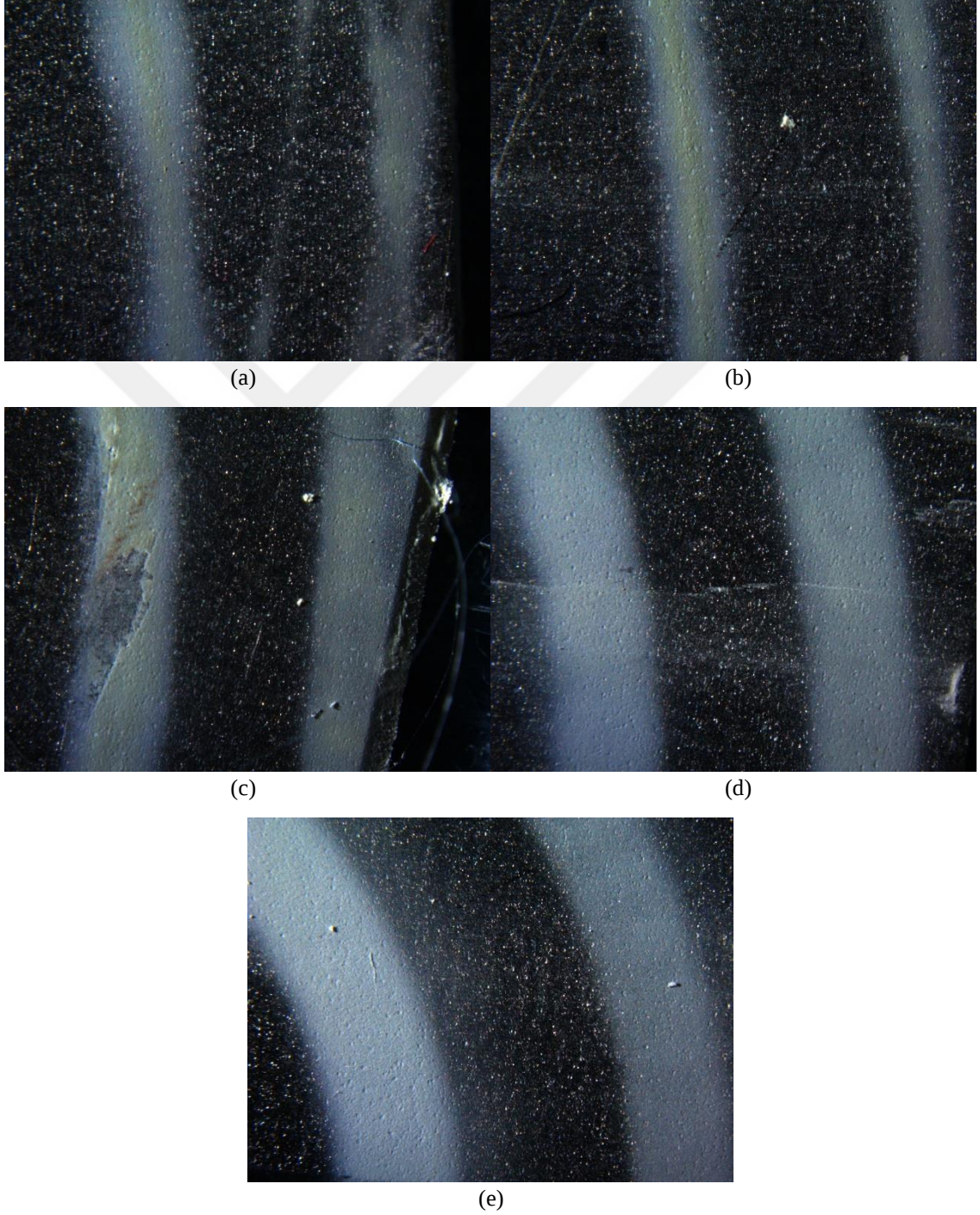
Şekil 6.10. (a) 1000 \text{ cm}^3/\text{dak} , (b) 2000 \text{ cm}^3/\text{dak} , (c) 5000 \text{ cm}^3/\text{dak} , (d) 10000 \text{ cm}^3/\text{dak} , (e) 15000 \text{ cm}^3/\text{dak} gaz akış hızı ile kaplanmış numunelerin 11x büyütmede optik mikroskop görüntüleri
