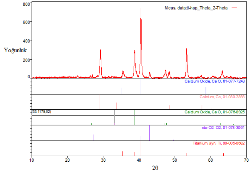
Şekil 6.21. 15000 cm 3 /dak gaz akış hızıyla ve HAP-s ile kaplanmış çelik numunesinin XRD örgüsü
