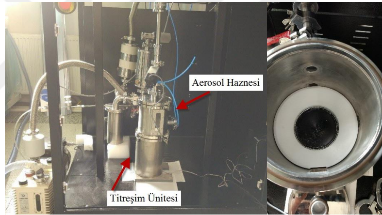
Şekil 5.12. Aerosol haznesi
