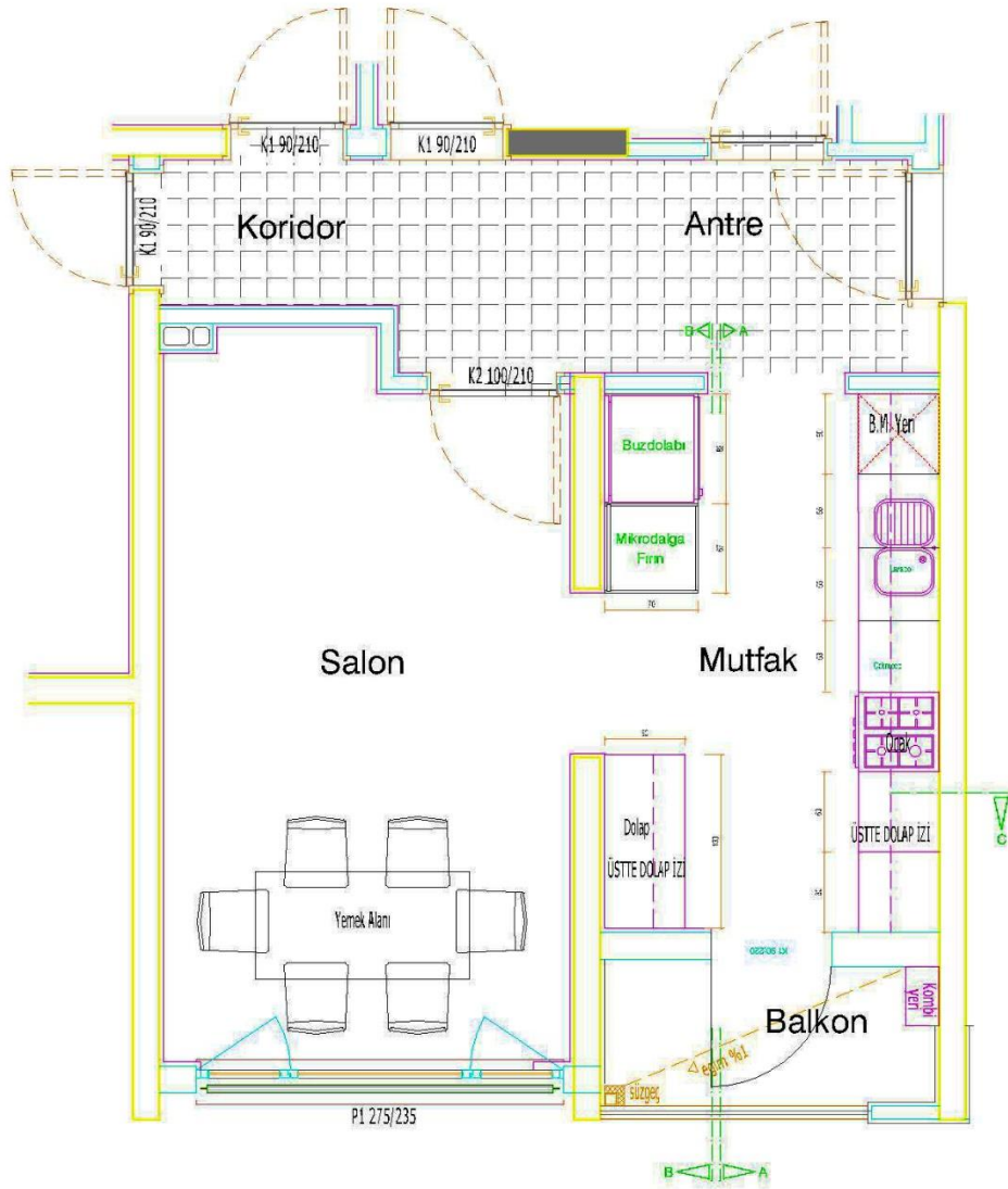
Şekil 4.29. İkinci alternatif TOKİ 2+1 konut mutfak 1/50 yerleşim planı
