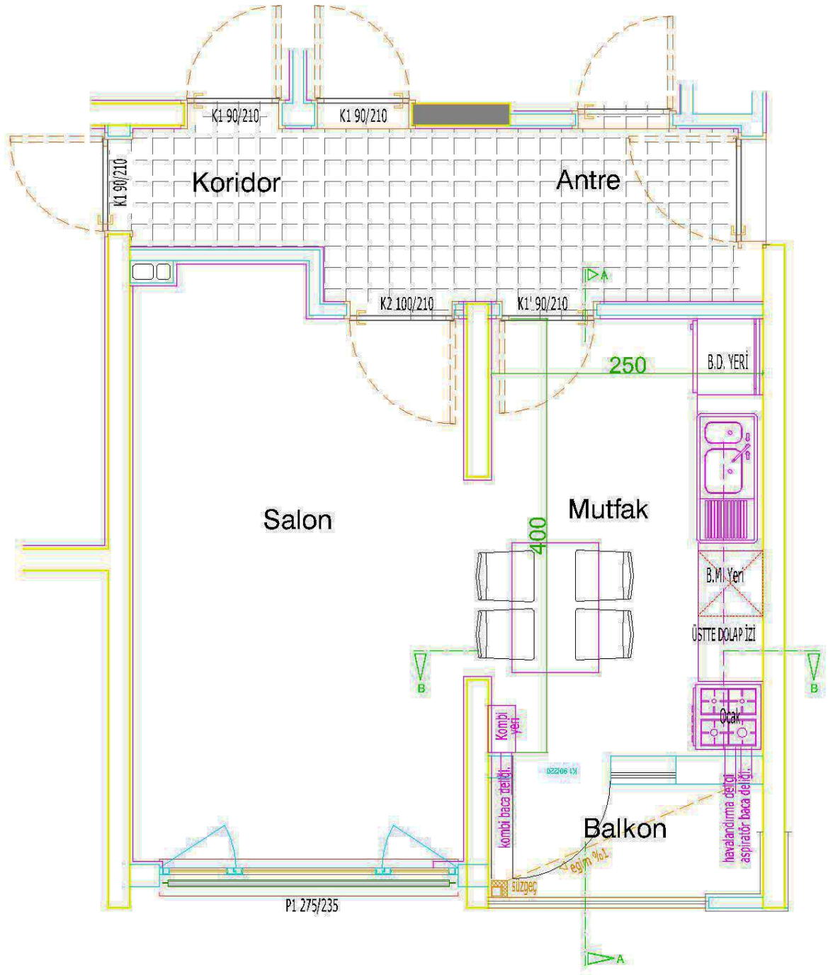
Şekil 3.6. TOKİ 2+1 mutfak yerleşim planı
