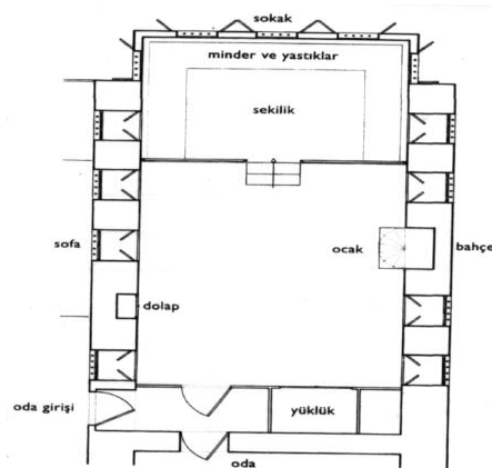
Şekil 2.10. Çelikbaşlar (Baki Bey) Konağı başoda planı (Reha,1999).
