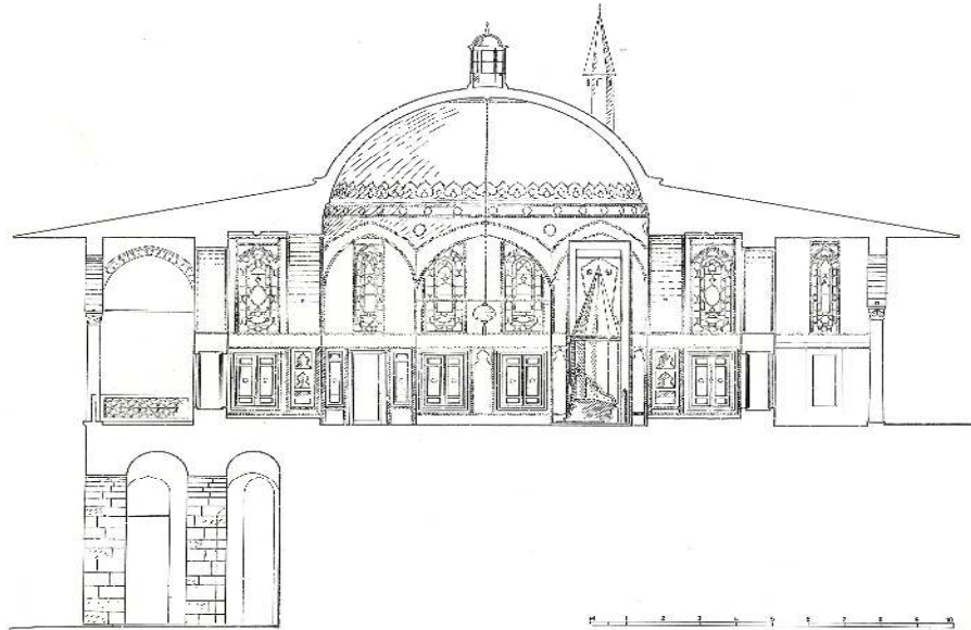
Şekil 4.3. Bağdat Köşkün Şematik Kesit (Eldem,1969).
