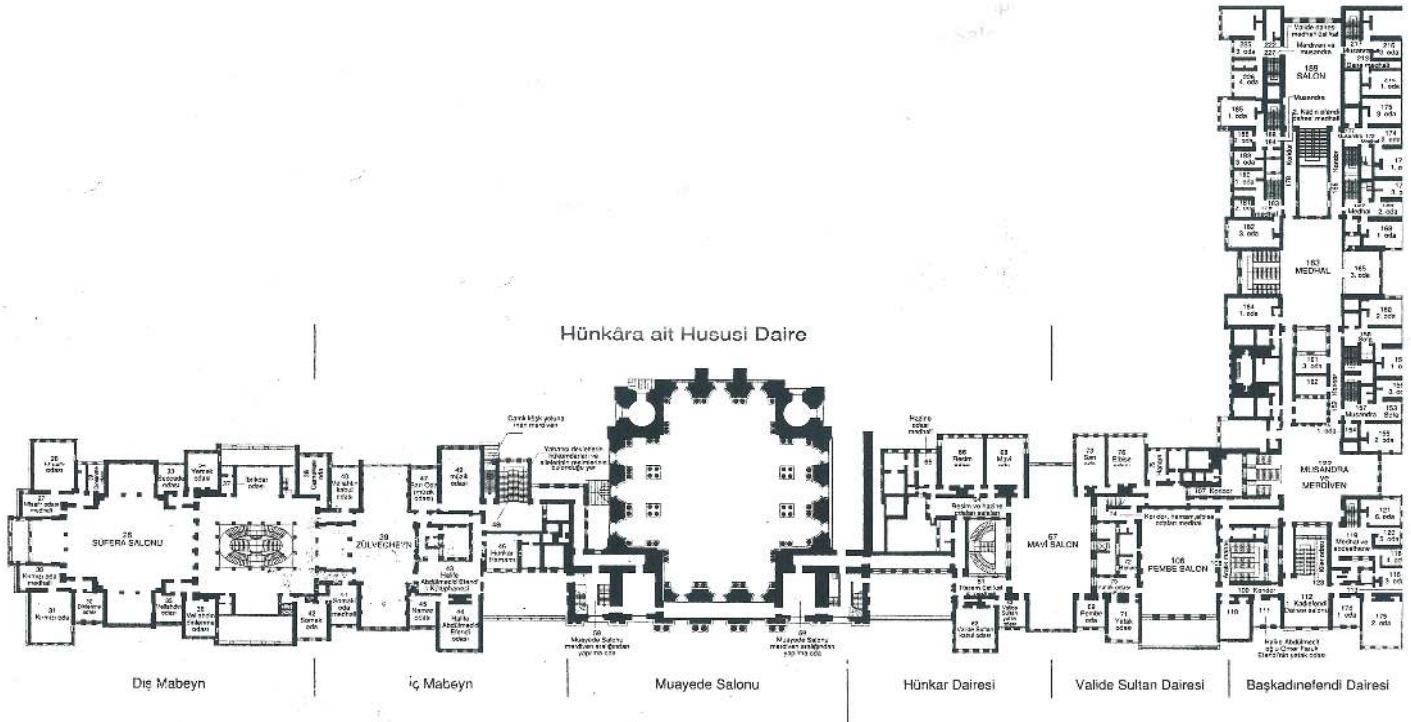
Şekil 4.11.Dolmabahçe Sarayın Planı (Esemenli,2002).
