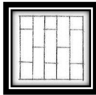
Çizim 104: Ardışık Dikey Formda Tuğla Örgüsü Detay Çizimi
