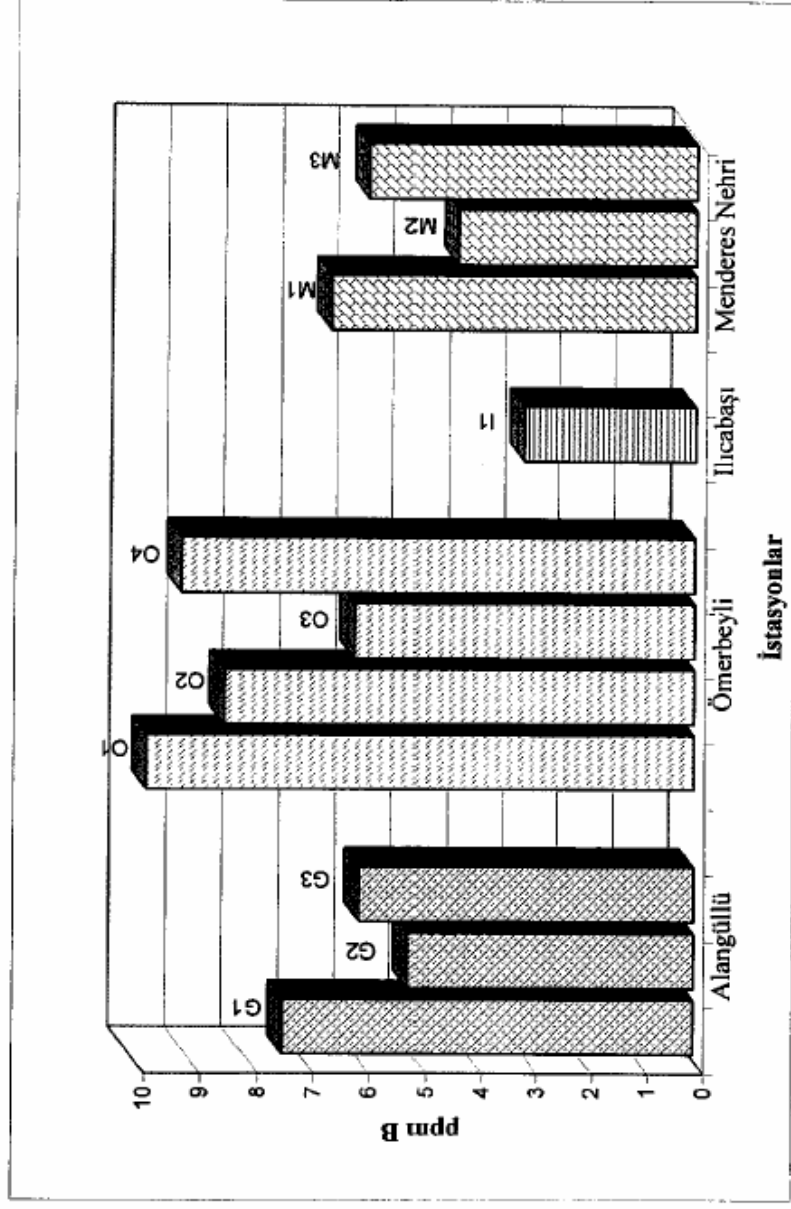
Şekil 3.6 Toprak numunelerinde kalan bor türleri
