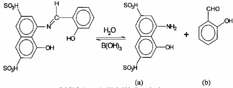
Şekil 1.2 Azometin-H'nin hidroliz mekanizması
