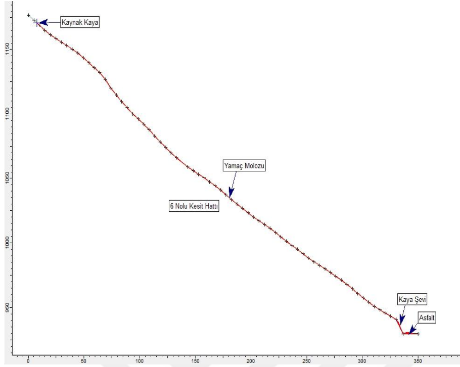
Ek Şekil 2.13. Kızılkaya Dasiti KH-6 nolu hat için kaya düşme analizi
