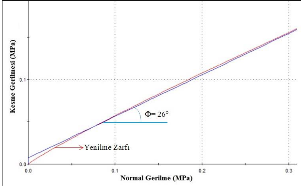
Şekil 3.21. Dasitlerin süreksizliklerine ait kesme gerilmesi- normal gerilme grafiği
