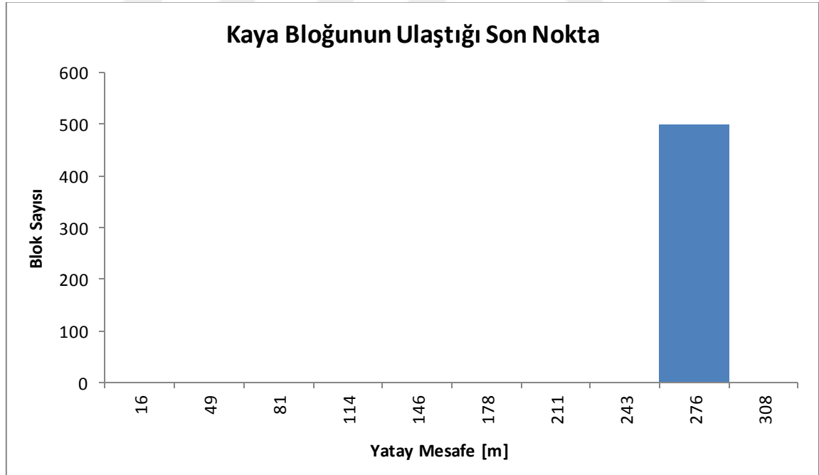
Ek Şekil 4.6.2. Sariosman Monzograniti SH-6 hattında bariyer uygulaması sonrası blokların ulaştığı son nokta
