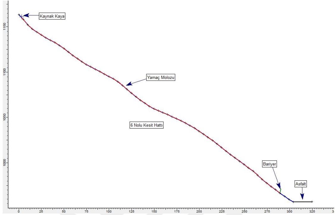
Ek Şekil 4.6.1. Sariosman Monzograniti SH-6 hattında bariyer uygulaması sonrası kaya düşme analizi
