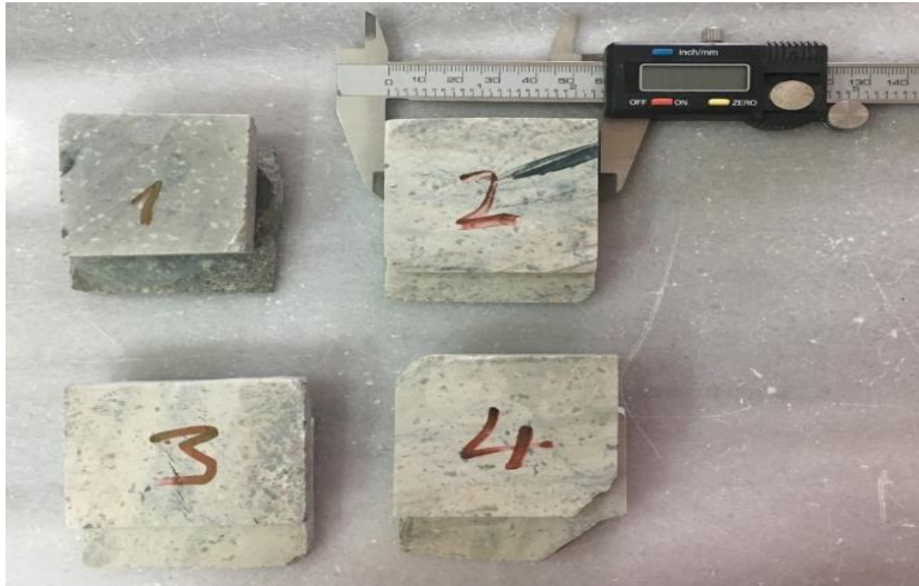
Şekil 3.17. Dasitlere ait makaslama deneyi örnekleri
