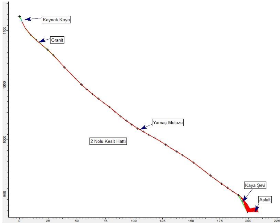
Ek Şekil 2.2. Sariosman Monzograniti SH-2 nolu hat için kaya düşme analizi
