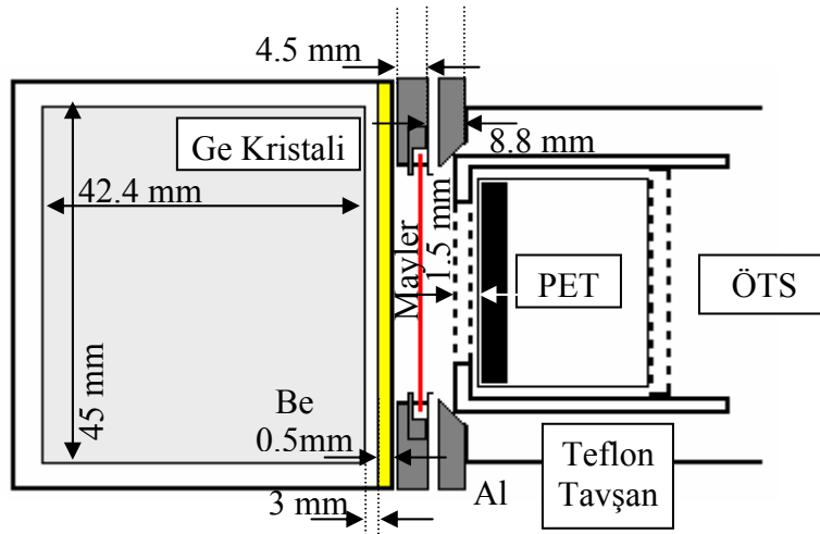
Şekil 4.1 Sayım geometrisi
