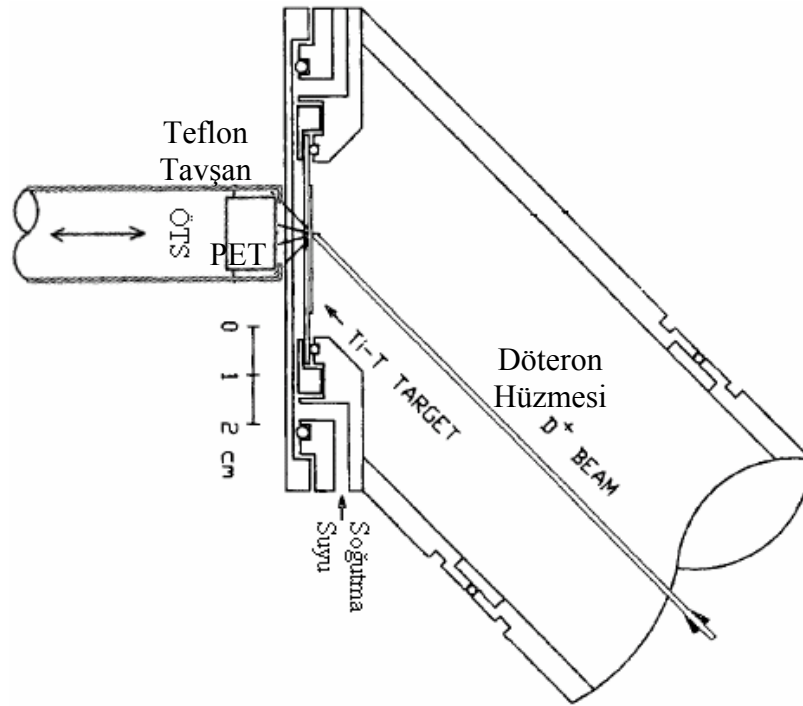
Şekil 4.5 Işınlama geometrisi
