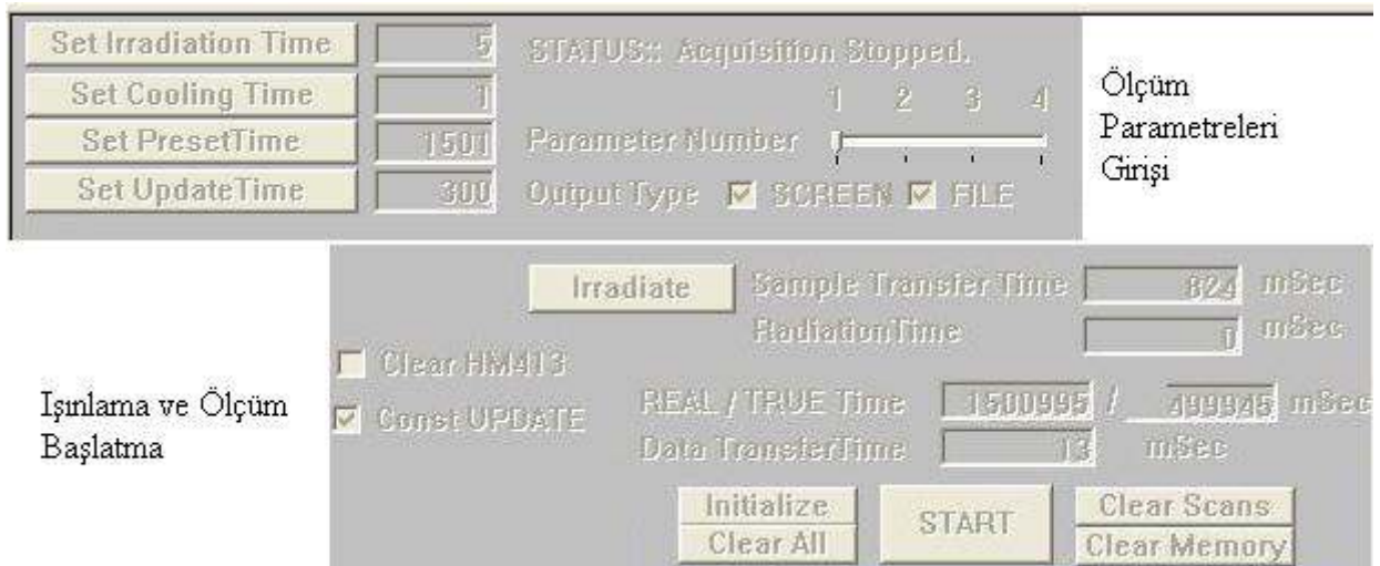
Şekil 3.5 MCA yazılımı komut bölümü
