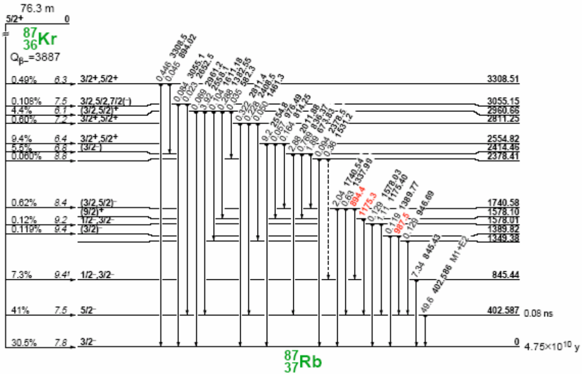
Şekil 5.1 ^{87}\text{Kr} \rightarrow ^{87}\text{Rb} t_{1/2}=76.3 m 5 \beta^- bozunumundan gelen \gamma geçişleri
