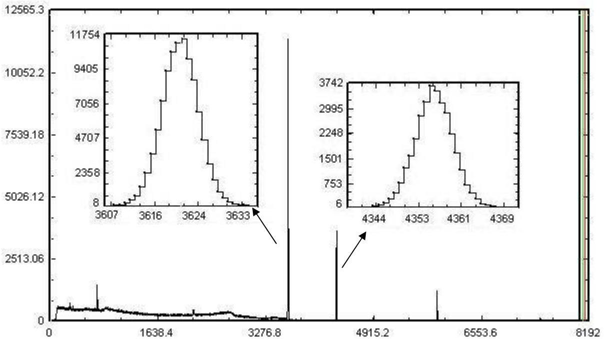
Şekil 4.7 \text{Al}(n,p)\text{Mg} reaksiyonu MCA spektrumu
