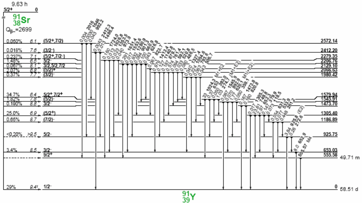
Şekil 5.5 ^{91}\text{Sr} \rightarrow ^{91}\text{Y} t_{1/2}=9.63 h \beta^- bozunumundan gelen \gamma geçişleri
